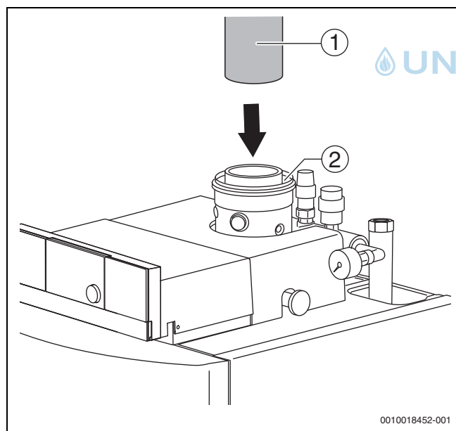
Bild 15 Montage Abgasrohr
