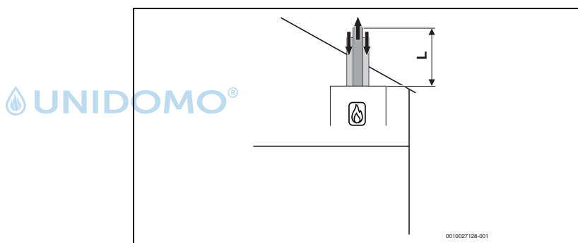
Bild 9 Vertikale konzentrische Luft-Abgas-Führung nach C 33x
