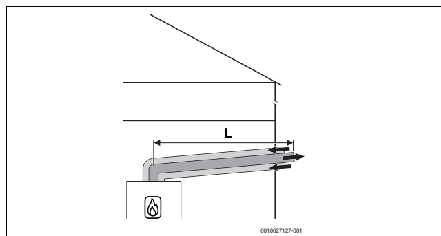
Bild 7 Horizontale konzentrische Luft-Abgas-Führung nach C 13x durch die Außenwand
