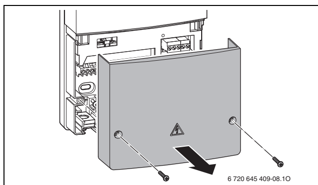
Bild 27 Gehäuse öffnen
