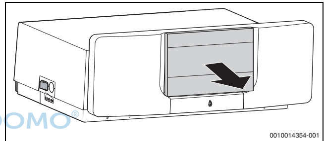
Bild 32 Abdeckung abziehen
