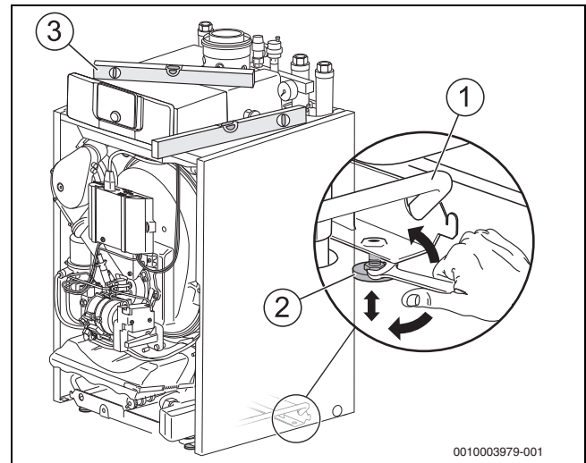
Bild 15 Heizkessel ausrichten
