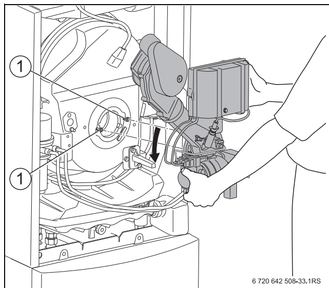
Bild 81 Brenner herausnehmen
