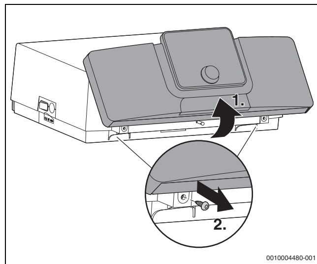
Bild 24 Bedieneinheit nach oben geklappt
