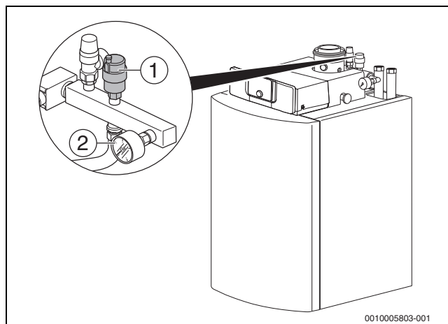
Bild 19 Heizungsanlage befüllen
