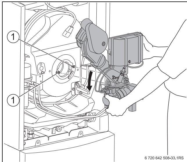
Bild 61 Brenner herausnehmen
