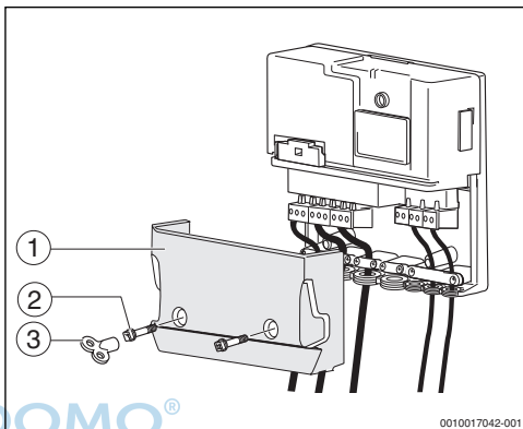
Afb. 77 Monteren klemmenafdekking
