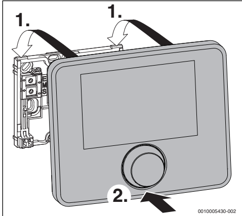
Bild 4 Bedieneinheit einhängen
