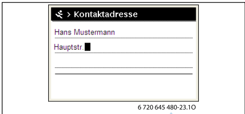
Bild 10 Kontaktadresse eingeben
