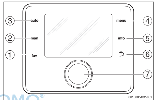
Bild 6 Bedienelemente
