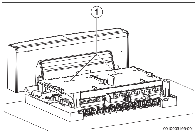
Bild 8 Ansicht ohne Abdeckhaube und ohne Module
