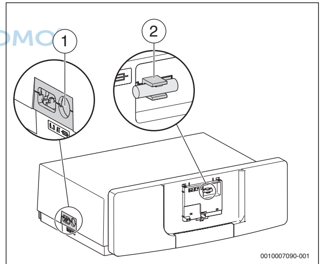
Bild 36 Sicherung ersetzen
