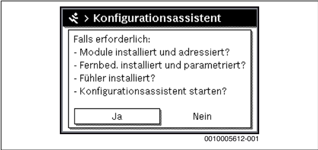
Bild 20 Konfigurationsassistent starten
