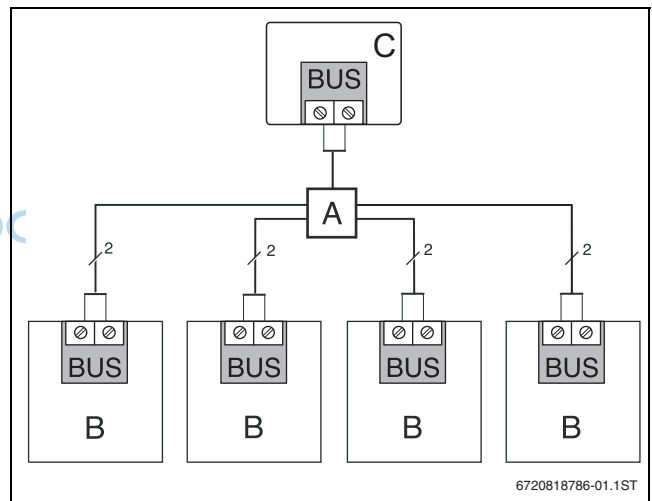
Bild 47 BUS-Leitungen anschließen
