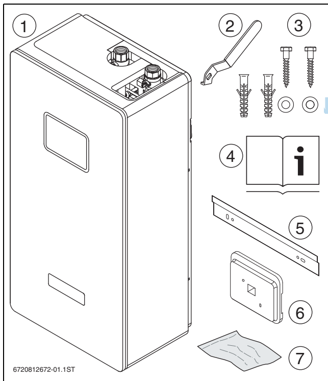
Bild 2 Lieferumfang Einzelstation
