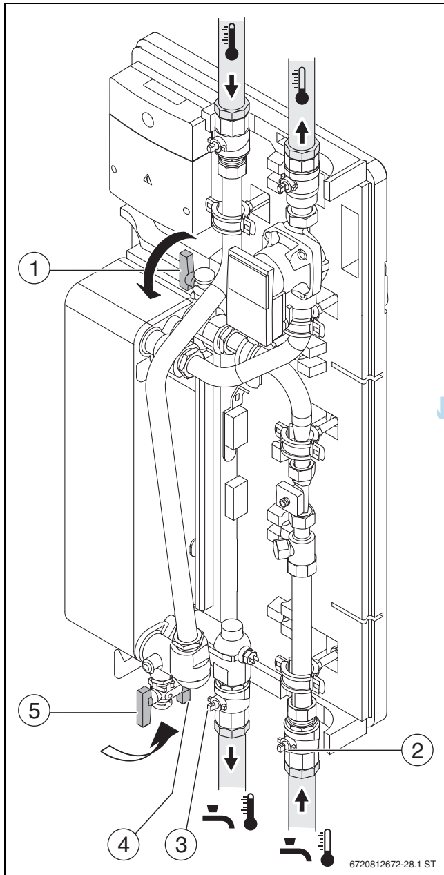
Bild 49 Spül-/Befüllanlagen an der Einzelstation
