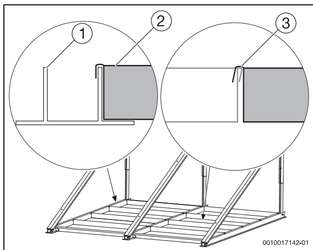
Bild 26 Kollektorstützen mit Beschwerungswannen für 2 Kollektoren
