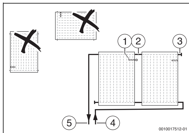
Bild 10 Kollektoren anordnen
