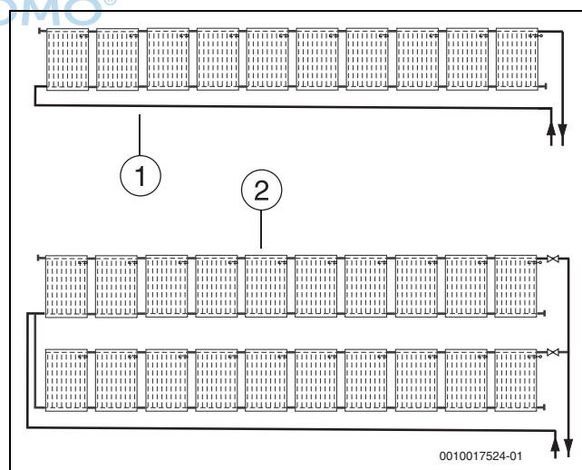
Bild 11 Hydraulischer Anschluss
