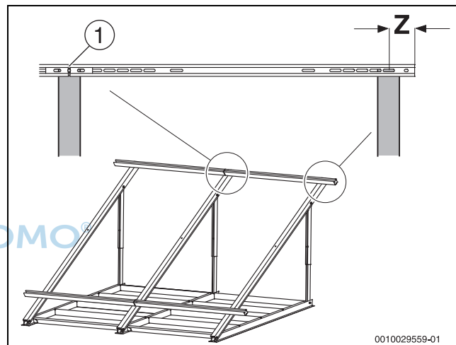
Bild 29 Profilschienen positionieren
