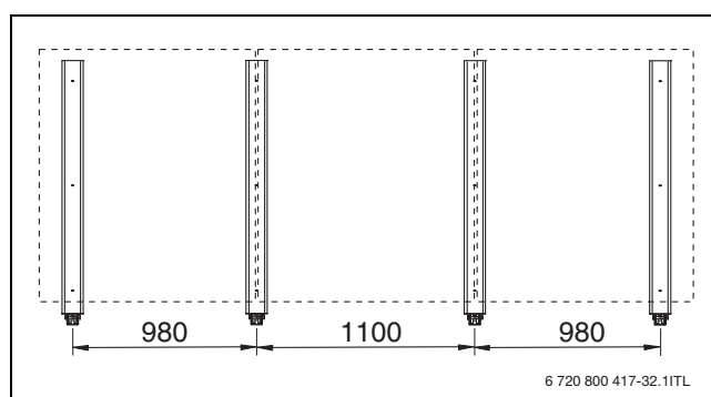
Bild 20 3 Kollektoren (Maße in mm)
