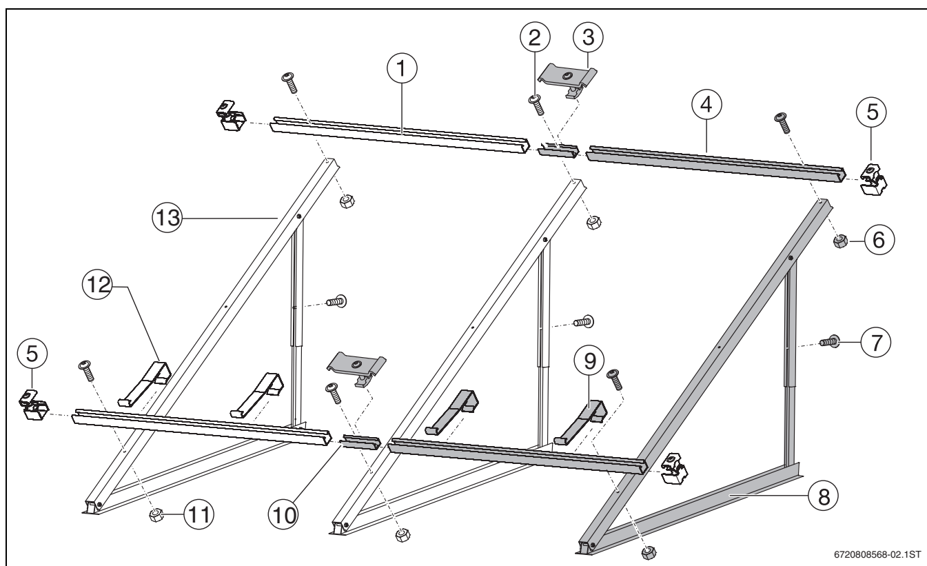
Bild 3 Montage-Set für 2 Kollektoren: 1 Montage-Set Grundaufführung, 1 Montage-Set Erweiterung (grau)
