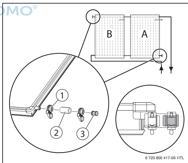
Bild 36 Stopfen montieren
