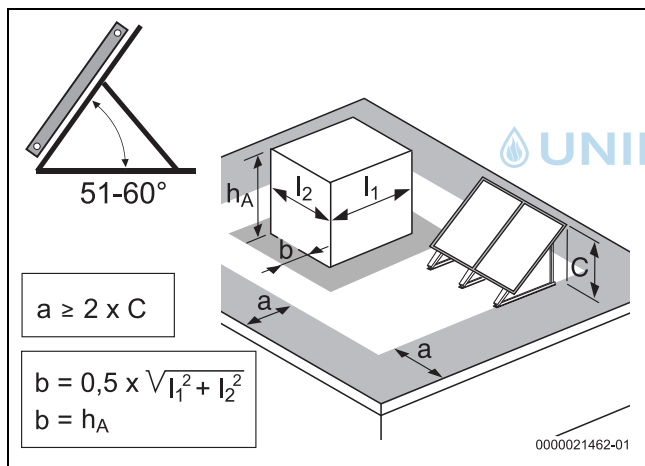
Bild 16 Bei Maß a ist der größere Wert maßgebend; bei [b] ist der kleinere Wert maßgebend (Anstellwinkel Kollektoren 51°-60°)
