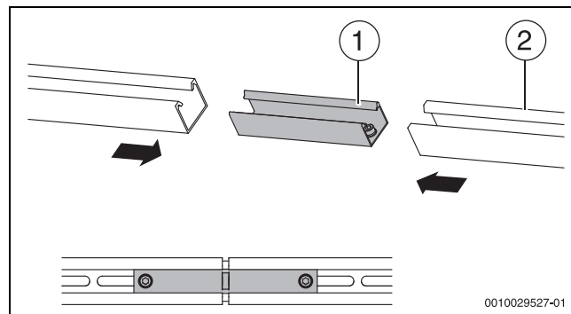
Bild 28 Profilschienen verbinden
