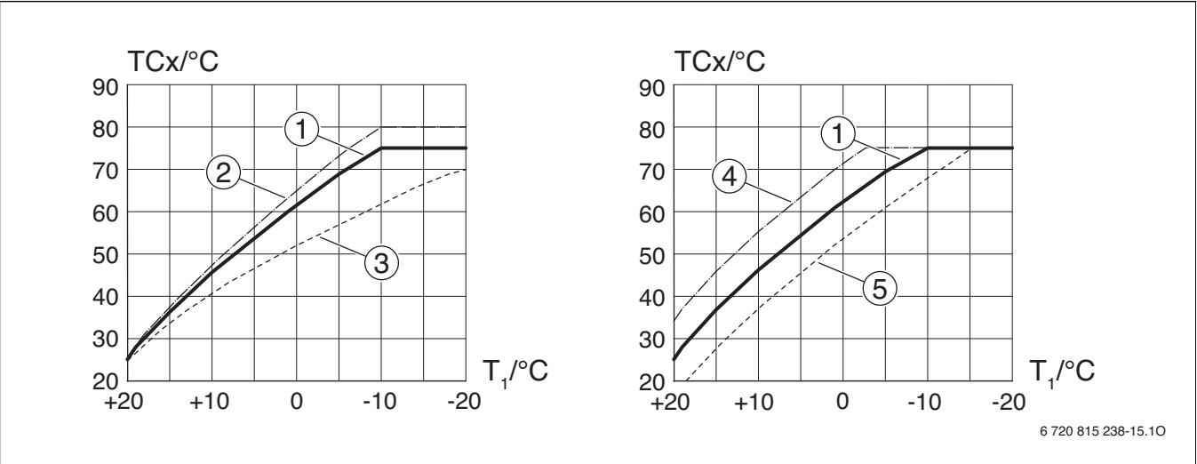
Bild 9 Einstellung der Heizkurve für Heizkörper / Konvektoren Links: Steigung über Auslegungstemperatur T_{AL} und minimale Außentemperatur T_{1,min} Rechts: Parallelverschiebung über Raumtemperatur-Offset oder über gewünschte Raumtemperatur
