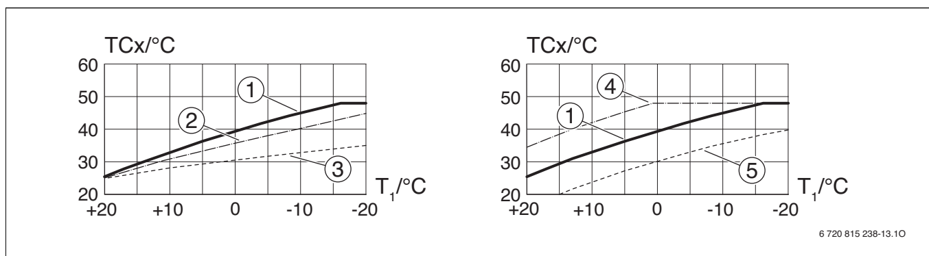
Bild 8 Einstellung der Heizkurve für Fußbodenheizung
