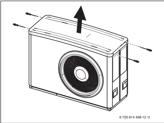
Bild 34 Abdeckung entfernen
