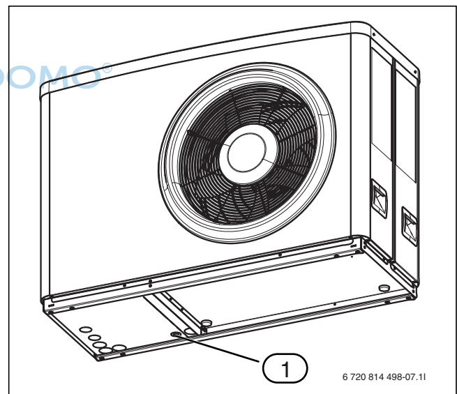
Bild 14 Kondensatablauf
