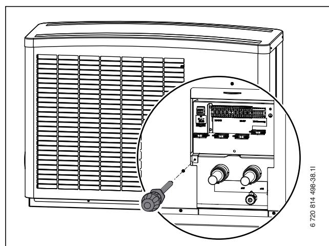
Bild 18 Anschlussbereich lösen
