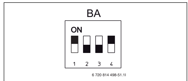
Bild 39 Nur Heizung
