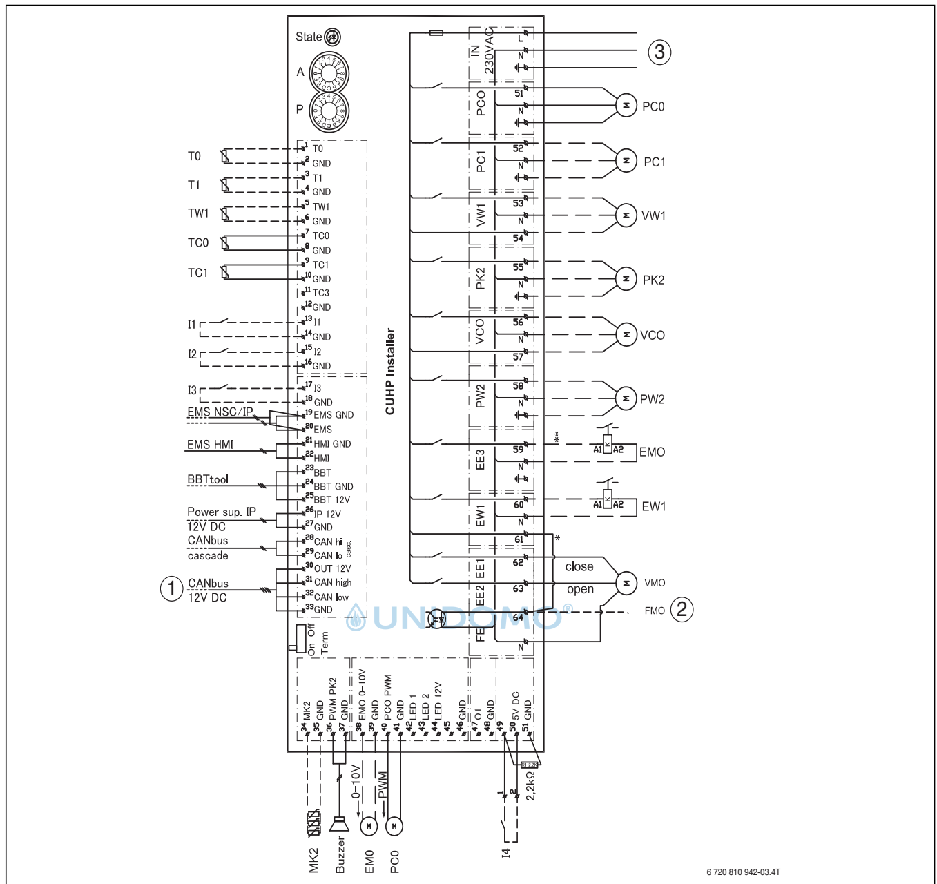
Bild 24 Schaltplan Installationsmodul
