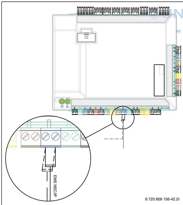
Bild 12 EMS-Anschluss am Installationsmodul
