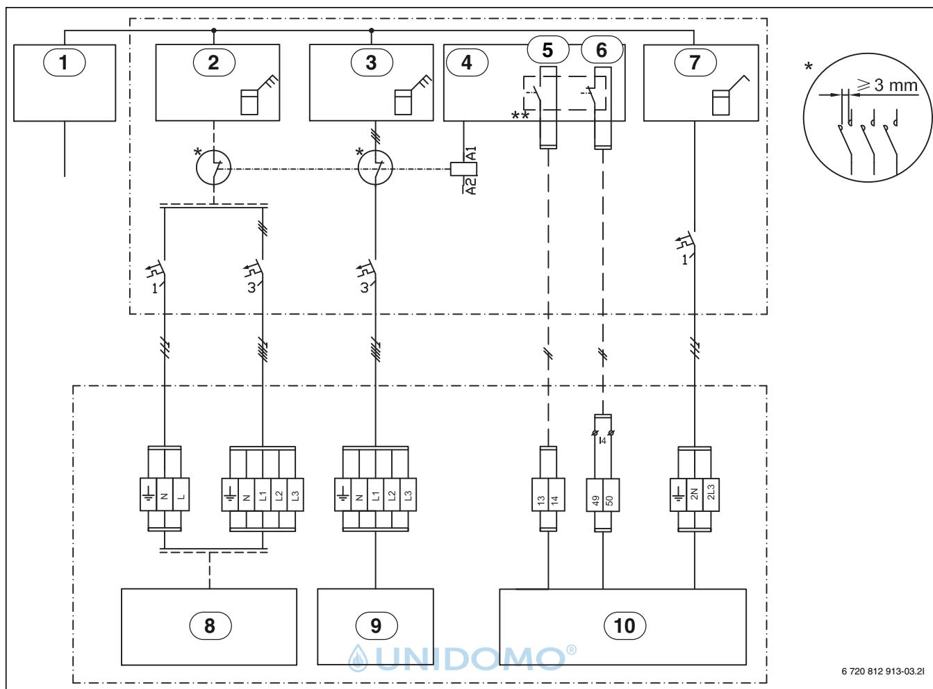
Bild 56 EVU Typ 1
