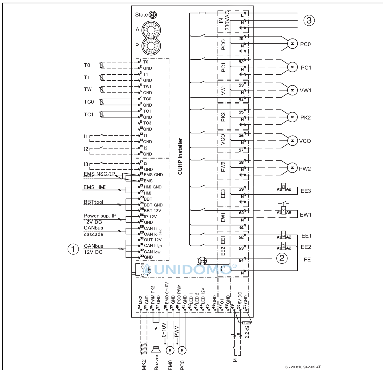
Bild 42 Schaltplan Installationsmodul
