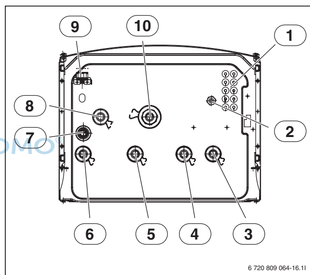
Bild 20 Rohranschlüsse Innenmodul für den bivalenten Betrieb ACB (Ansicht von unten)
