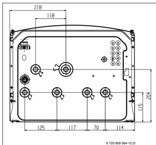
Bild 19 Innenmodul für den bivalenten Betrieb ACB, Abmessungen in mm (Ansicht von unten)
