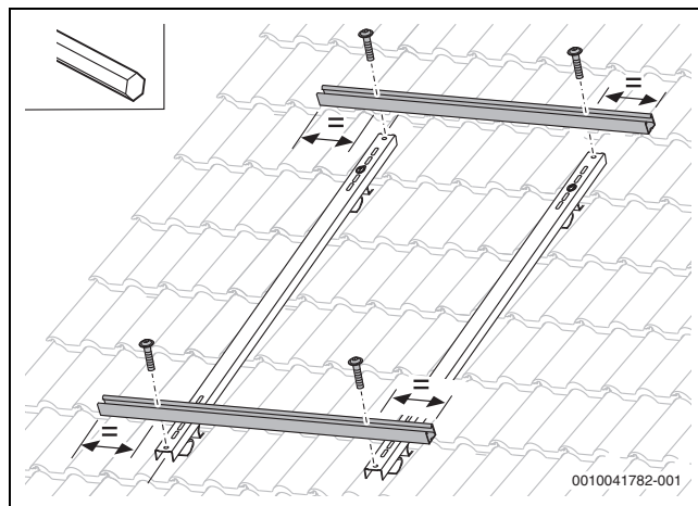
Bild 39 Profilschienen mit Schraube und Nietmutter verbinden
