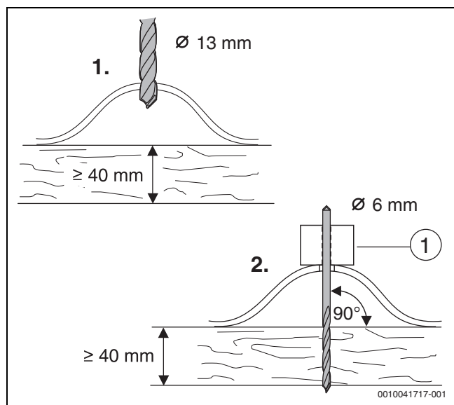
Bild 32 Vorborenen
