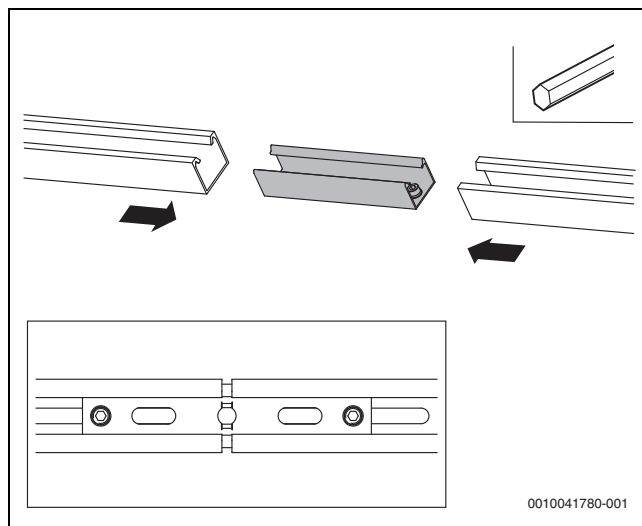
Bild 38 Profilschienen verbinden
