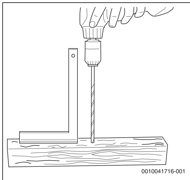
Bild 31 Bohrschablone herstellen
