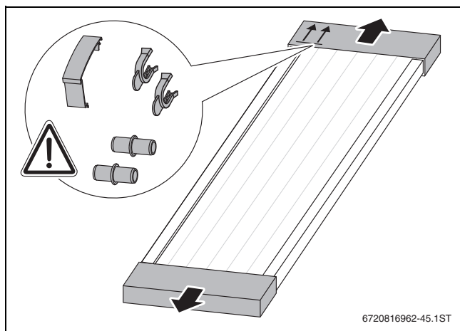
Bild 44 Verpackungsdeckel entfernen
