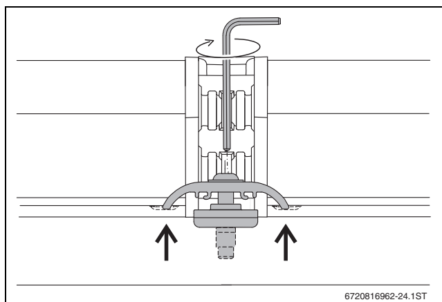
Bild 51 Doppelseitigen Kollektorspanner befestigen
