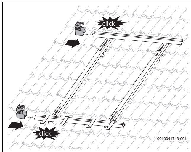
Bild 43 Kollektorspanner montieren
