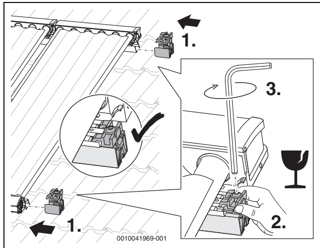
Bild 52 Kollektorspanner montieren
