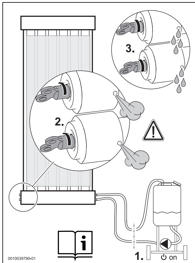
Bild 57 Entlüften
