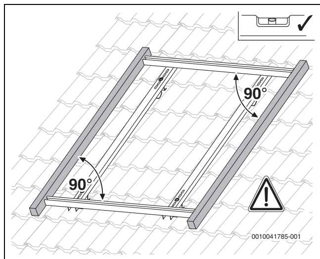
Bild 40 Profilschienen ausrichten
