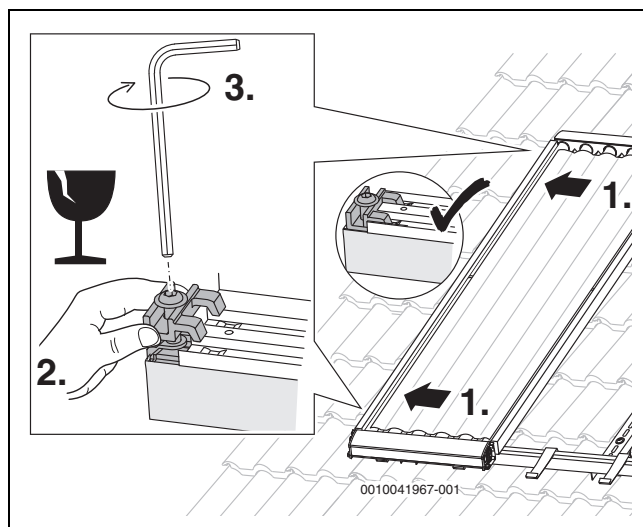
Bild 46 Ersten Kollektor befestigen
