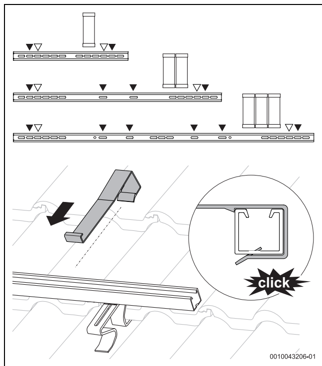
Bild 41 Abrutschsicherung montieren
