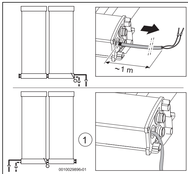
Bild 53 Kollektortemperaturfühler vorsichtig herausziehen
