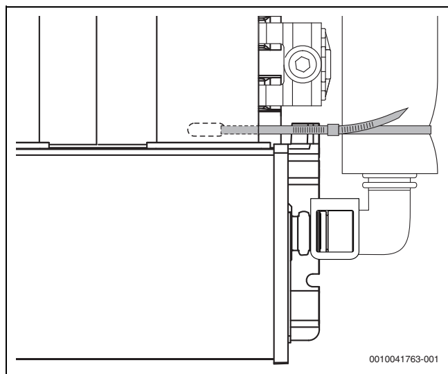
Bild 55 Beide Anschlussrohre mit Kabelbinder sichern
