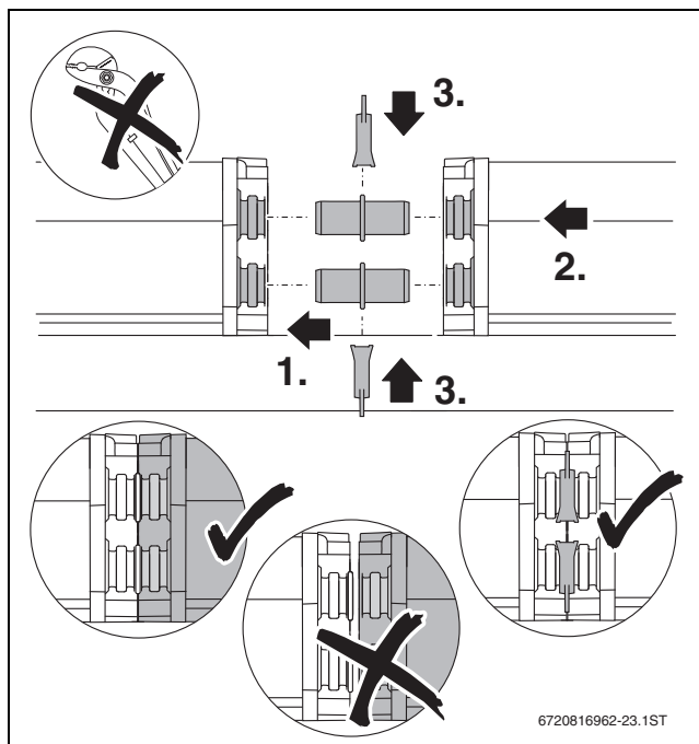
Bild 50 Ersten und zweiten Kollektor miteinander verbinden
