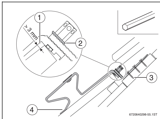
Bild 26 Sparrenanker befestigen
