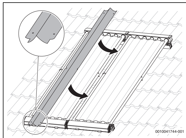
Bild 58 Zwischenspiegel einlegen
