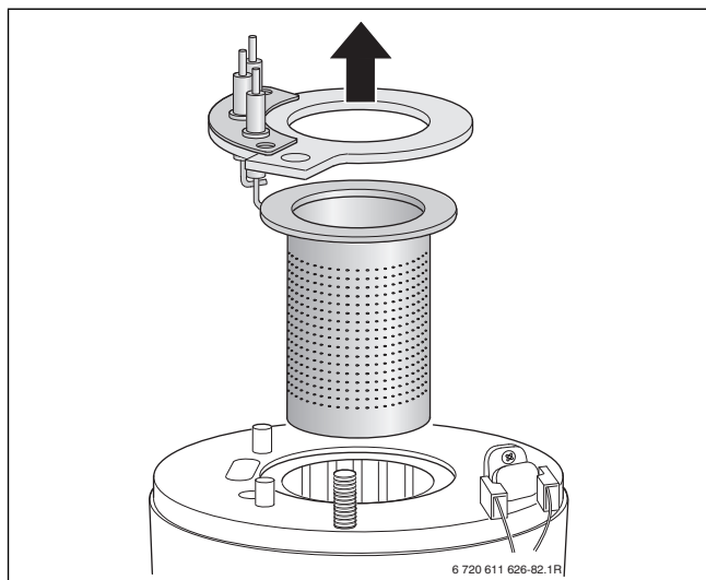
Bild 88 Brenner herausnehmen
