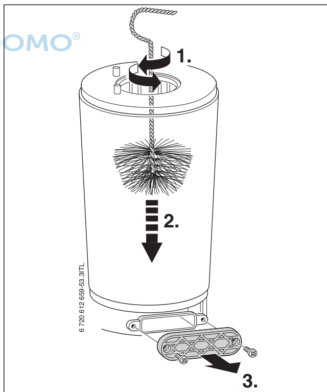
Bild 91 Wärmeblock reinigen
