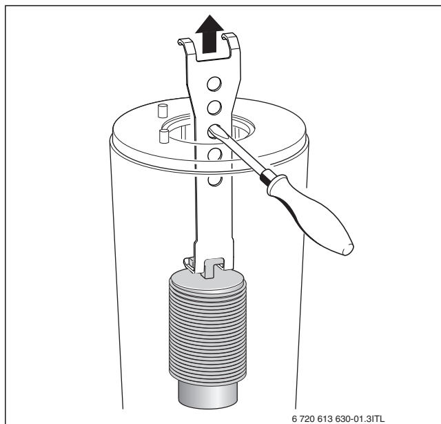
Bild 90 Unteren Verdrängungskörper herausnehmen
