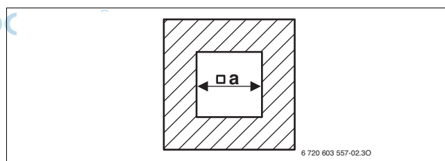
Bild 9 Quadratischer Querschnitt für raumluftabhängig
