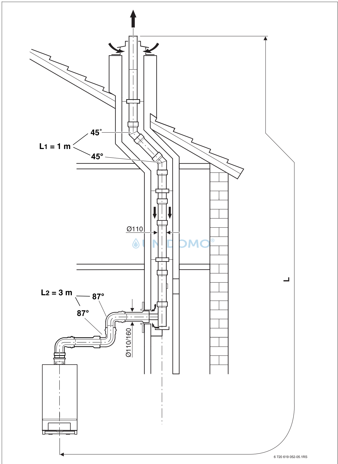
Bild 13 Beispiel Abgasrohlängen
