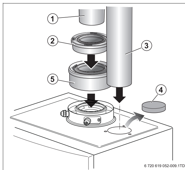
Bild 7 Getrenntrohranschluss
