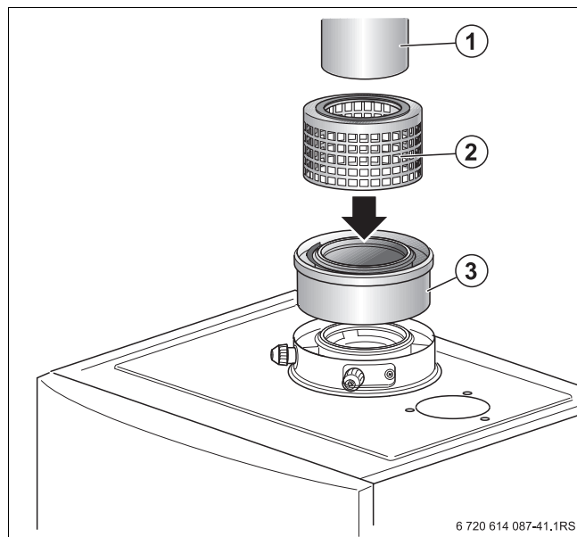
Bild 8 Einzelrohranschluss (raumluftabhängig)
