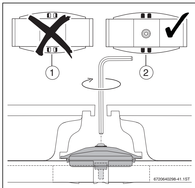
Bild 48 Kollektorspanner montiert
