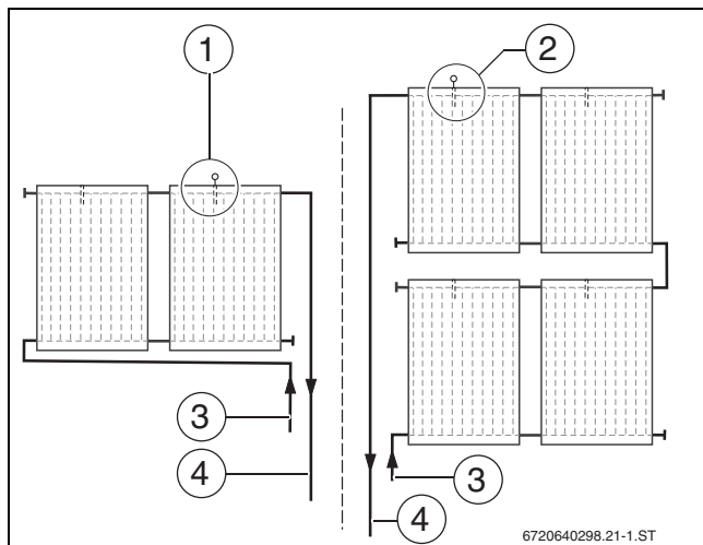
Bild 51 Position des Kolleortemperaturfühlers
