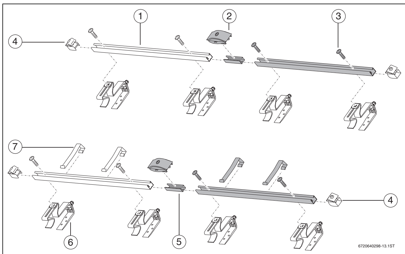
Bild 5 Montage-Set für 2 Kollektoren: 1 Montage-Set Grundaufbau, 1 Montage-Set Erweiterung (grau) und 2 Montage-Sets für Dachziegel
