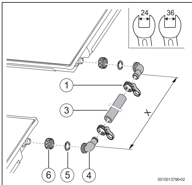
Bild 63 Verbindungs-Set montieren
