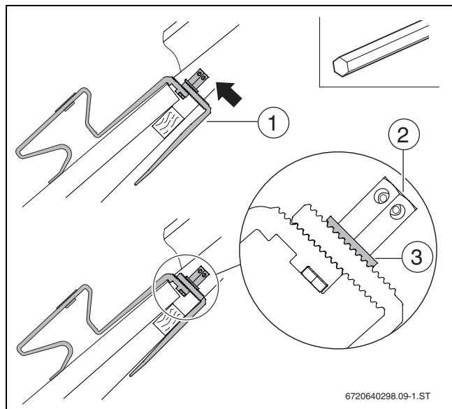
Bild 19 Dachhaken-Unterteil hochschieben
