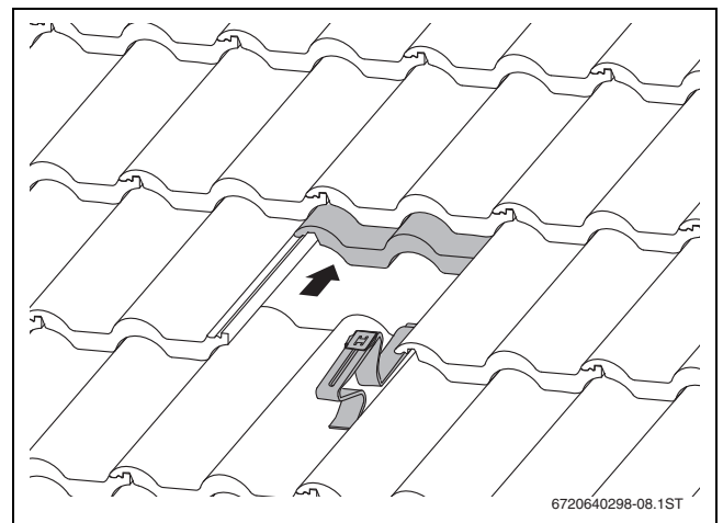
Bild 18 Eingehängter Dachhaken
