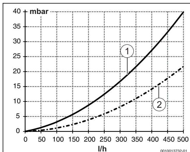
Bild 3 Druckverlustkurve (Wasser-Glykol-Gemisch)
