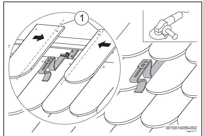
Bild 25 Biberschwanzziegel anpassen
