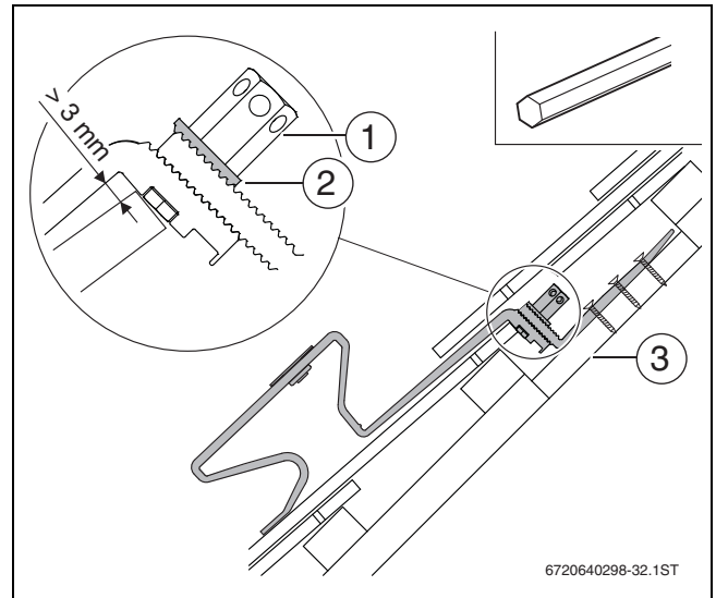
Bild 24 Sparrenanker montieren
