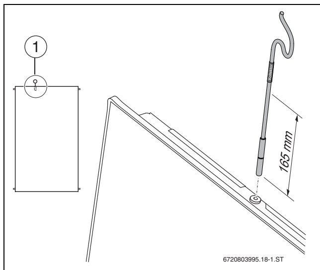
Bild 52 Kolleortemperaturfühler montieren
