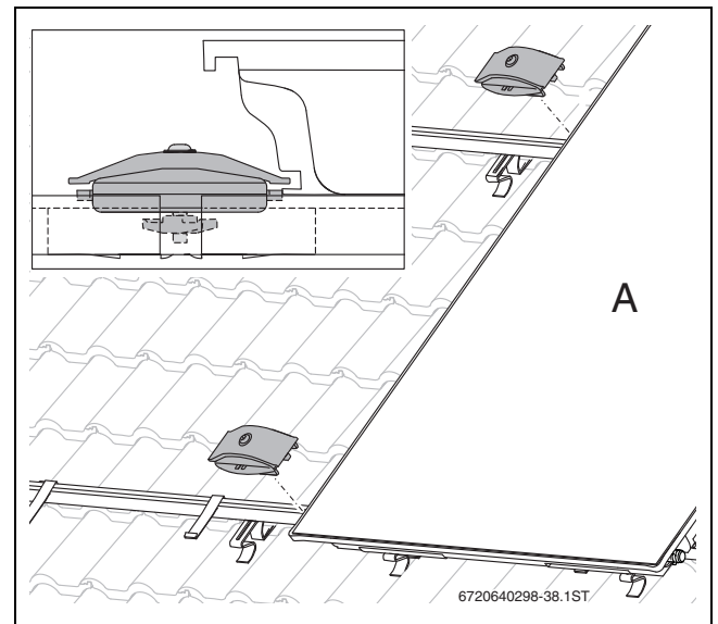
Bild 46 Doppelseitigen Kollektorspanner einlegen
