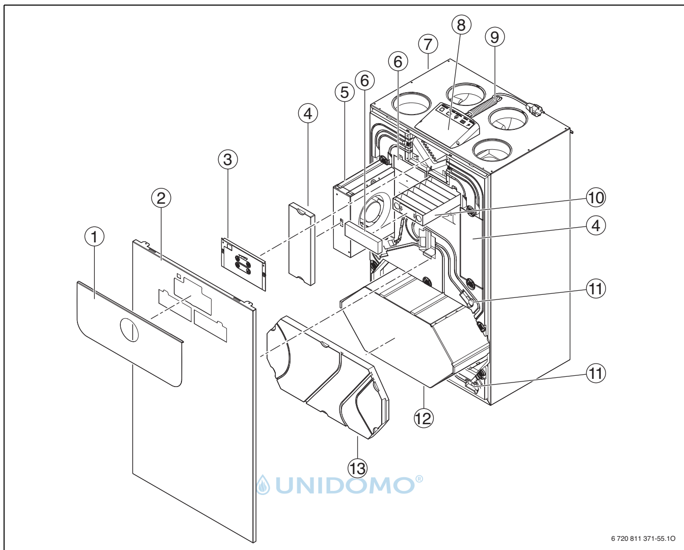
Bild 5 Wohnungslüftungsgerät Vent 5000 C HR 140 W(S)
