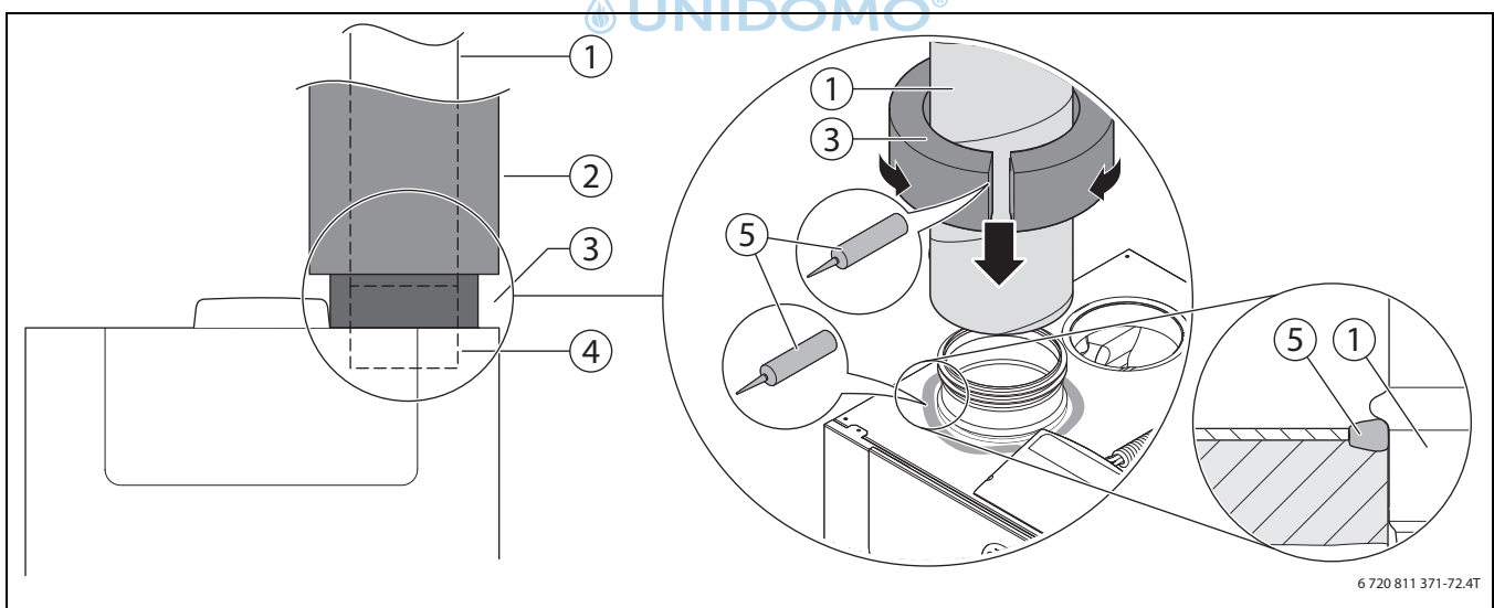
Bild 32 Aufbau Luftrohranschluss mit Wickelfalzrohr
