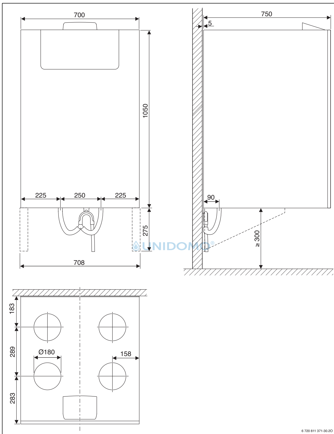
Bild 4 Vent 5000 C HR 350 W(S)
