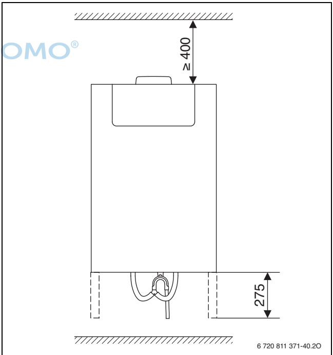
Bild 22 HR 230 W(S), HR 350 W(S)
