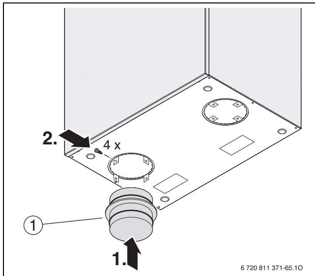
Bild 28 Montage Steckverbinder – Variante A
