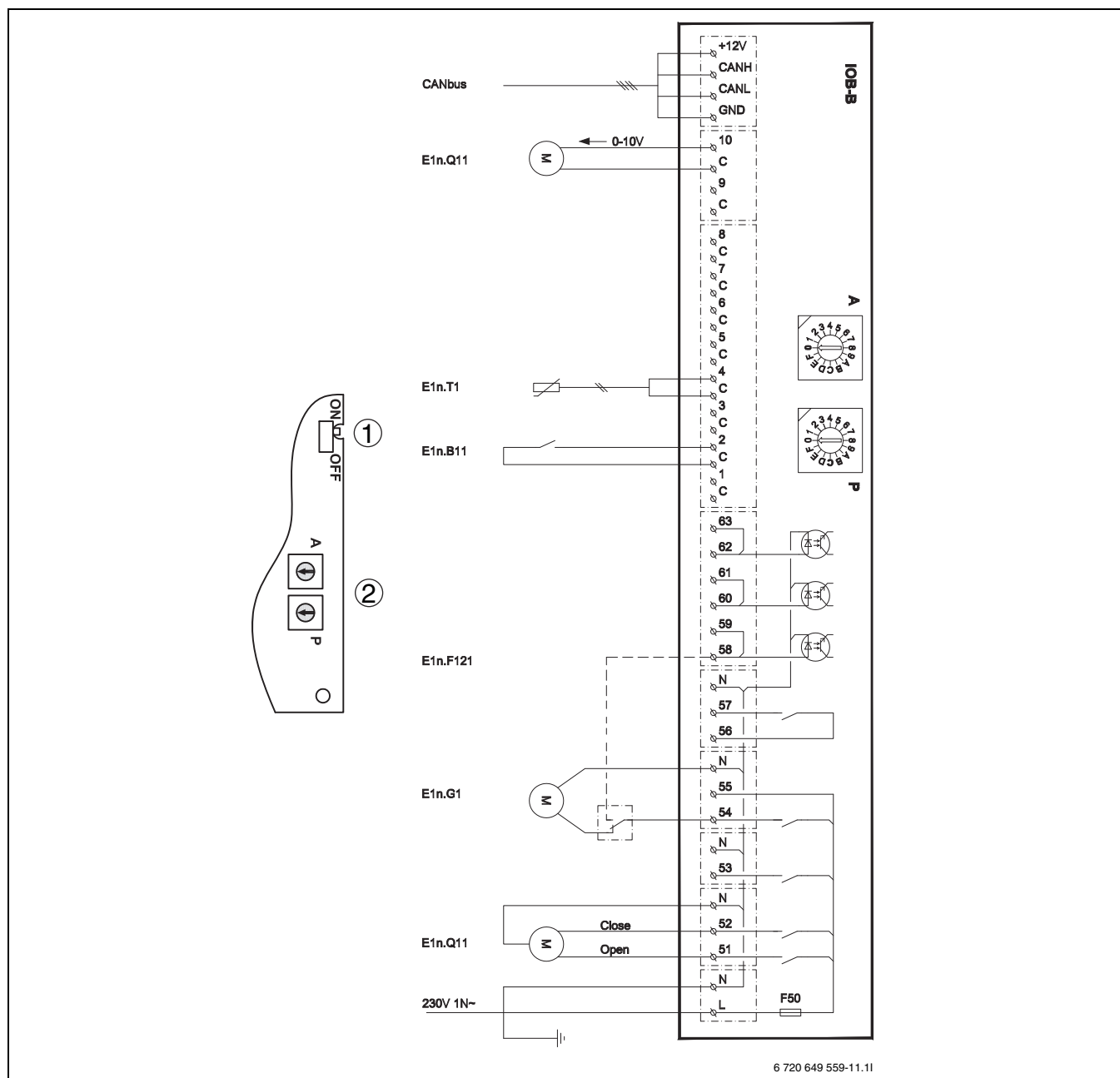
Bild 11 Schaltplan Kreis 3-4
