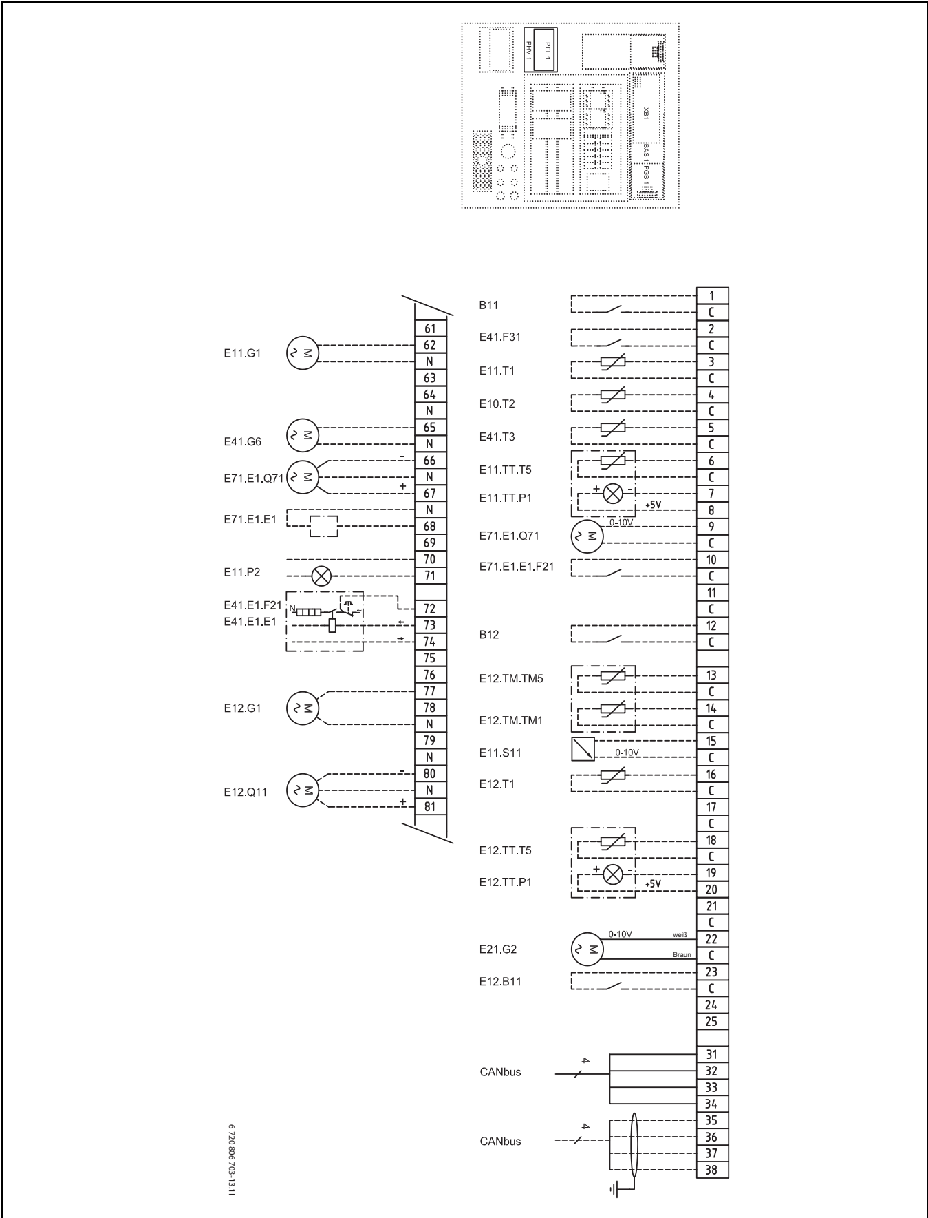
Bild 38 Externe Anschlüsse E21
