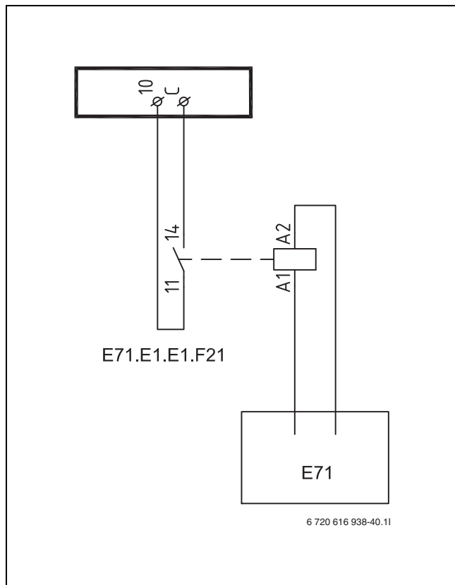
Bild 42 Alarm Zuheizung
