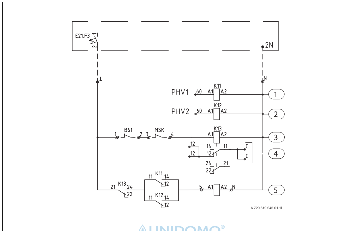
Bild 24 Übersicht Anschluss Elektroschaltschrank - Wärmepumpe
