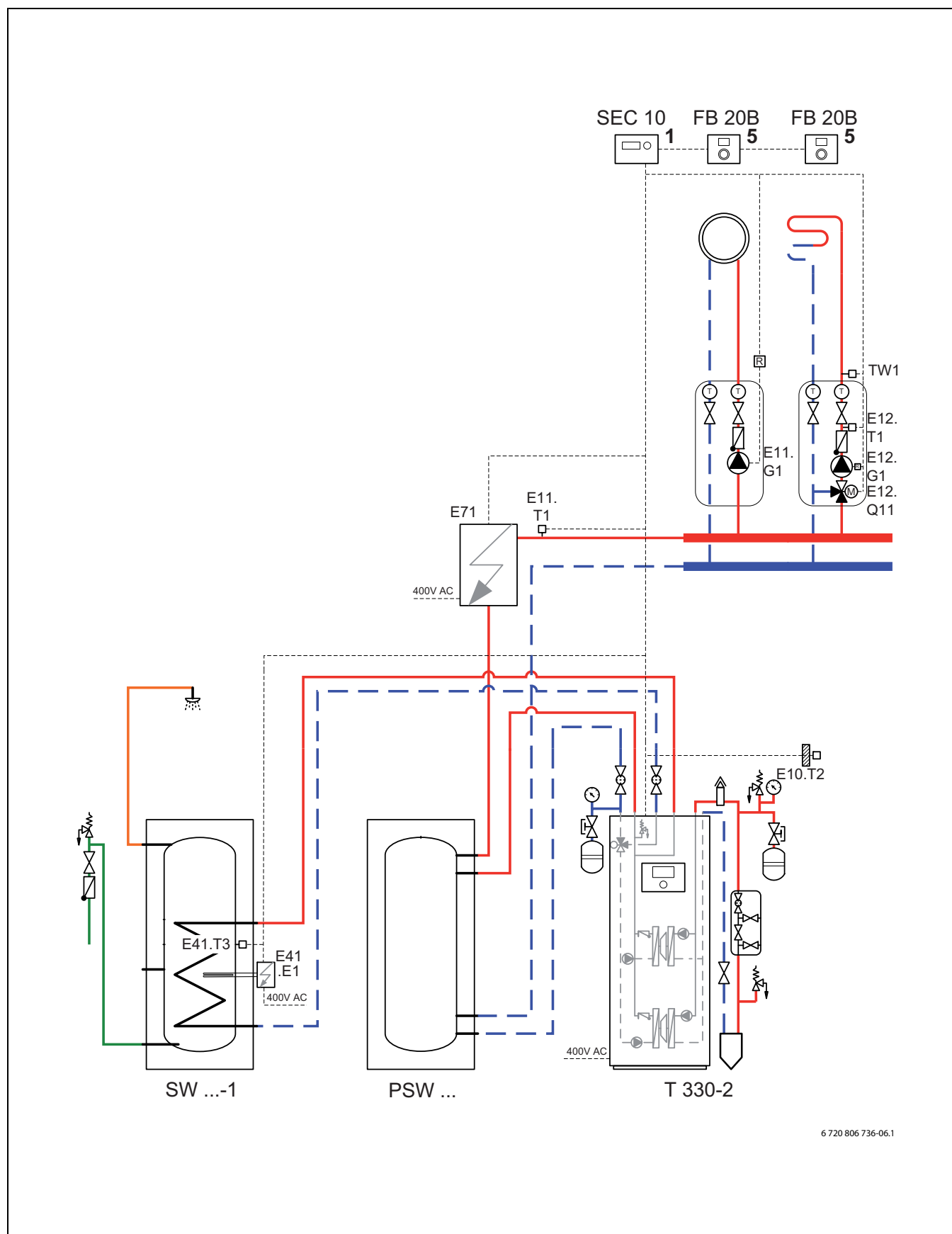
Bild 12 Heizkreis, elektrischer Zuheizer und Pufferspeicher (→ Kapitel 9.2.1, 9.3)
