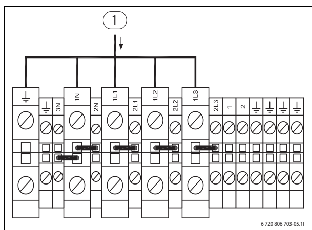
Bild 30 Standardausführung
