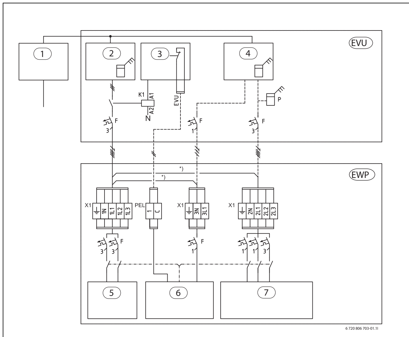
Bild 25 Übersicht Anschluss Elektroschaltschrank - Wärmepumpe
