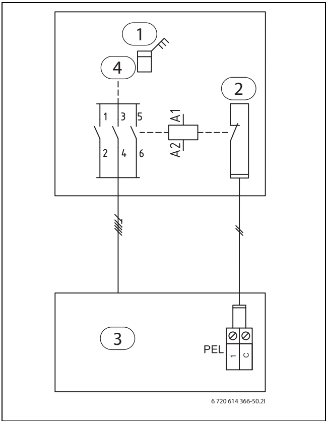
Bild 28 Sperrzeit aktiv
