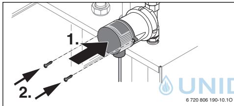
Bild 5 Anschlussdose montieren
