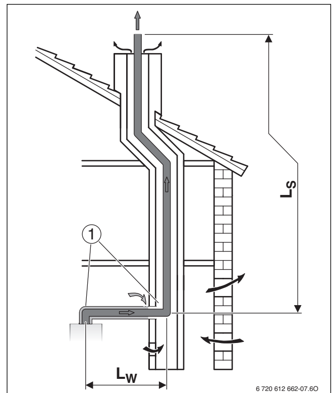
Bild 11 Abgasführung im Schacht nach B 33x
