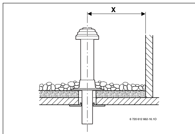
Bild 6 Abstandsmaße bei Flachdach
