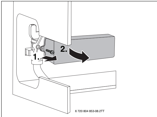
Bild 57 Plattenwärmetauscher ausbauen
