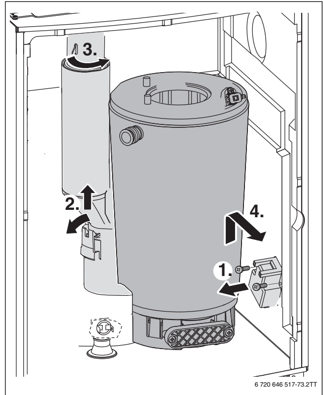
Bild 71 Wärmeblock ausbauen
