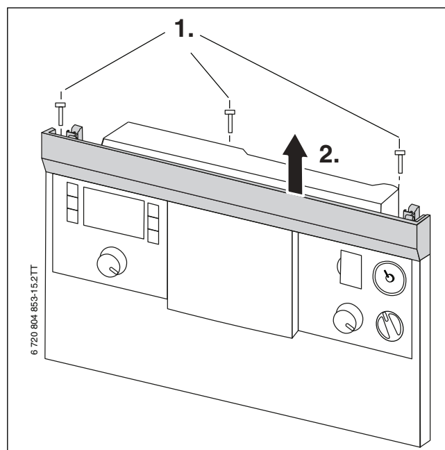
Bild 27 Abdeckung entfernen
