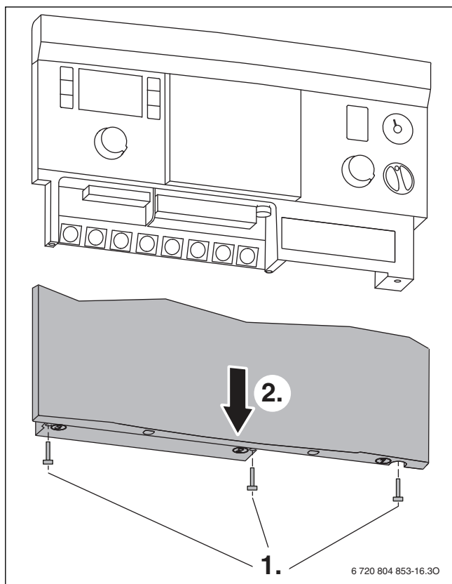
Bild 29 Abdeckung entfernen
