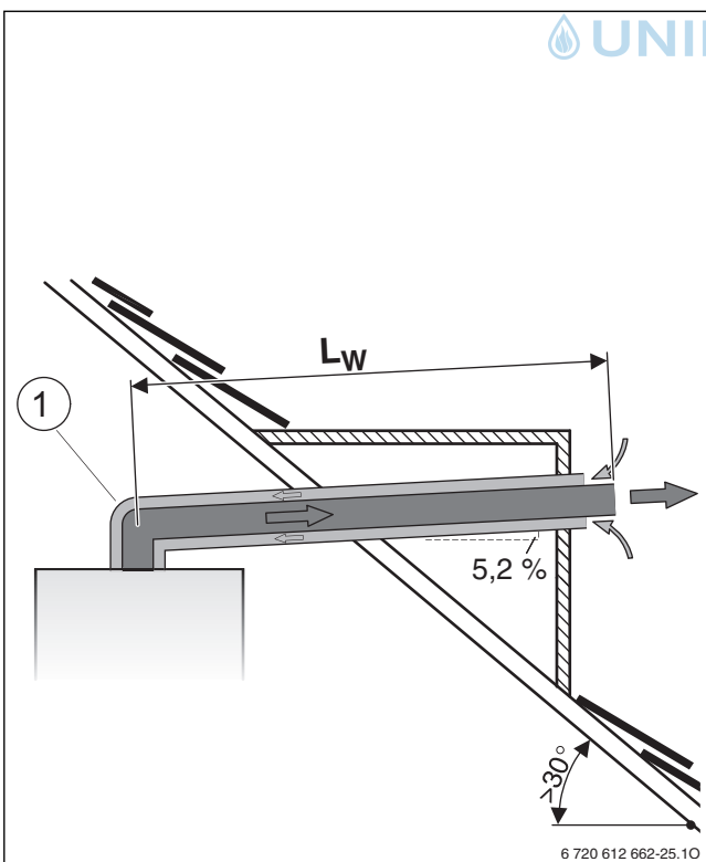
Bild 17 Abgasführung waagerecht nach C 33x (Ø 80/125 mm)
