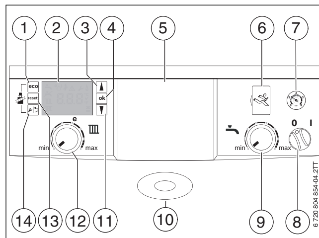
Bild 32 Bedienfeld bei geöffneter Bedienfeldblende
