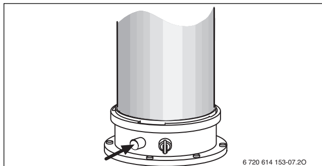
Bild 35 Abgasmessstutzen
