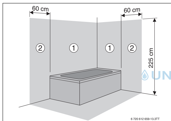
Bild 26 Schutzbereiche
