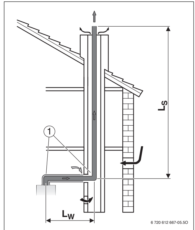
Bild 10 Abgasführung im Schacht nach B 33x
