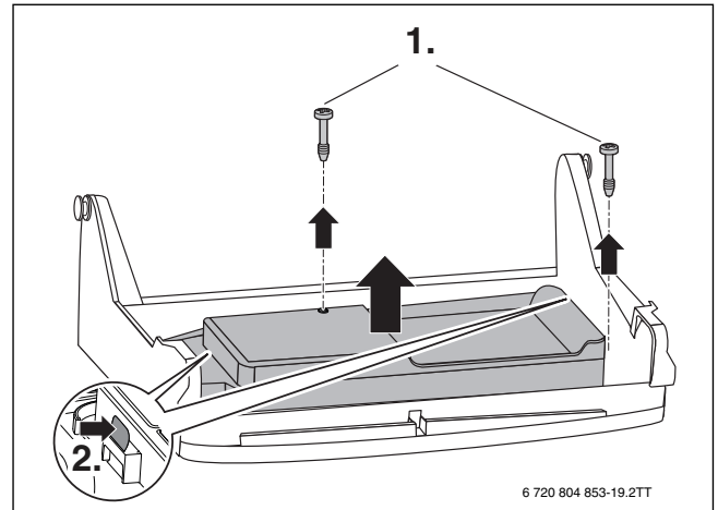
Bild 67 Abdeckung entfernen
