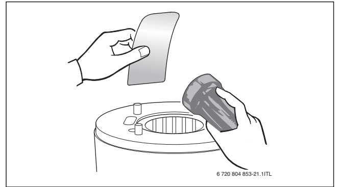
Bild 51 Wärmeblock auf Rückstände prüfen
