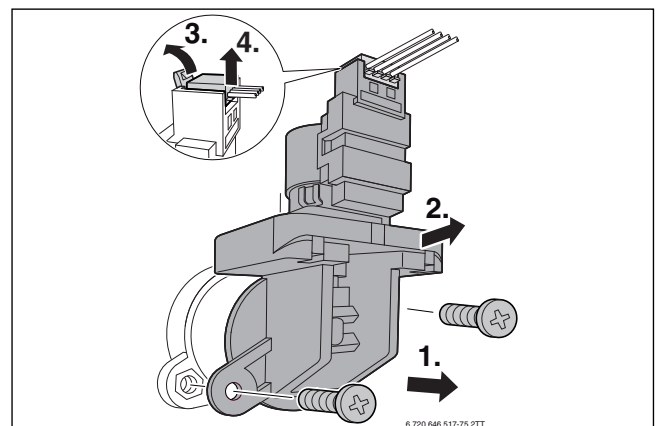
Bild 60 3-Wege-Ventil ausbauen
