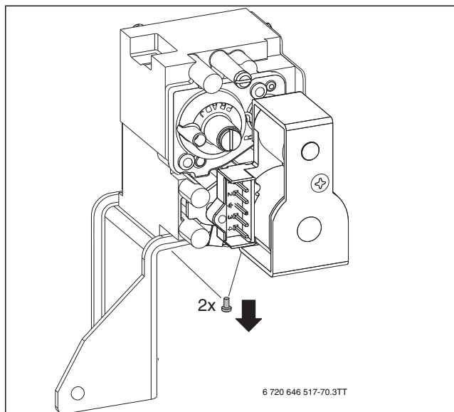
Bild 63 Gasarmatur ausbauen
