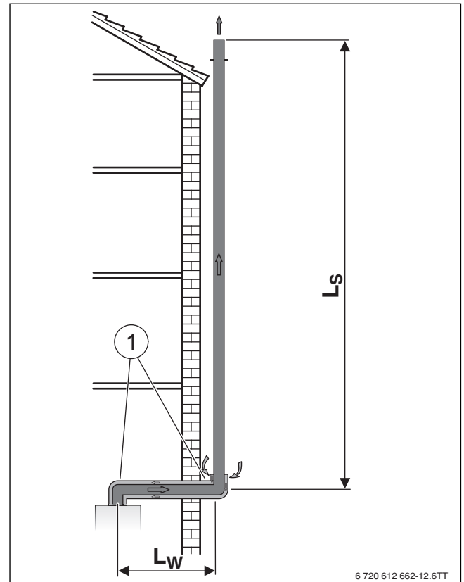
Bild 18 Abgasführung an der Fassade nach C 53x
