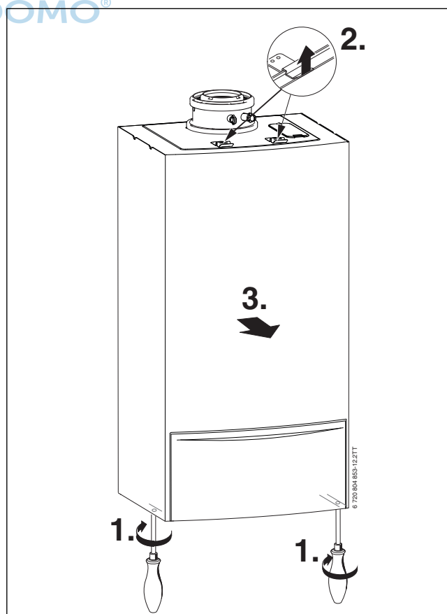
Bild 22 Verkleidung abnehmen
