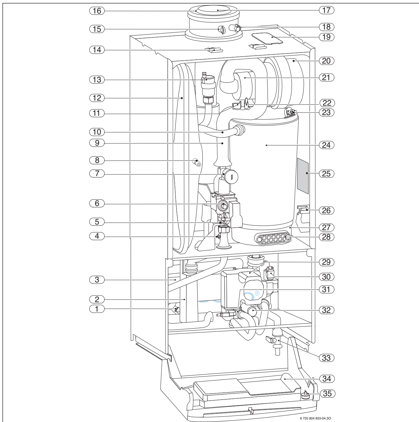
Bild 3 Produktübersicht
