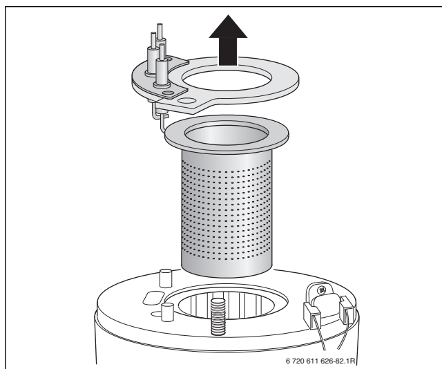
Bild 47 Brenner herausnehmen
