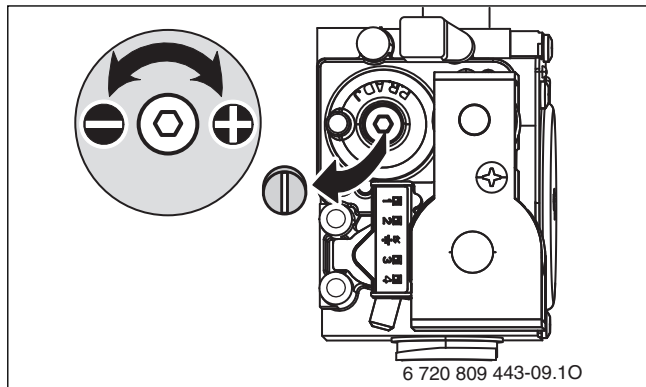
Bild 39 Plombe an der Gasarmatur entfernen
