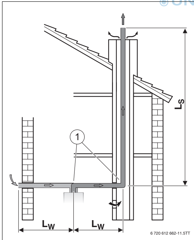
Bild 13 Abgasführung im Schacht nach C 53x
