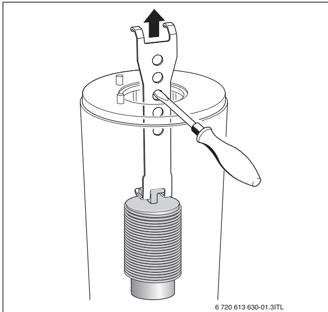
Bild 49 Unteren Verdrängungskörper herausnehmen
