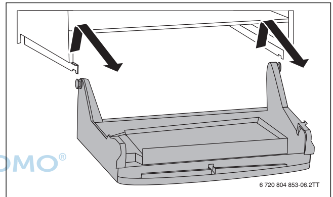
Bild 68 Steuergerät aushängen
