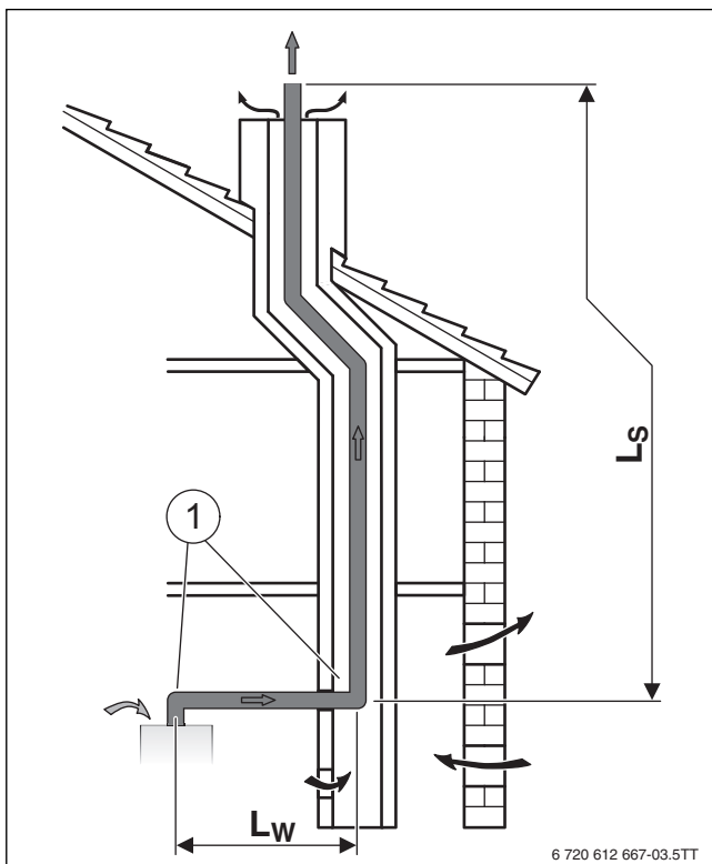
Bild 9 Abgasführung im Schacht nach B 23
