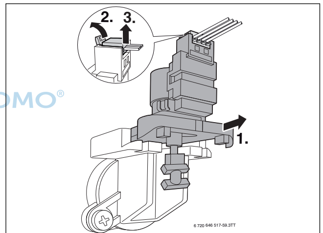
Bild 59 Motor des 3-Wege-Ventils ausbauen
