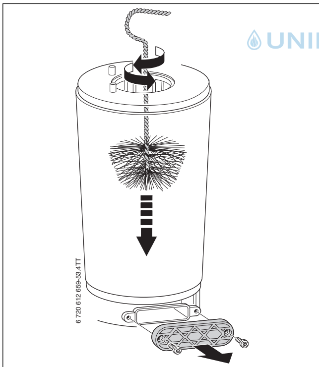
Bild 50 Wärmeblock reinigen
