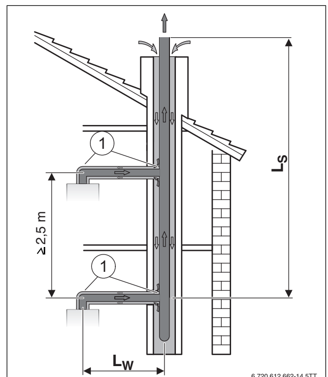
Bild 19 Mehrfachbelegung mit konzentrischem Rohr nach C 43x
