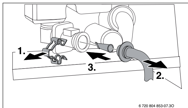
Bild 55 Sieb aus Kaltwasserrohr ausbauen
