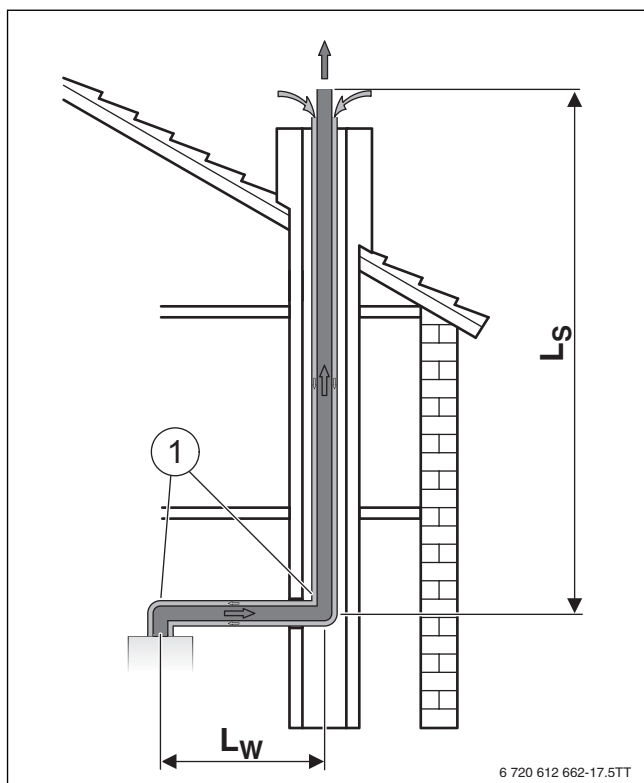
Bild 12 Abgasführung mit konzentrischem Rohr im Schacht nach C 33x
