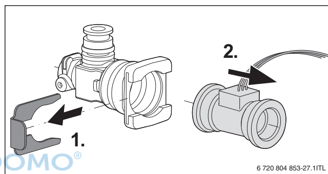
Bild 56 Turbine am Kaltwasserrohr ausbauen
