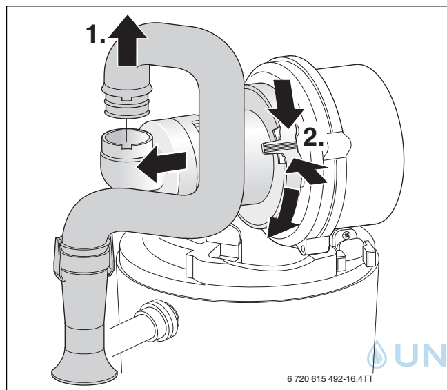
Bild 45 Saugrohr und Mischeinrichtung ausbauen
