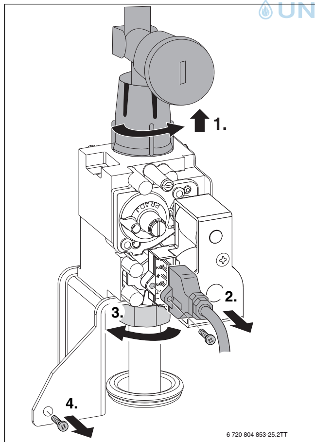
Bild 62 Gasarmatur ausbauen
