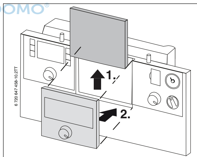
Bild 28 Abdeckung entfernen und Heizungsregler montieren
