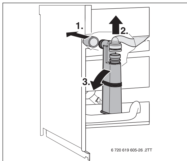
Bild 53 Kondensatsiphon ausbauen
