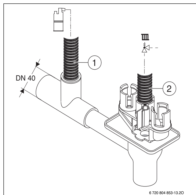
Bild 25 Kondensatschlauch und Schlauch vom Sicherheitsventil am Siphon montieren
