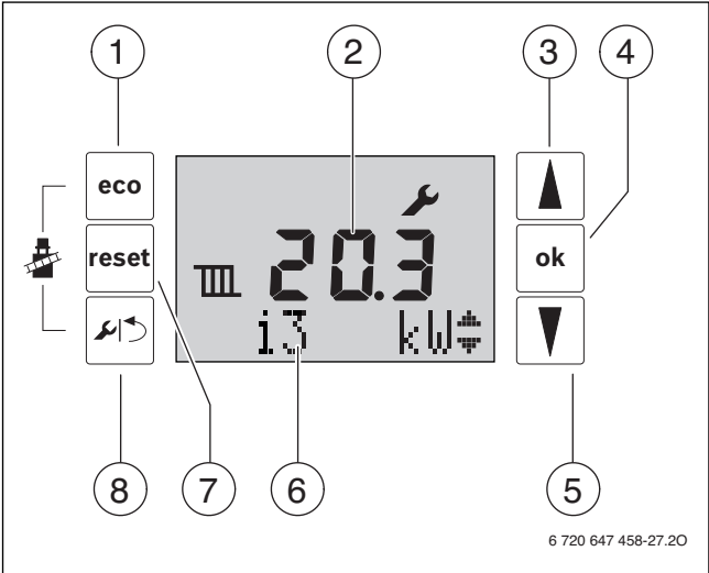
Bild 34 Übersicht der Bedienelemente
