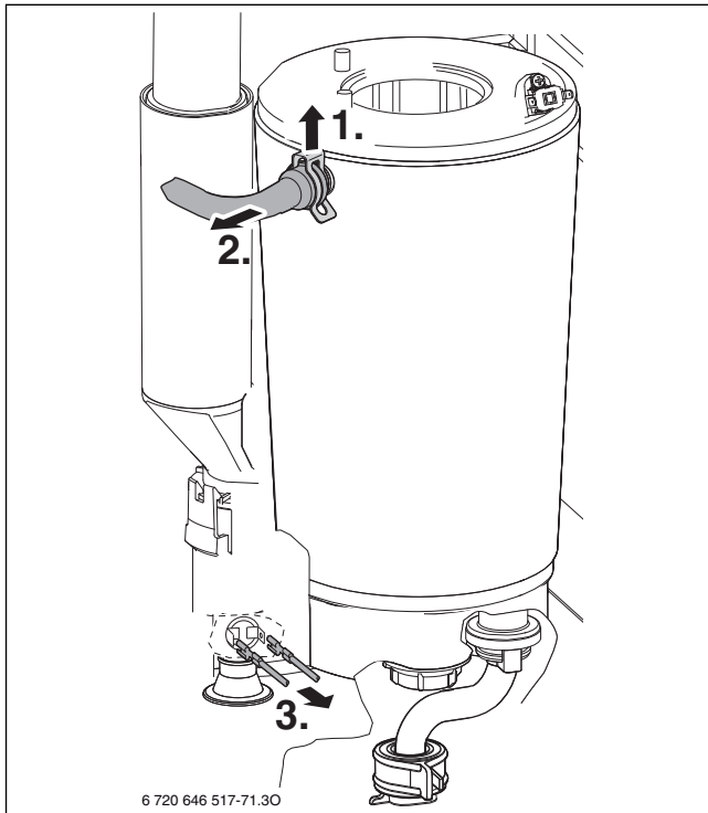
Bild 69 Vorlaufrohr lösen und Kabel abziehen
