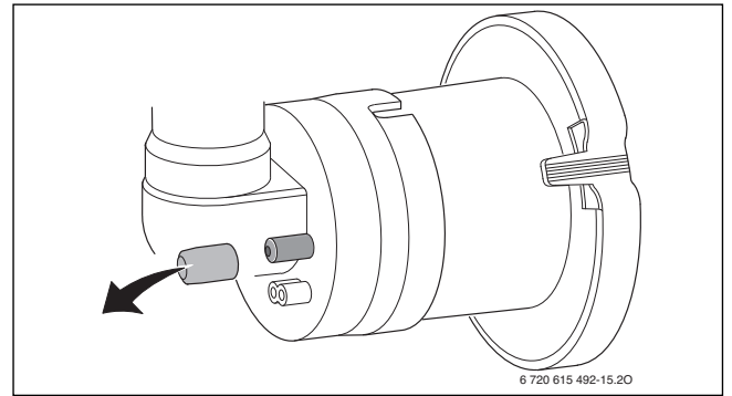
Bild 44 Messstutzen an der Mischeinrichtung
