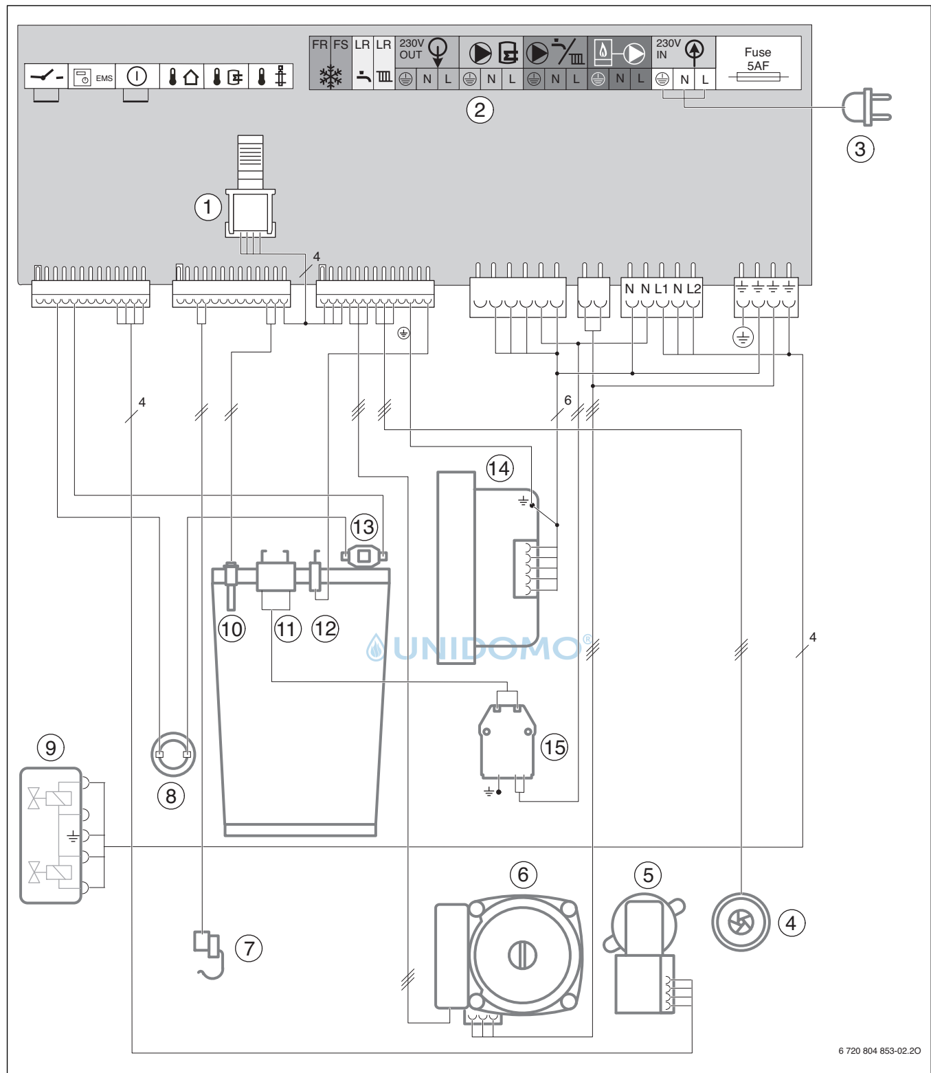
Bild 4 Elektrische Verdrahtung
