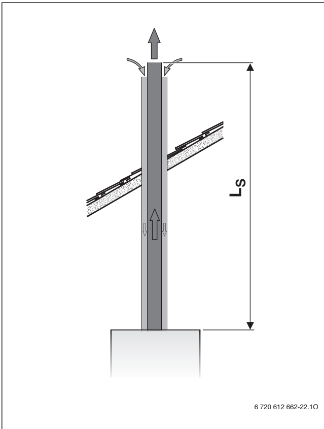
Bild 16 Abgasführung senkrecht nach C 33x
