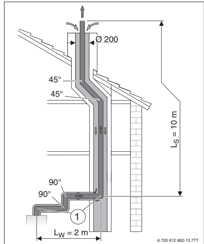
Bild 20 Einbausituation einer Abgasführung nach C 93x
