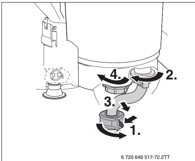
Bild 70 Mutter entfernen und Rücklaufrohr lösen
