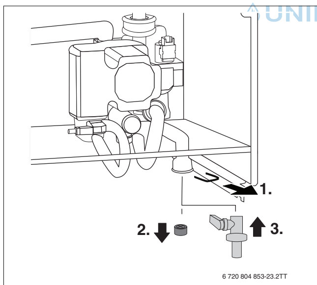
Bild 24 Füll- und Entleerhahn montieren
