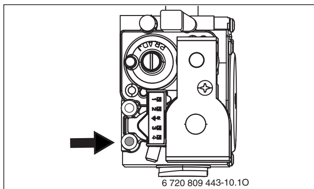
Bild 40 Messstutzen für Gas-Anschlussdruck
