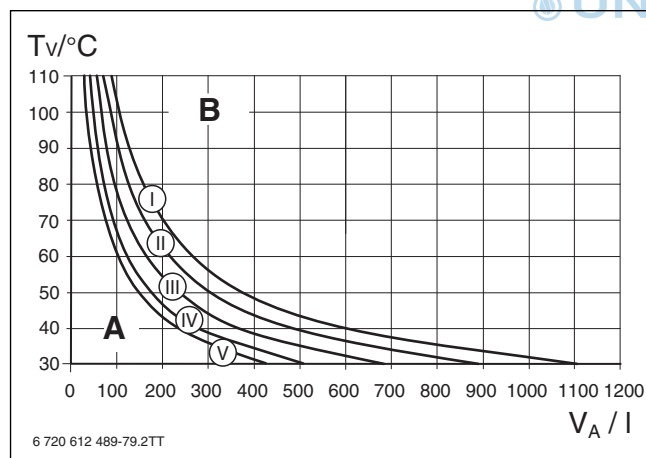
Bild 21 Kennlinien des Ausdehnungsgefäßes
