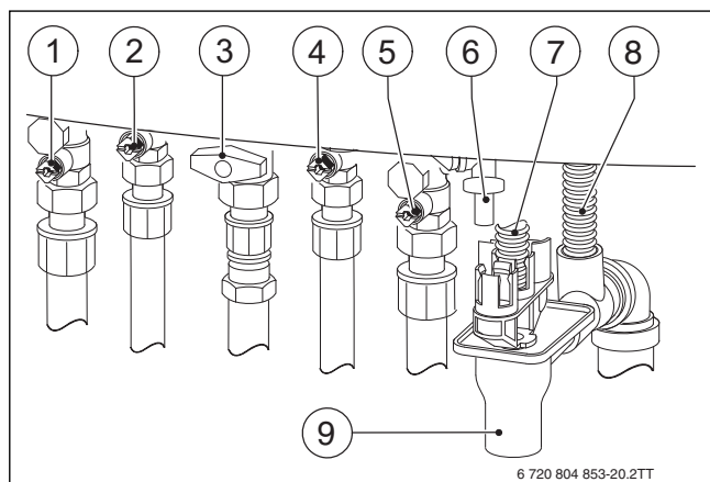
Bild 31 Gas- und wasserseitige Anschlüsse (Zubehör)
