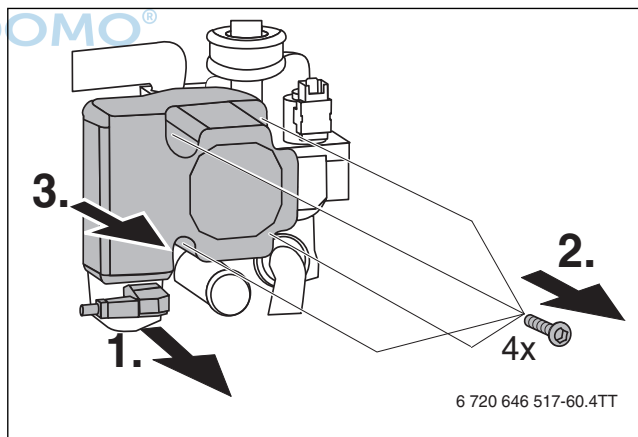
Bild 64 Heizungspumpe ausbauen
