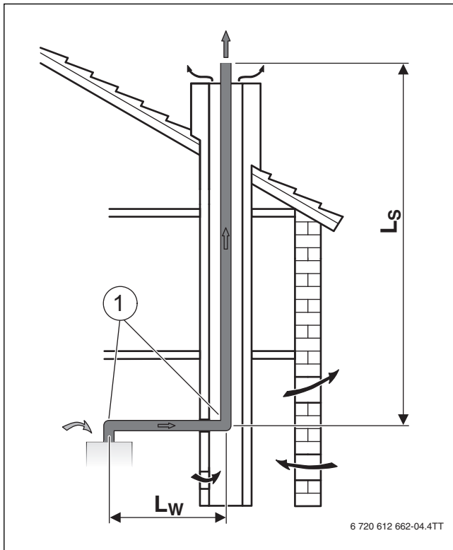
Bild 8 Abgasführung im Schacht nach B 23
