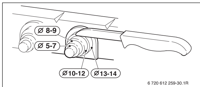
Bild 30 Zugentlastung an Kabeldurchmesser anpassen
