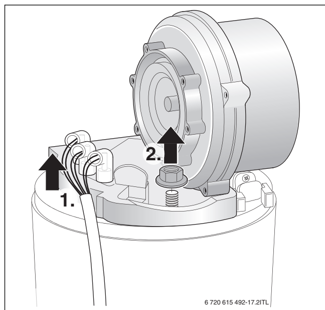
Bild 46 Gebläse herausnehmen
