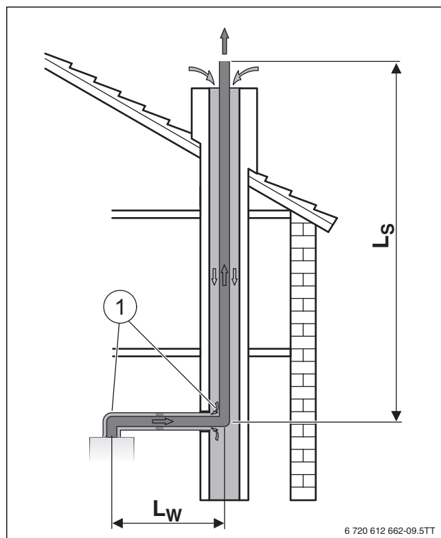
Bild 14 Abgasführung im Schacht nach C 93x
