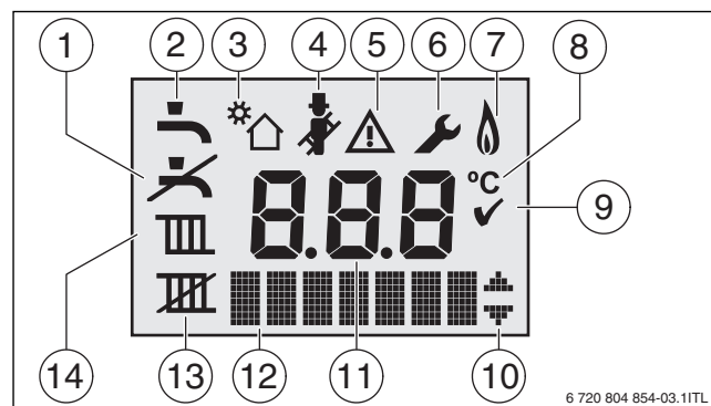
Bild 33 Displayanzeigen
