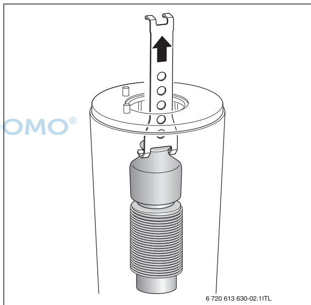
Bild 48 Oberen Verdrängungskörper herausnehmen
