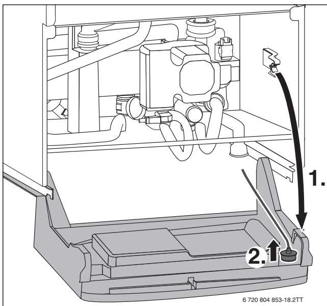
Bild 66 Steuergerät nach unten klappen
