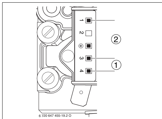
Bild 61 Messstellen an der Gasarmatur
