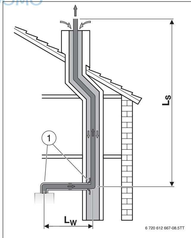
Bild 15 Abgasführung im Schacht nach C 93x
