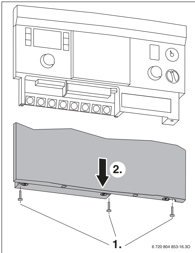
Bild 65 Abdeckung entfernen
