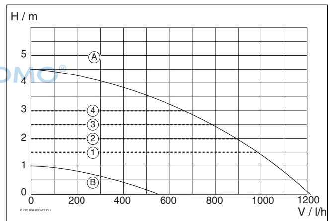
Bild 74 Pumpenkennfelder und Pumpenkennlinien
