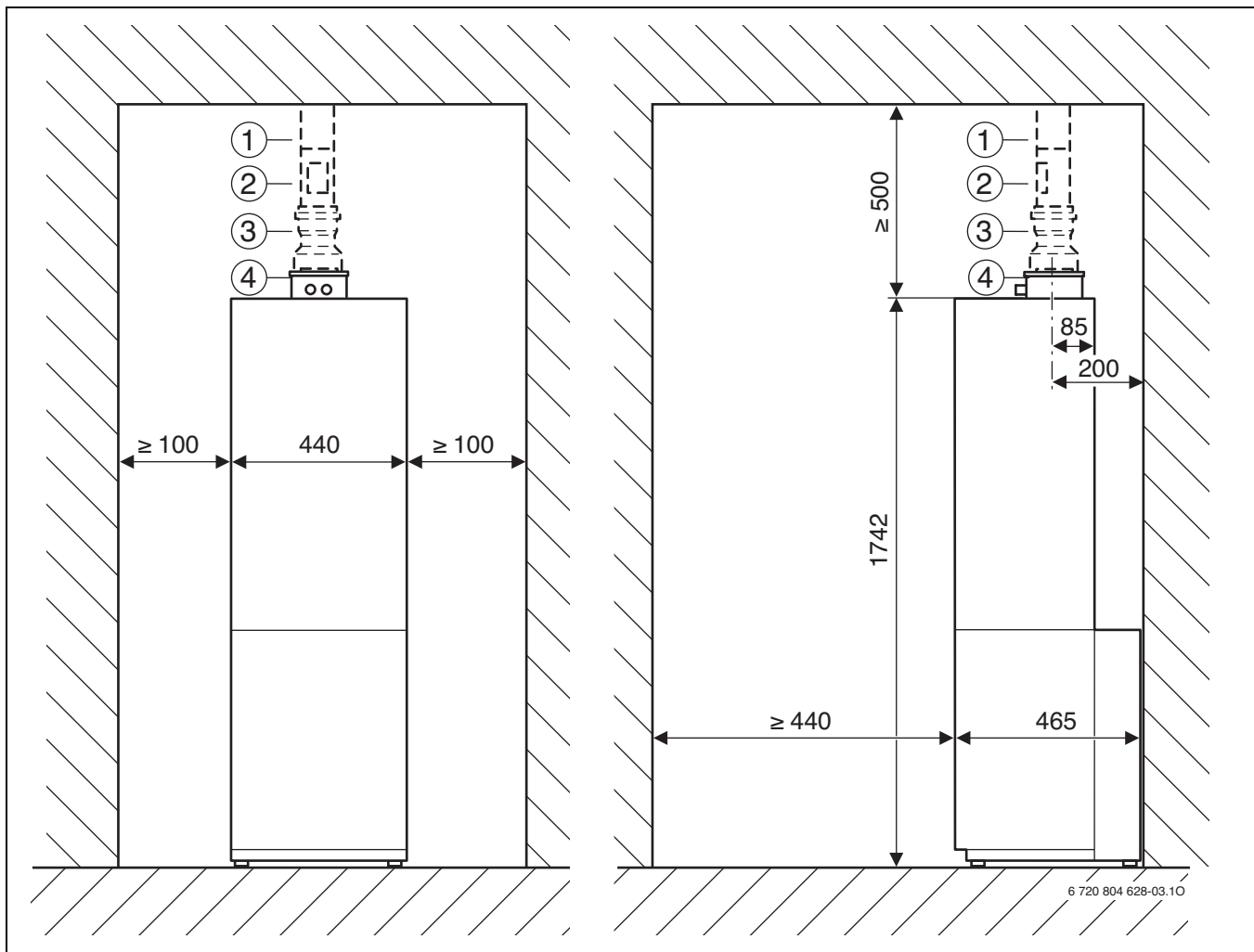
Bild 7 Flachdach
