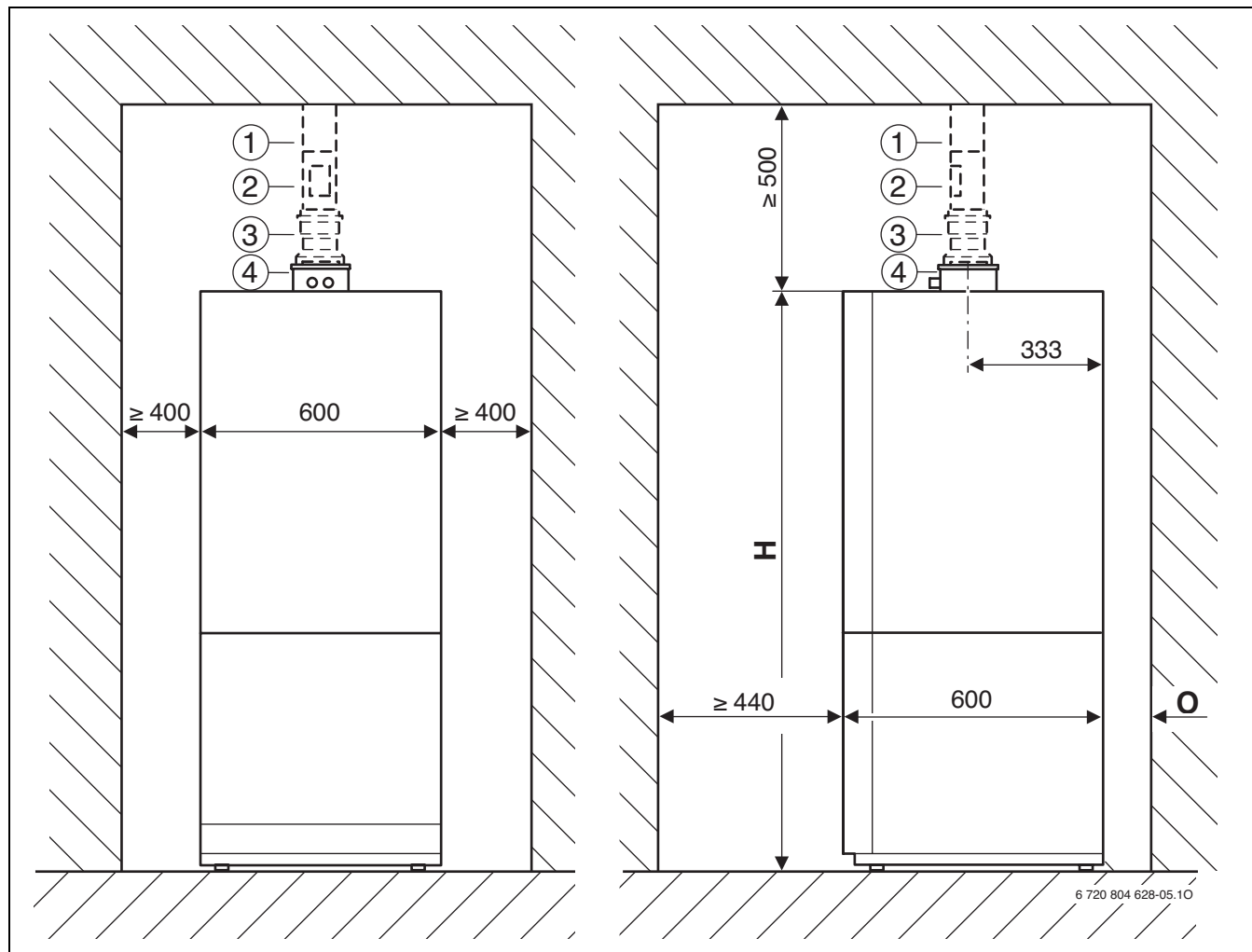
Bild 9 Flachdach
