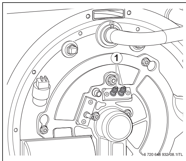
5. ábra Gyújtóelektroda
