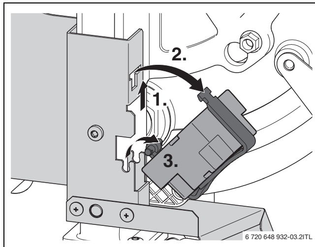
Fig. 6 Retirer le transformateur d'allumage
