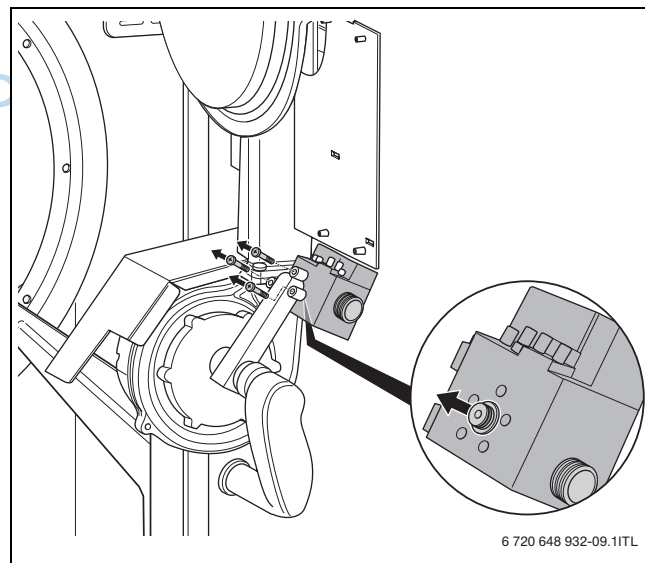
Fig. 12 Sostituzione ugello del gas
