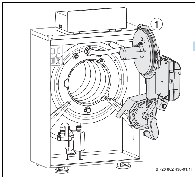
Obr. 13 O-kružok v kryte horáka
