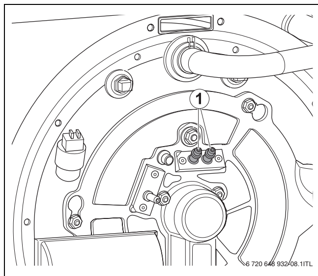
Fig. 5 Electrode d'allumage
