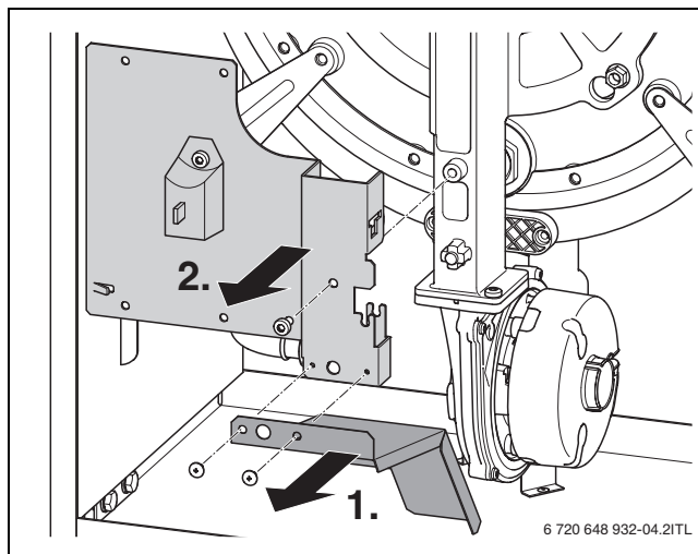
Rys. 7 Demontaż osłony przed kapieniem i wsporników blaszanych
