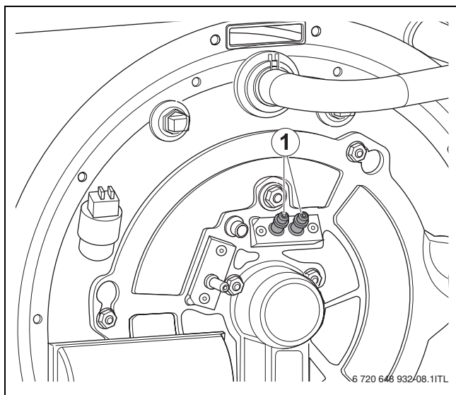
Bild 5 Zündelektrode
