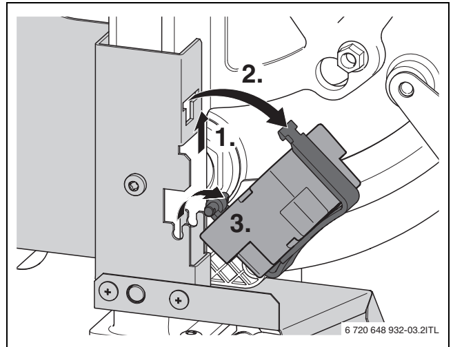
Afb. 6 Ontstekingsstrafo verwijderen
