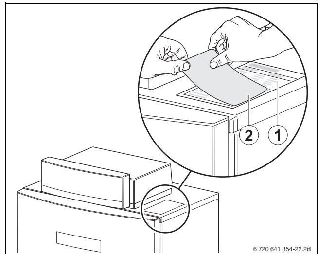
14. ábra Adattábla aktualizálása
