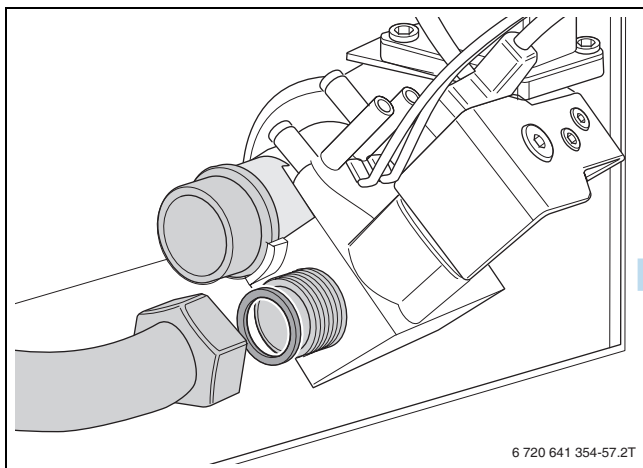
Fig. 9 Soltar as uniões rosçadas no dispositivo de controlo do gás
