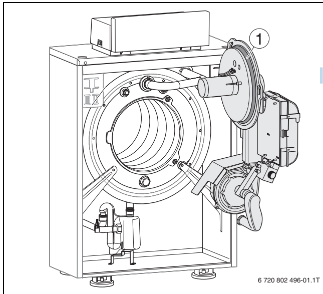
Afb. 13 O-ring branderhuis
