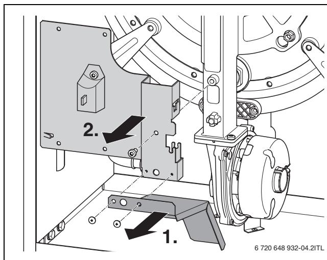
Fig. 7 Démonter le tôle anti-goutte et les plaques de jonction
