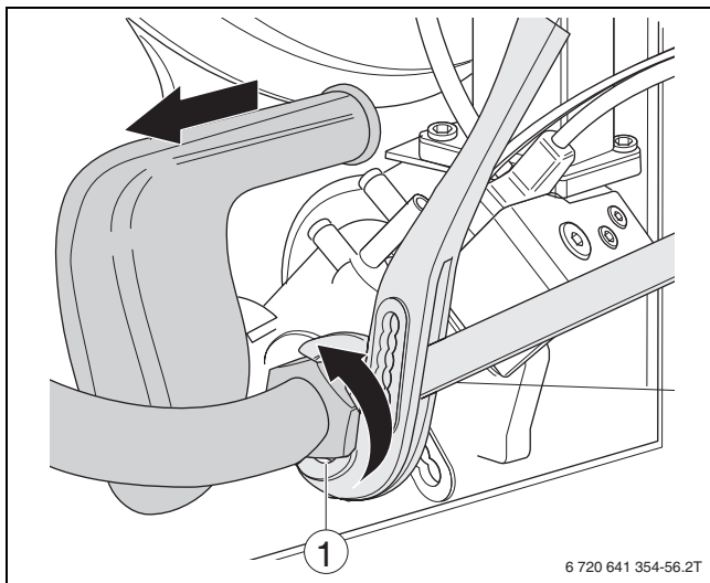
Fig. 8 Soltar as uniões rosçadas no dispositivo de controlo do gás (imagem exemplificativa da caldeira de 22 kW)
