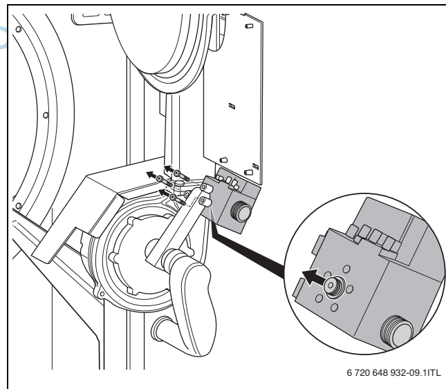
Rys. 12 Wymiana dyszy gazowej
