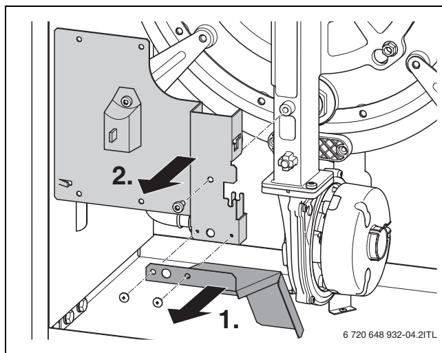
Fig. 7 Desmontar a chapa de proteção anti-gotas e as chapas de fixação
