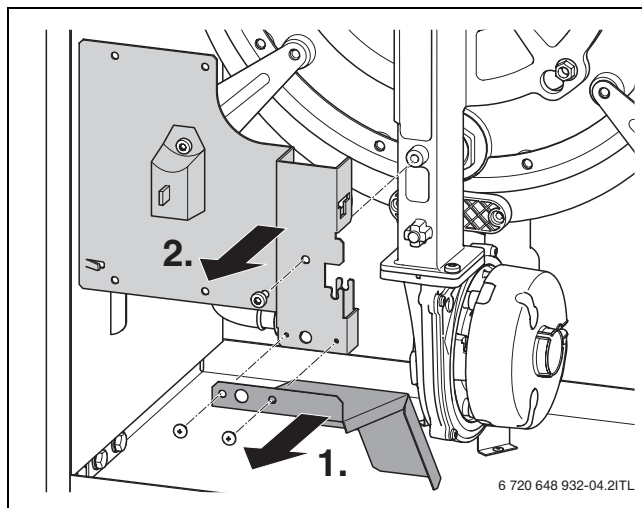
Fig. 7 Smontaggio di lamiera di protezione dallo sgocciolamento lamiera di bloccaggio
