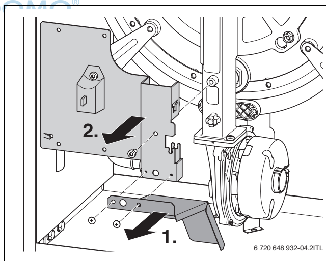
Bild 7 Tropfschutzblech und Haltebleche demontieren
