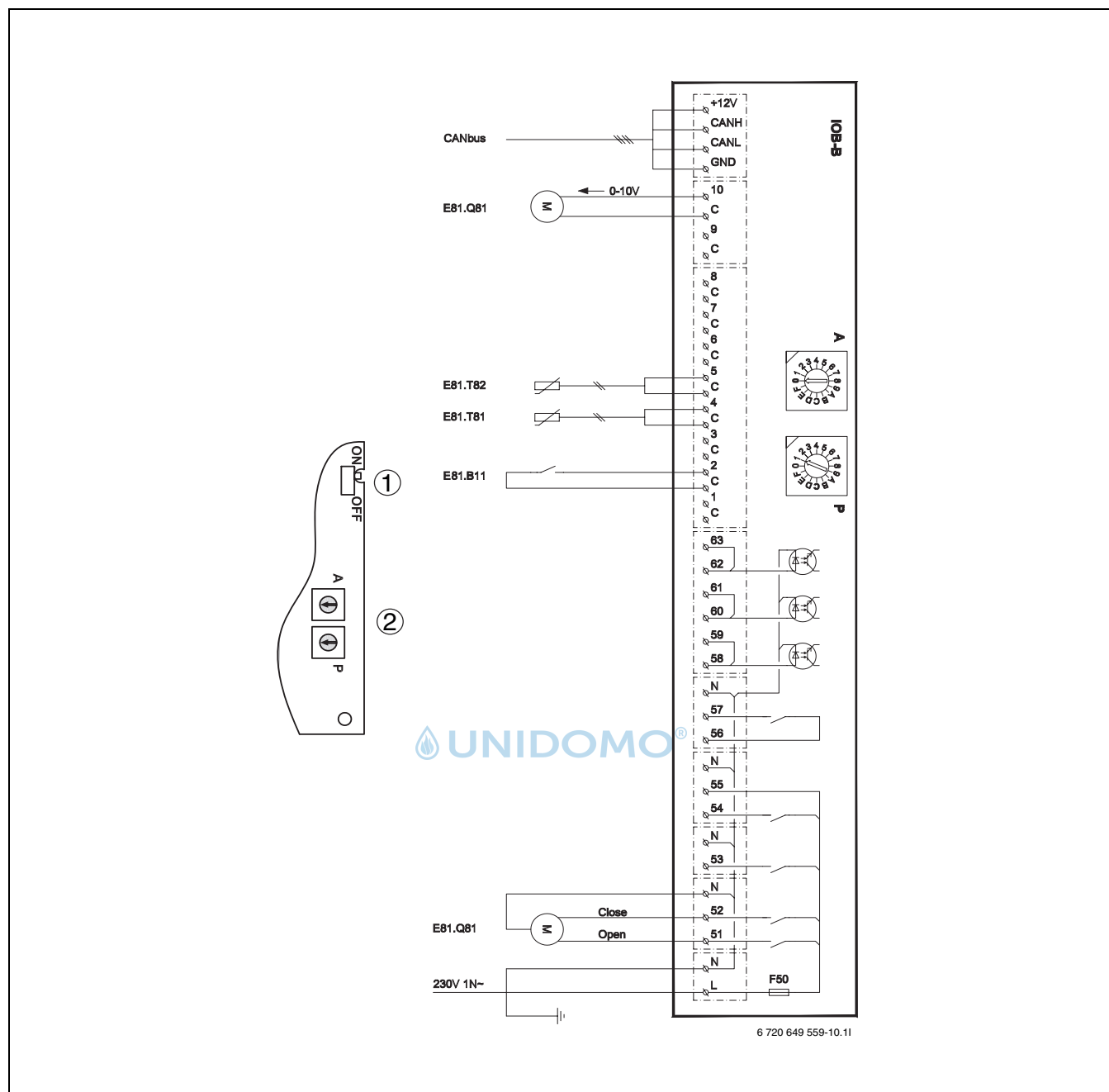
Bild 23 Schaltplan Schwimmbadsteuerung
