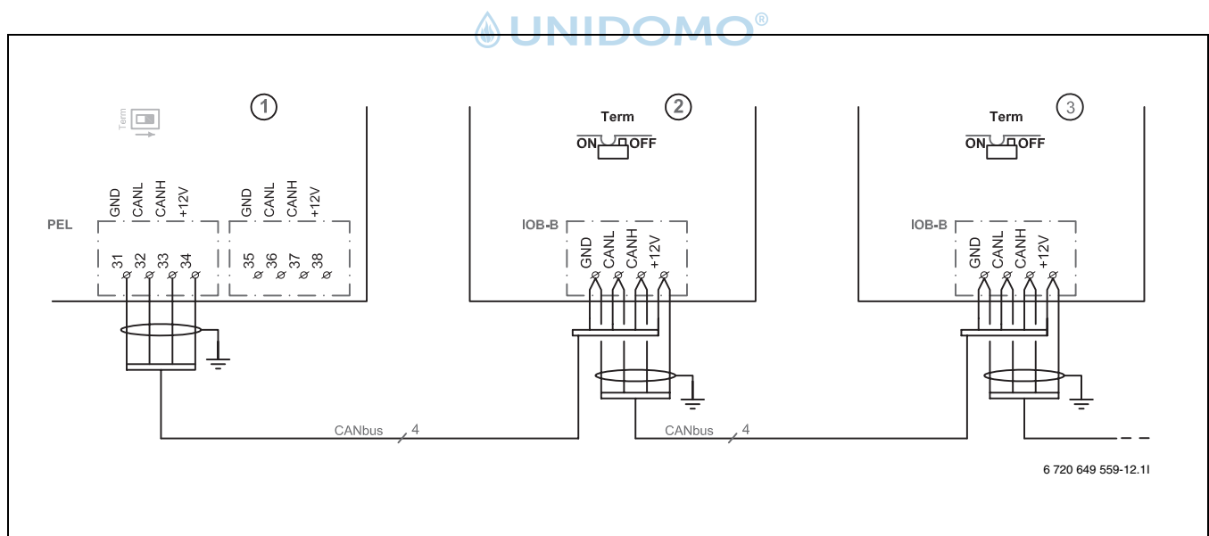
Bild 9 CANbus-Anschlüsse zwischen Steuerschrank, SEM-1 und Wärmepumpe
