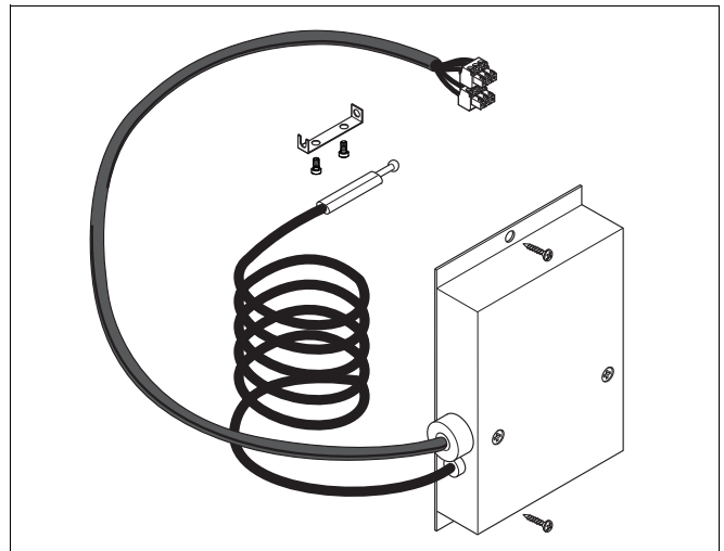
Fig. 1 Volumen de suministro AW50 Kombi
