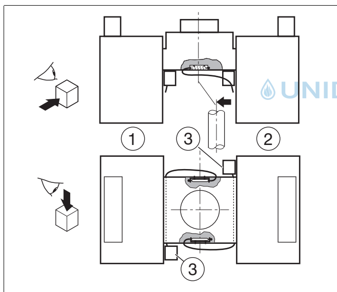
Afb. 24 2 stuks AW50 bij G334 XD.
