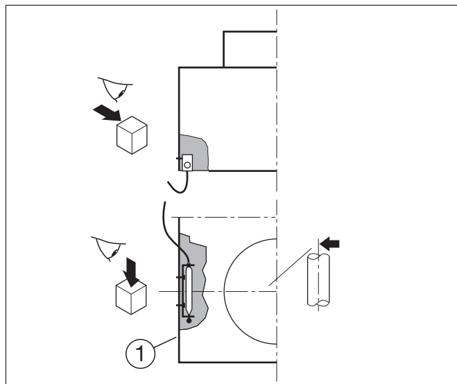
Sl. 6 Osjetnik temperature dimnih plinova G124 x/xv i Gaz 5000F - 28 / 32.
