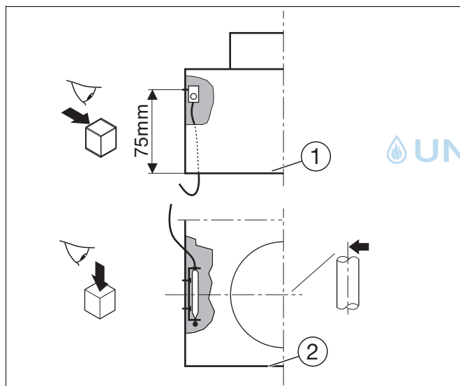
Sl. 7 Osjetnik temperature dimnih plinova G134, veličina 2 Gld.
