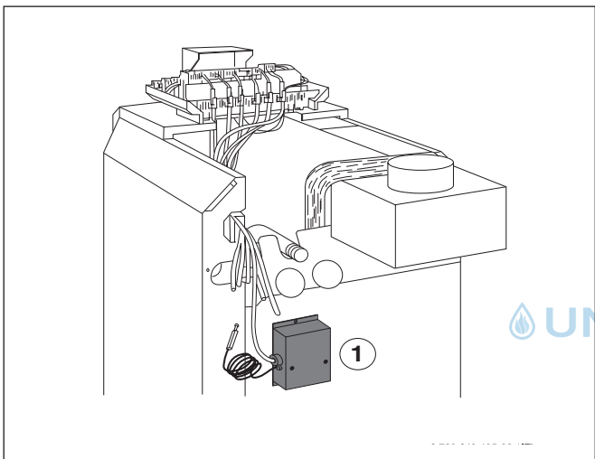
شكل 2 موضع وحدة التحكم Gaz 5000F - 28 | 32 أو G124 X
