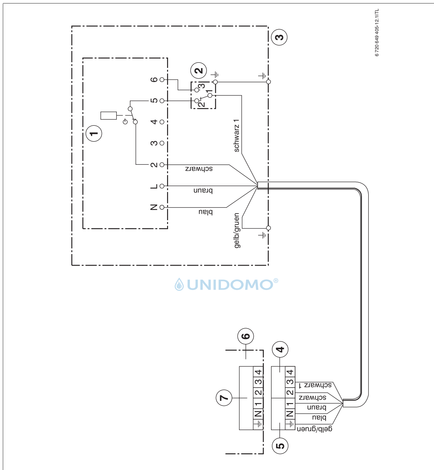
мал.12 Схема підключення для пристрою контролю відпрацьованих газів AW50.00 (дійсна для регулювального приладу HS3 220)
