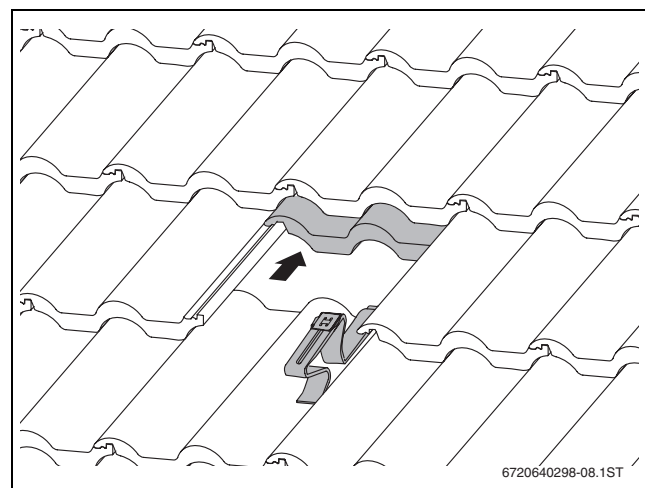
Bild 18 Eingehängter Dachhaken
