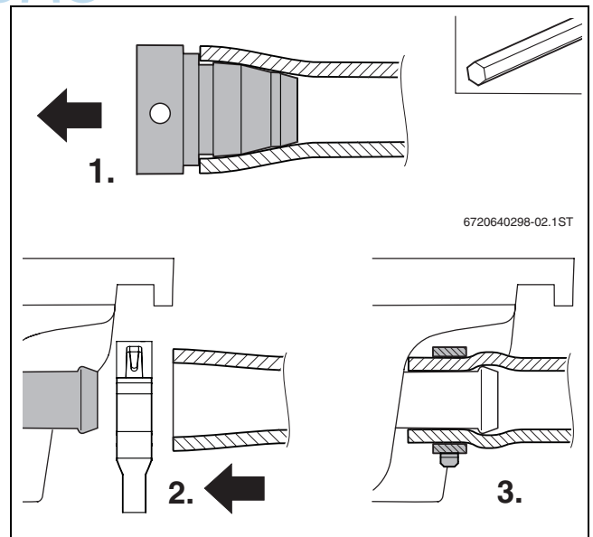
Bild 38 Montage des Solarschlau- ches
