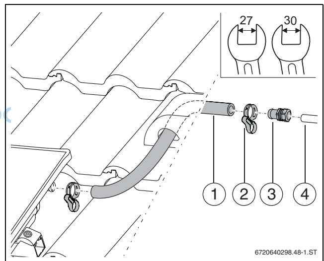
Bild 52 Solarschlauch (Vorlauf) durch das Dach führen
