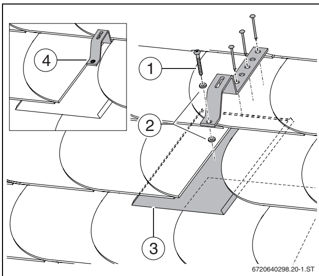
Bild 26 Beispielhafte Abdichtung
