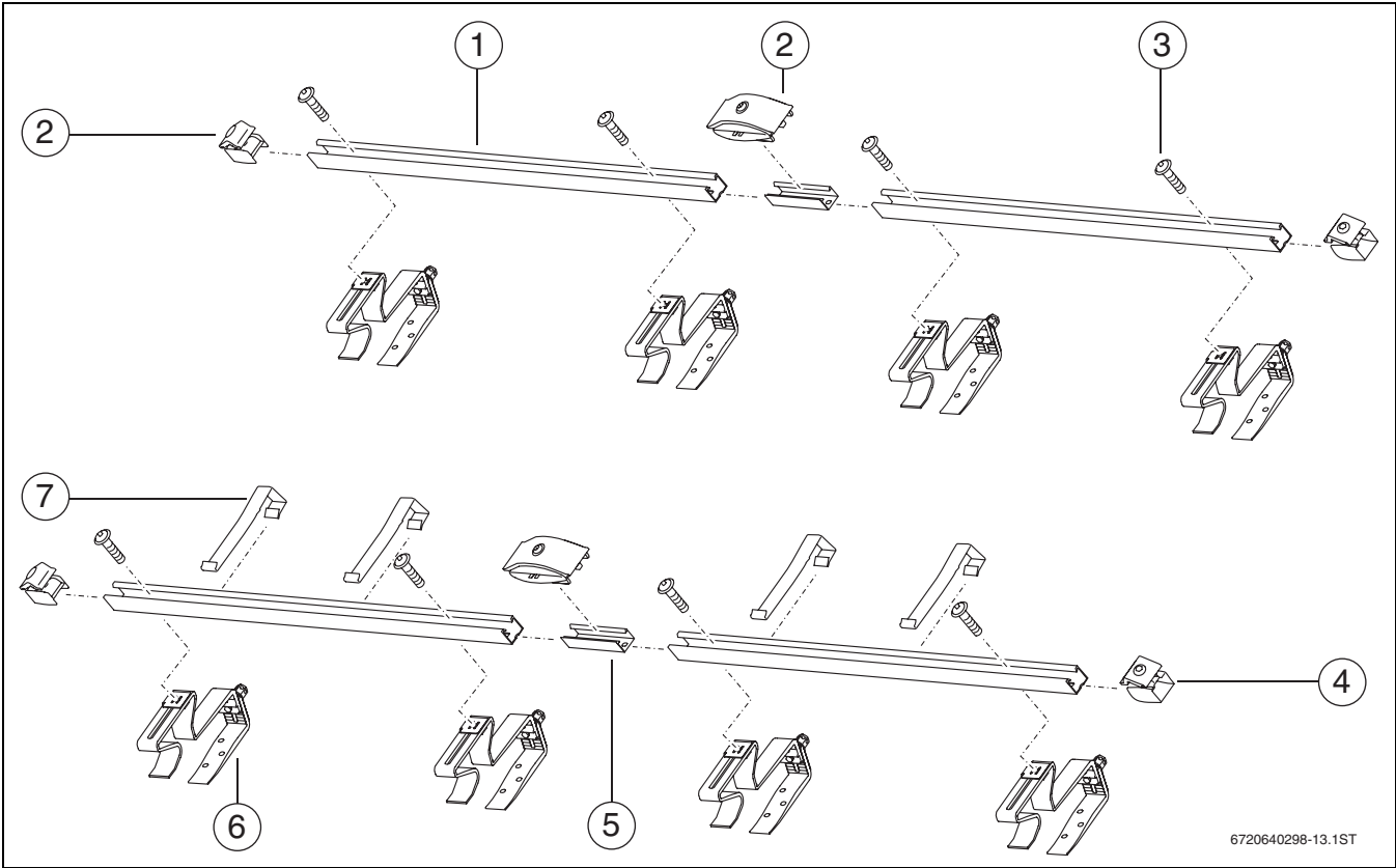
Bild 5 Montage-Set für 2 Kollektoren: 1 Montage-Set Grundauführung, 1 Montage-Set Erweiterung und 2 Montage-Sets für Dachziegel
