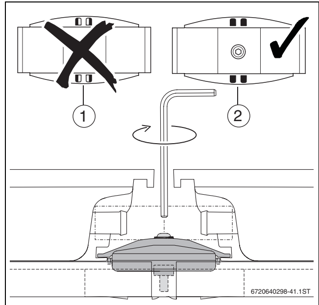
Bild 46 Doppelseitiger Kollektorspanner montiert
