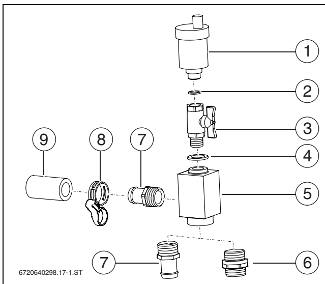
Bild 54 Lieferumfang Entlüftersatz
