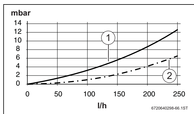
Bild 4 Druckverluste der Kollektoren
