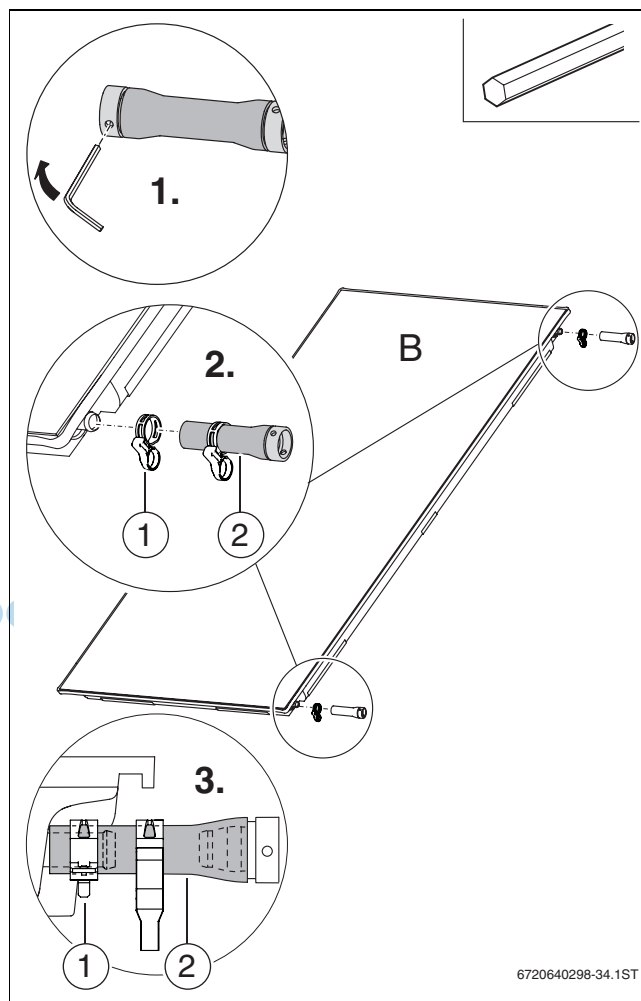
Bild 40 Verbindungs-Set am zweiten und allen weiteren Kollektoren
