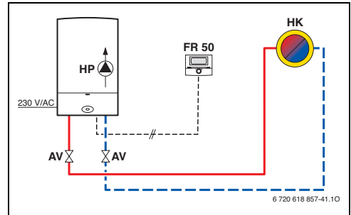
Bild 3 Vereinfachtes Anlagenschema
