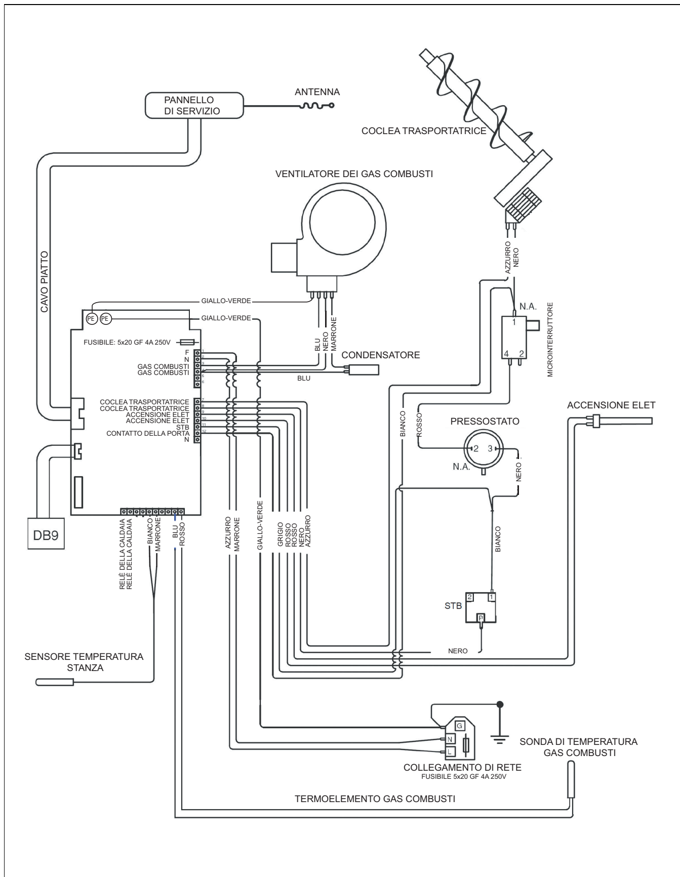
Fig. 15 Schema elettrico
