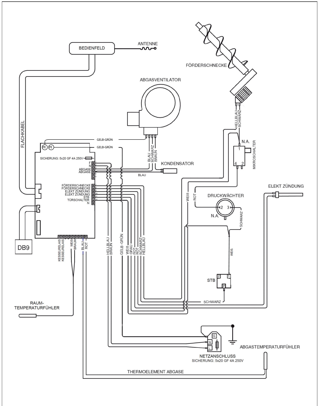
Bild 4 Schaltplan
