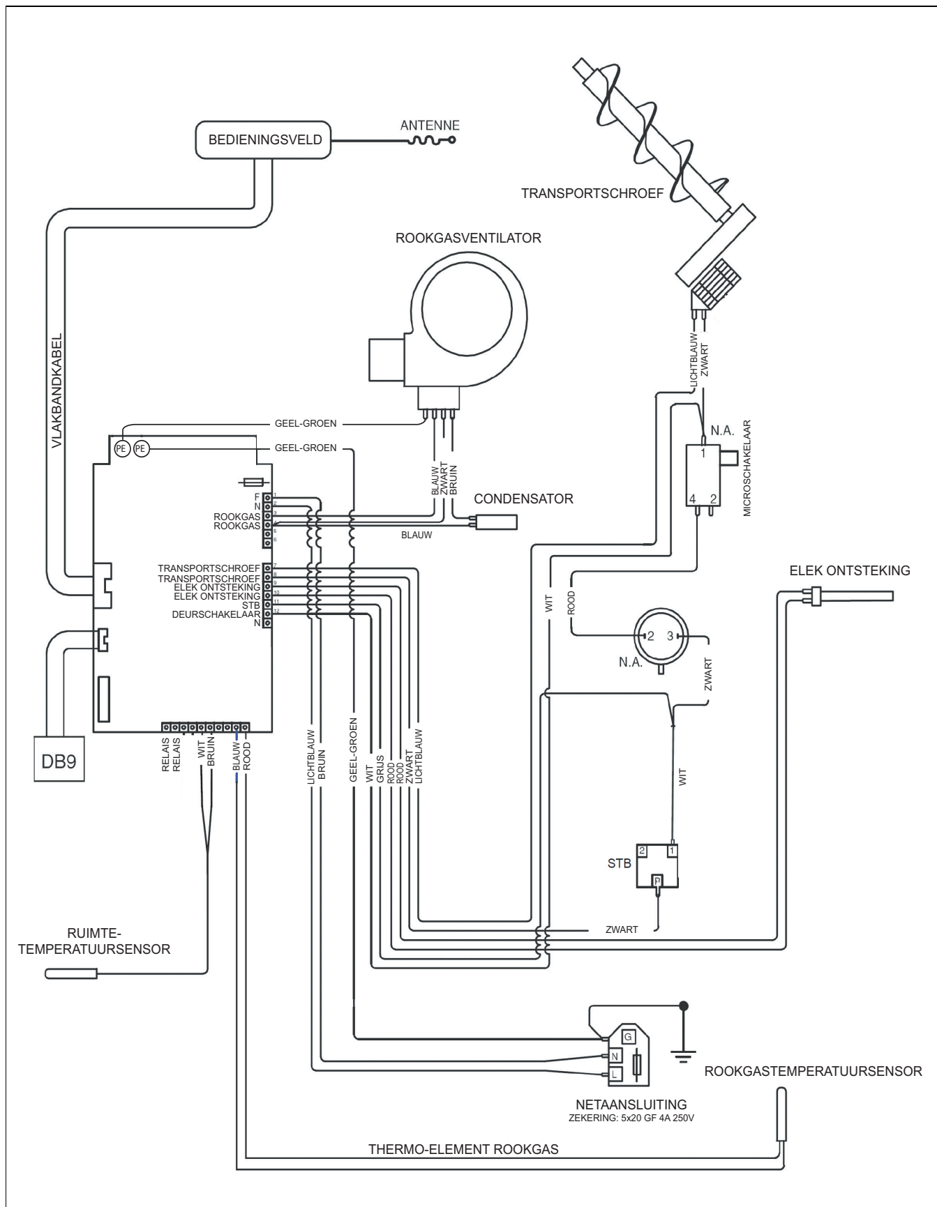
Afb. 11 Schakelschema
