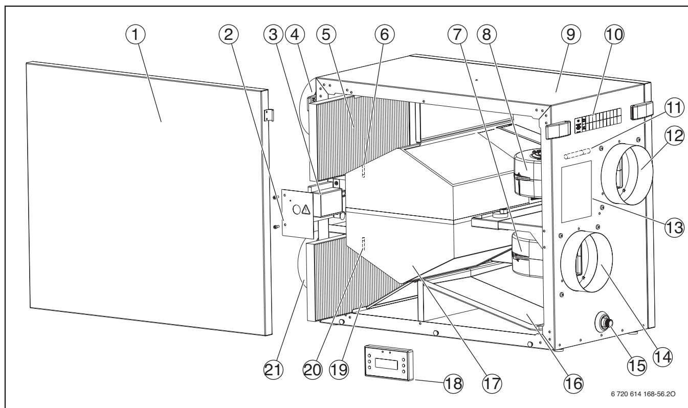
Bild 5 LP 250
