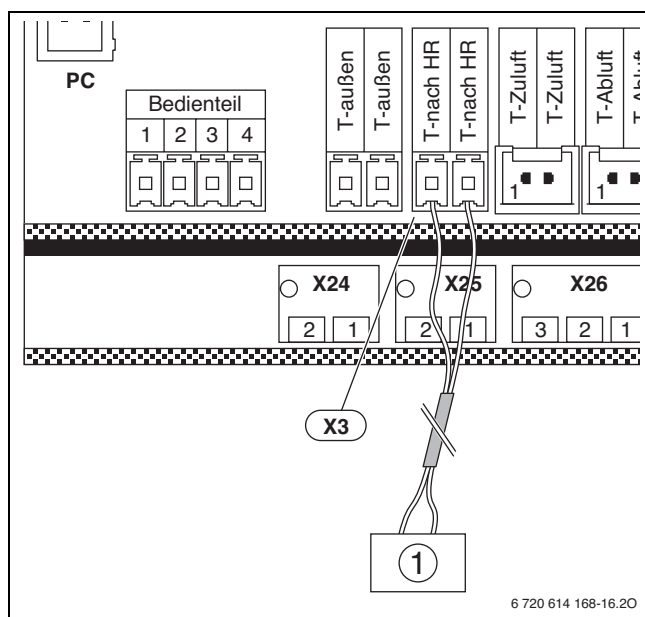
Bild 30 Klemmenbelegung Temperaturfühler für Nachheizung
