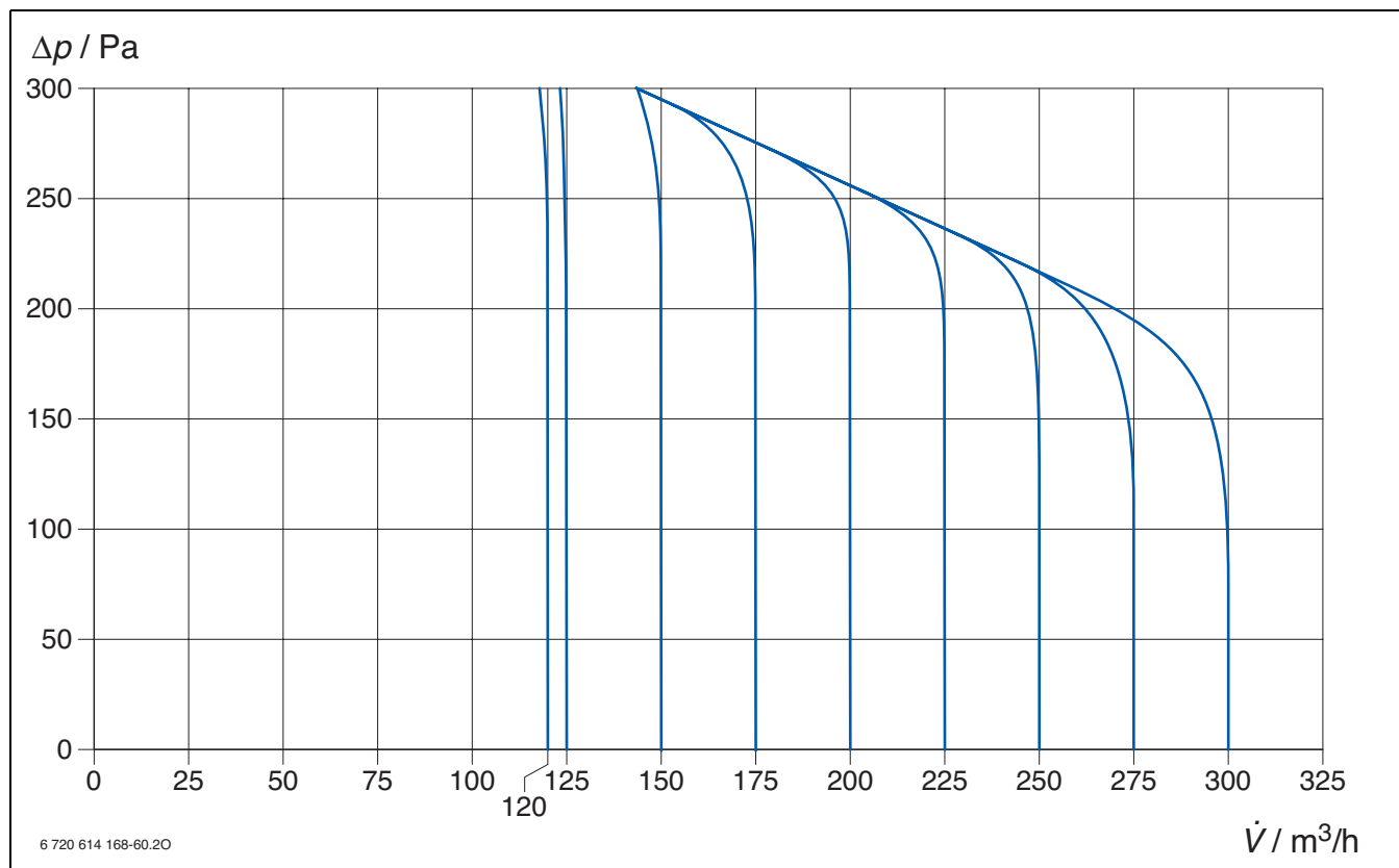
Bild 10 LP 250
