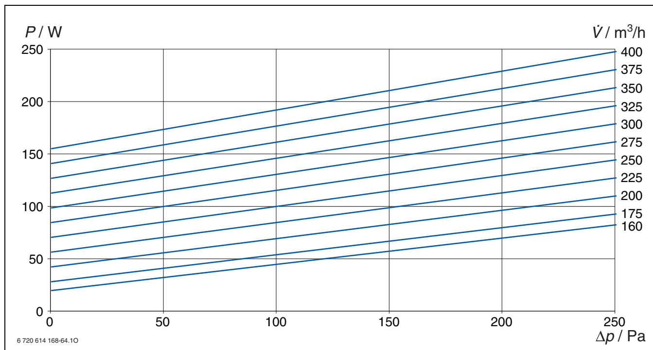
Bild 14 LP 350
