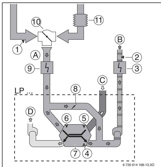
Bild 15 Funktionsprinzip
