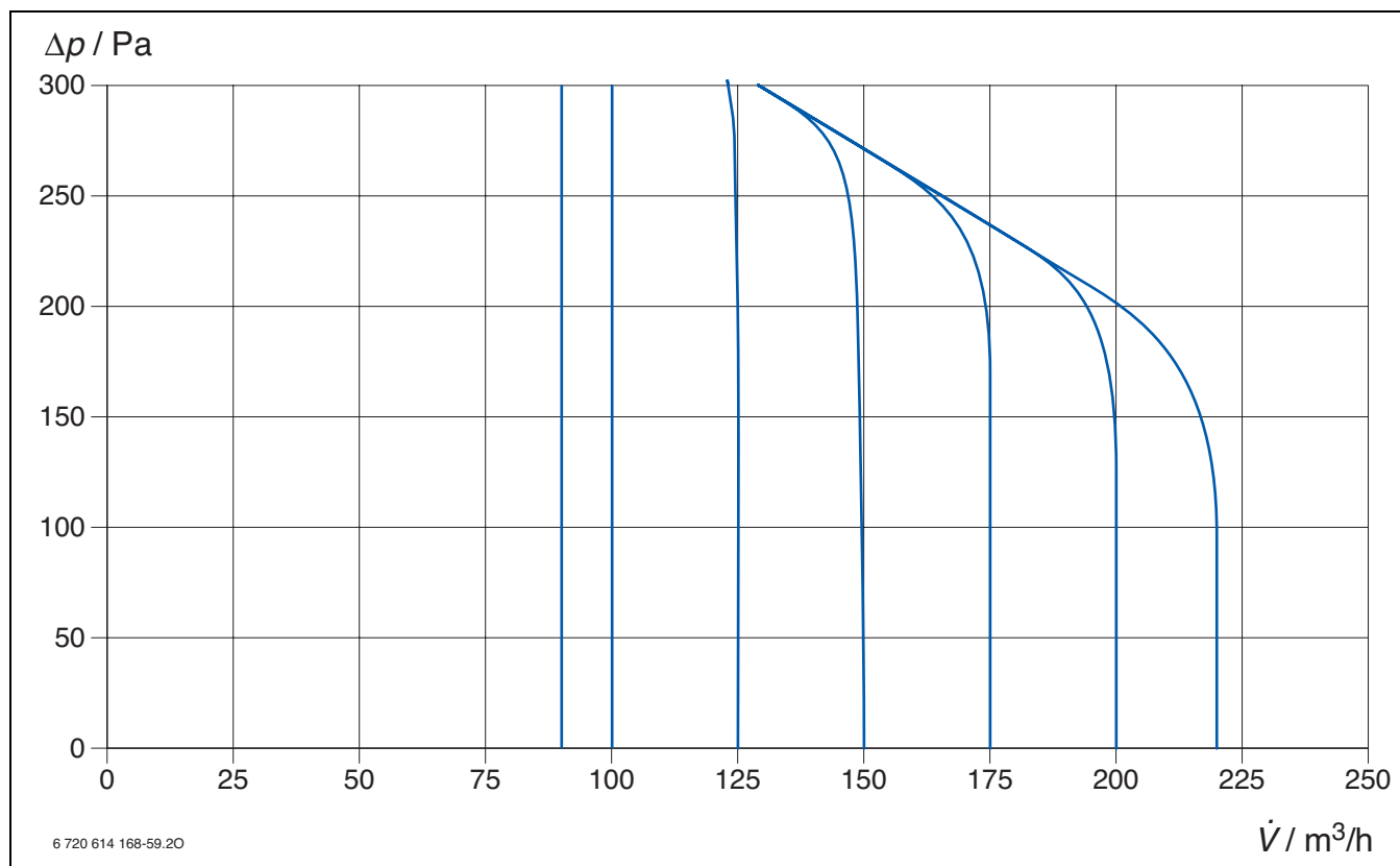
Bild 9 LP 150
