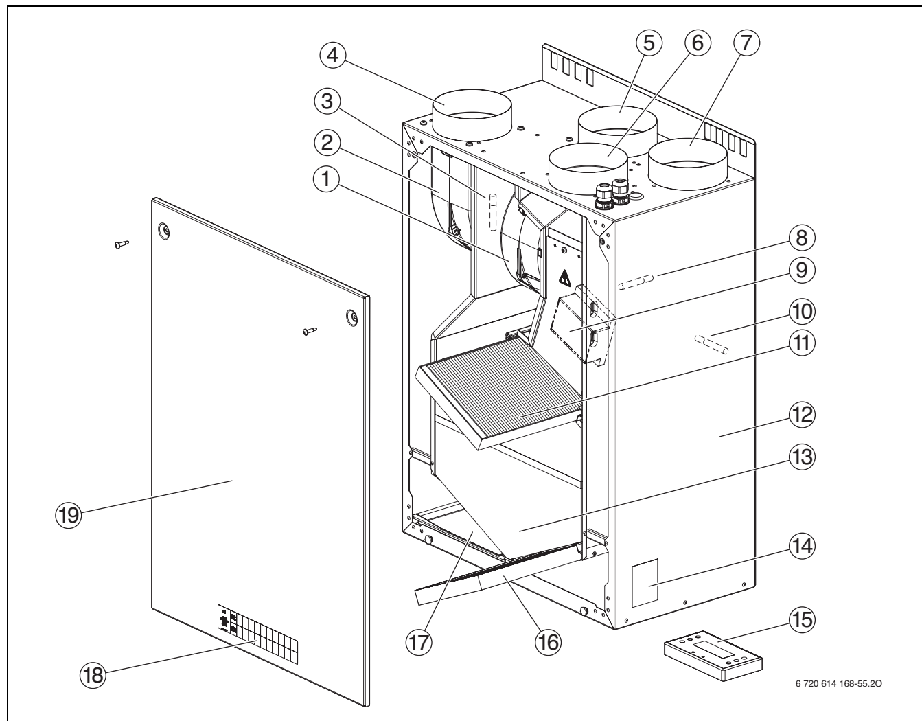
Bild 4 LP 150
