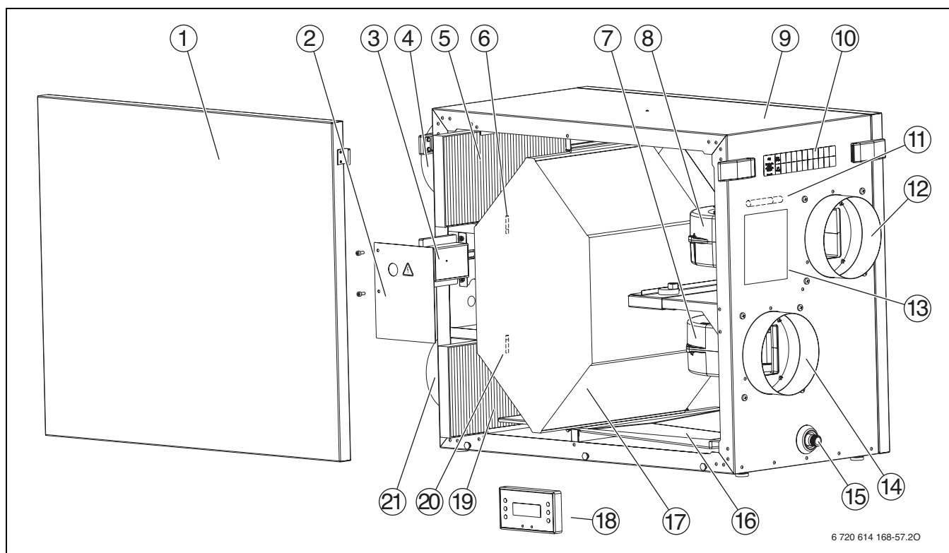
Bild 6 LP 350
