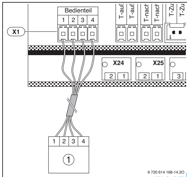
Bild 26 Klemmenbelegung Fernbedienung
