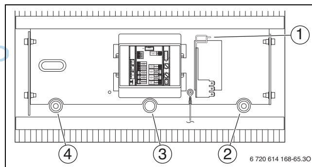
Bild 25 Erdungsanschluss und Kabeldurchführungen LP 250/LP 350
