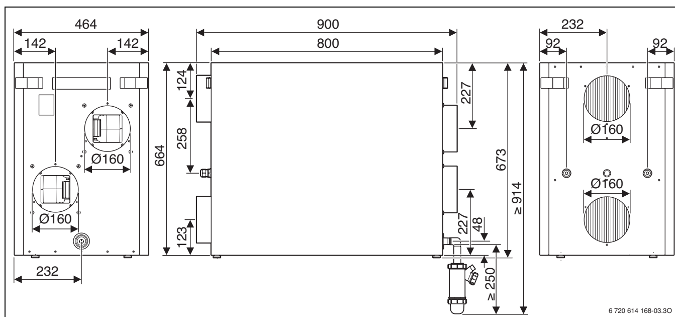
Bild 3 LP 250/LP 350 (Abmessungen in mm)
