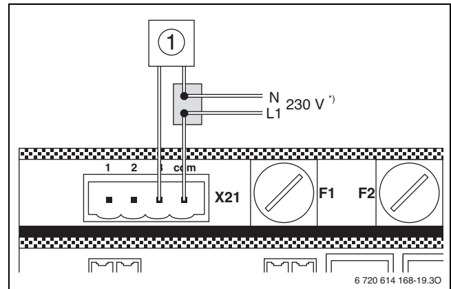
Bild 27 Klemmenbelegung Stellmotor
