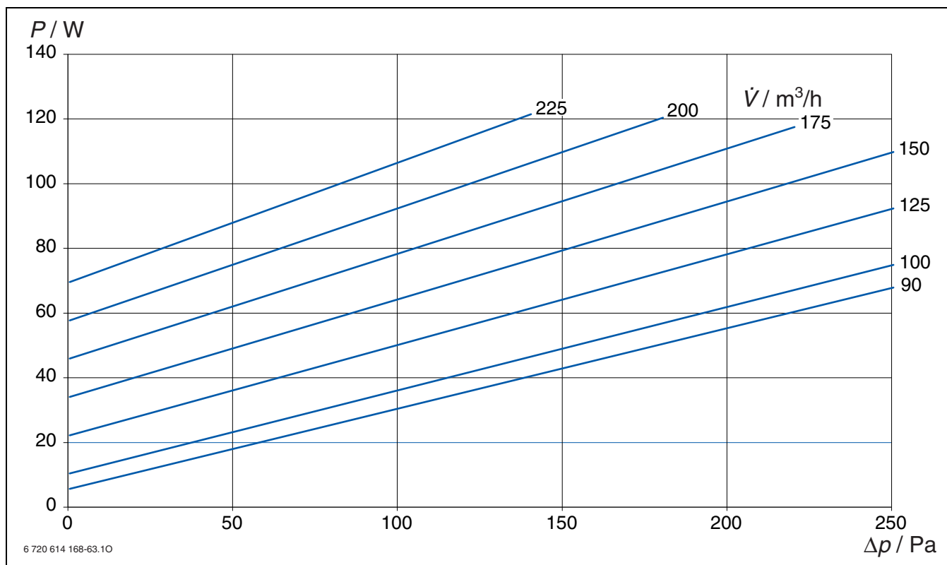
Bild 12 LP 150
