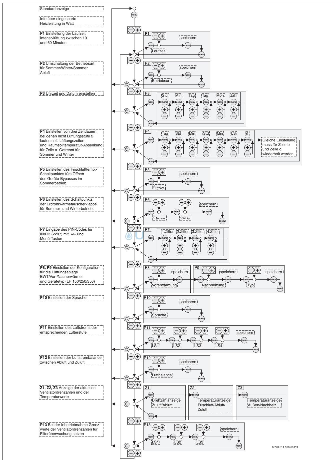
Bild 39 Menüstruktur
