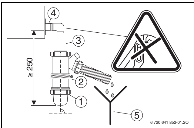
Bild 20 Kondensatableitung (LP 250/LP 350)
