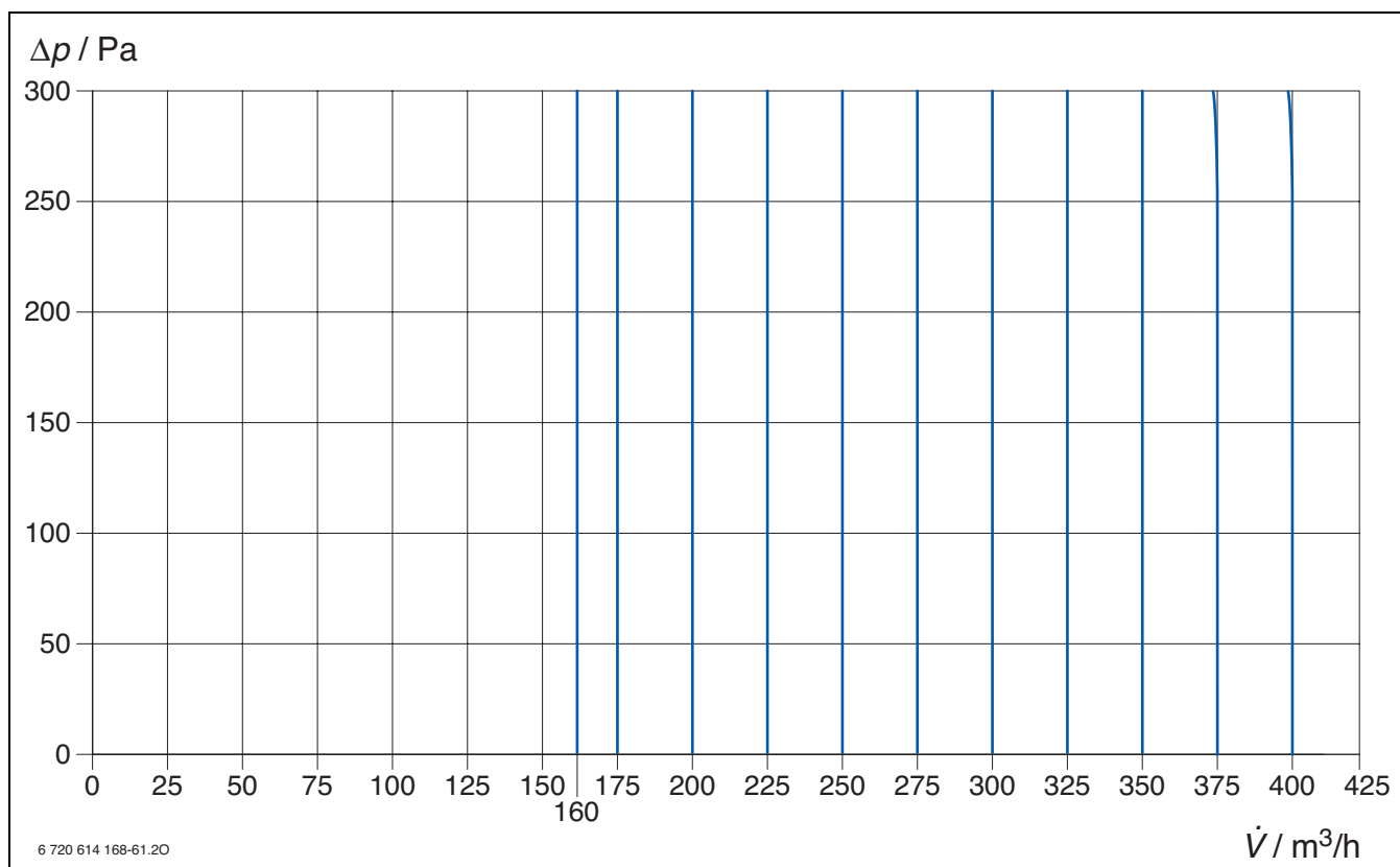
Bild 11 LP 350
