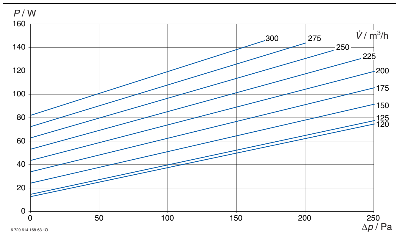
Bild 13 LP 250
