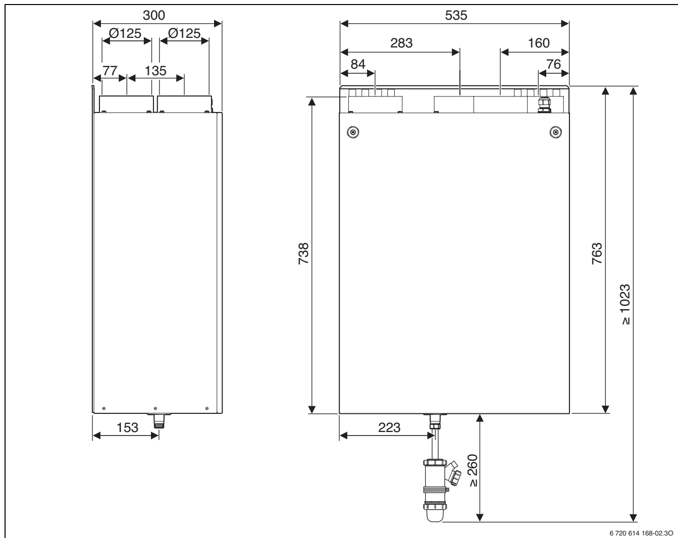
Bild 2 LP 150 (Abmessungen in mm)
