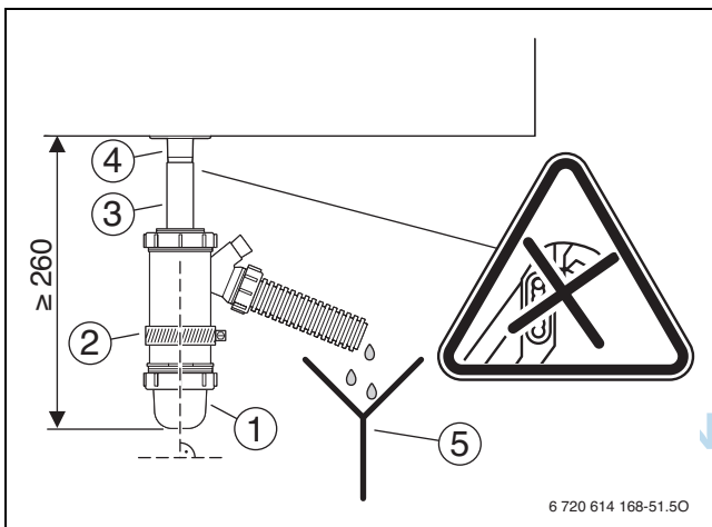
Bild 19 Kondensatableitung (LP 150)
