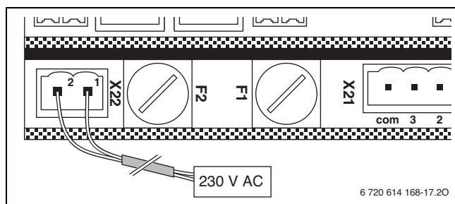
Bild 23 Klemmenbelegung Netzanschluss
