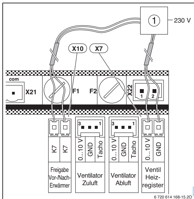
Bild 29 Klemmenbelegung Heizregister
