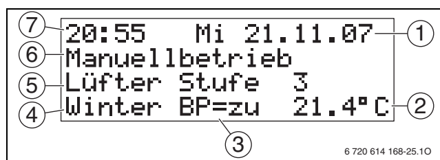
Bild 37 Standardanzeige
