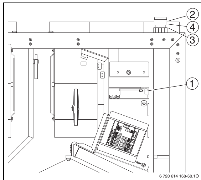
Bild 24 Erdungsanschluss und Kabeldurchführungen LP 150
