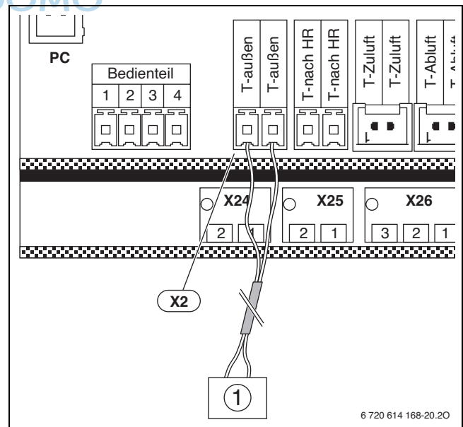
Bild 28 Klemmenbelegung Temperaturfühler für Außentemperatur
