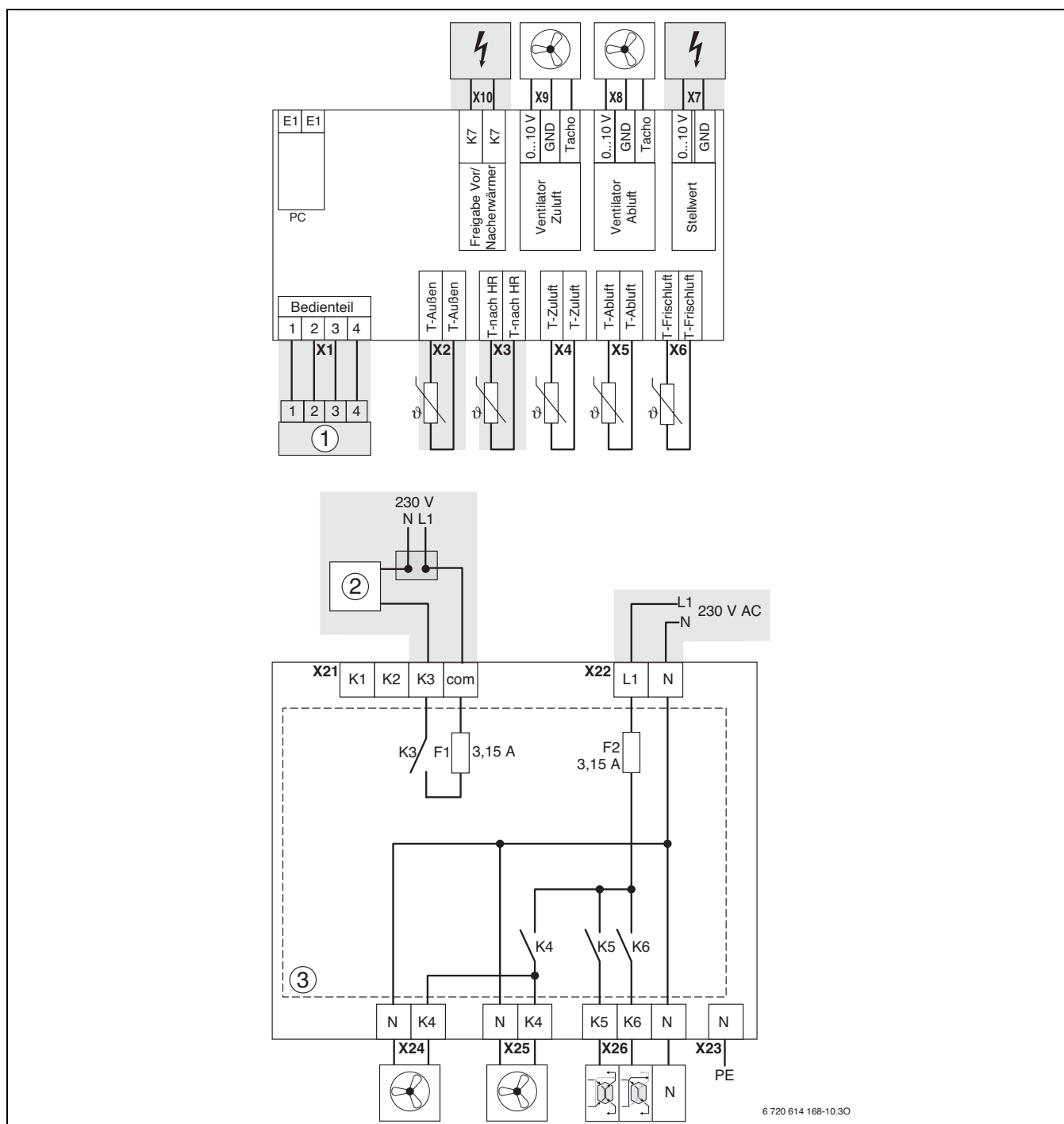
Bild 8 Anschlussplan (für Installation relevante Anschlüsse sind grau hinterlegt)
