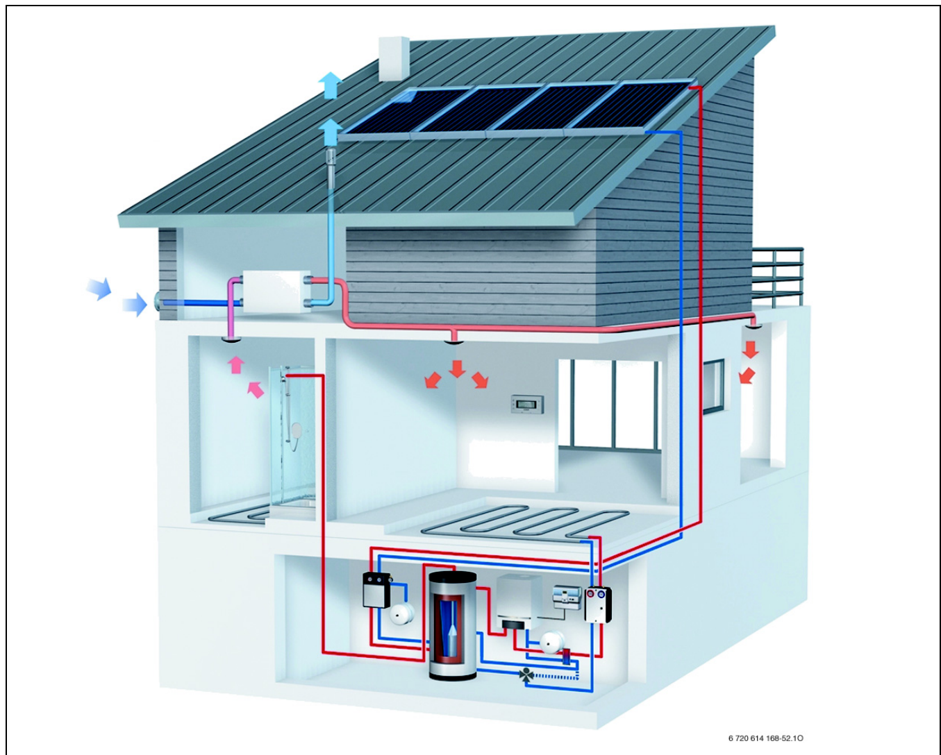
Bild 16 Anlagenbeispiel
