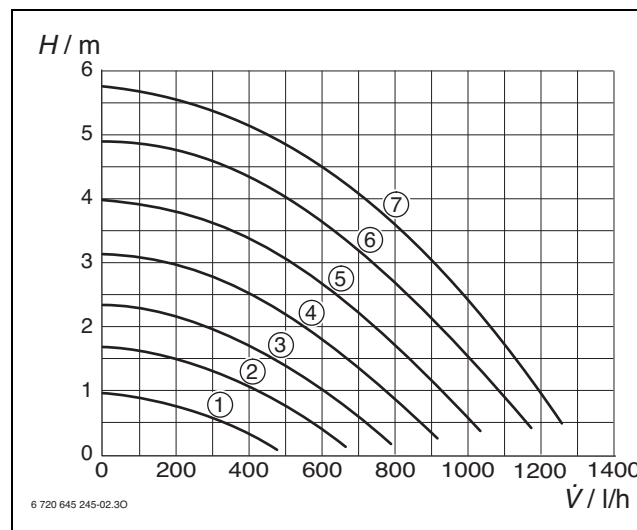
Bild 38 Pumpenkennlinien
