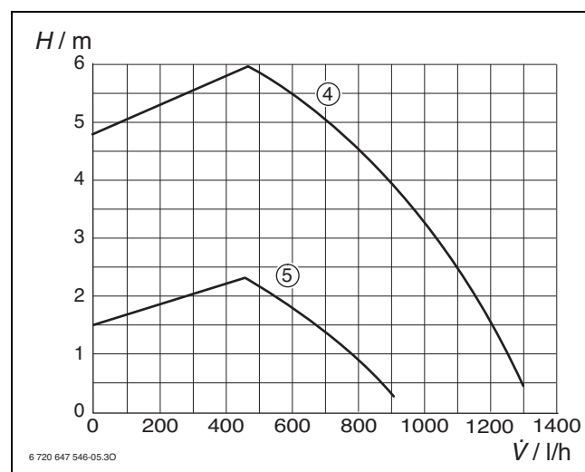
Bild 37 Proportionaldruck
