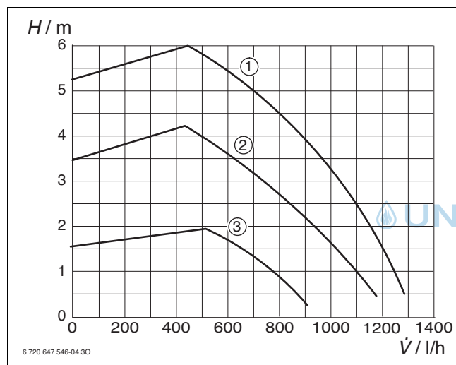
Bild 36 Konstantdruck
