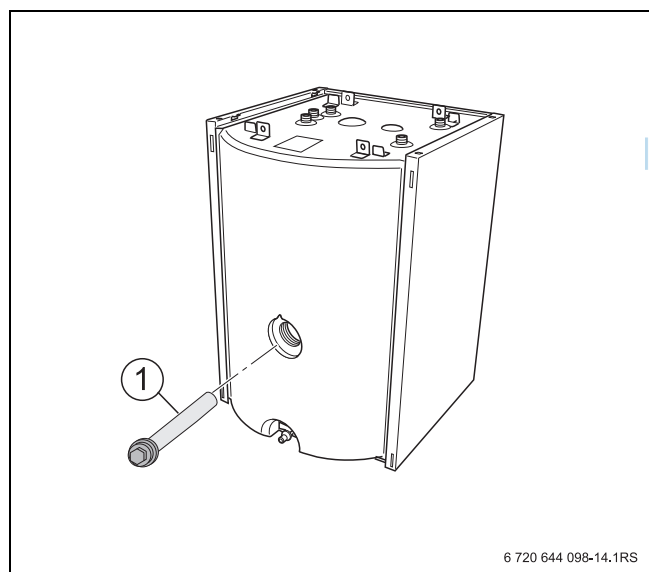
Bild 15 Magnesium-Anode prüfen
