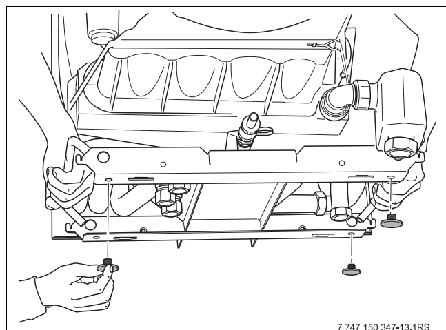
Bild 18 Fußschrauben ohne Transportmittel montieren
