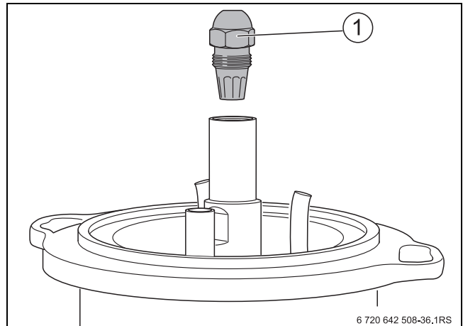
Bild 51 Düse abschrauben
