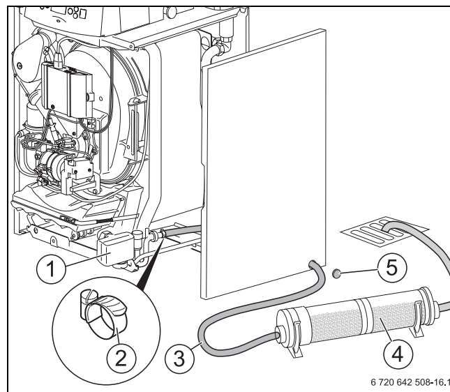
Bild 21 Kondensatablauf mit Neutralisation
