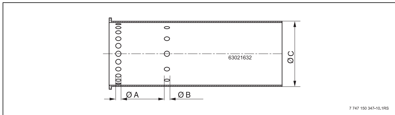
Bild 7 Brennerrohre
