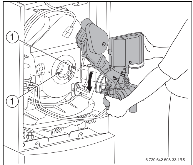
Bild 68 Brenner herausnehmen
