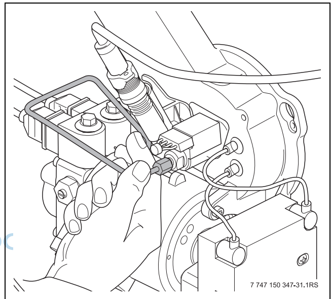
Bild 57 Ölleitung herausziehen
