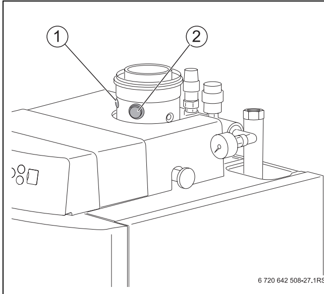
Bild 39 Messwerte aufnehmen
