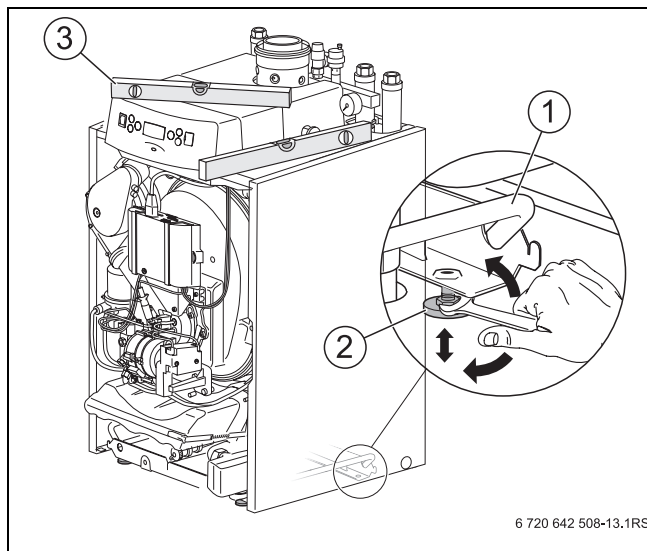
Bild 20 Heizkessel ausrichten
