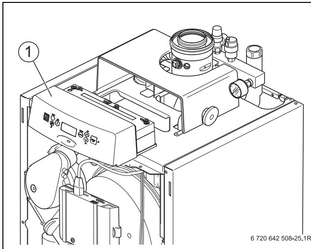
Bild 28 Bedieneinheit
