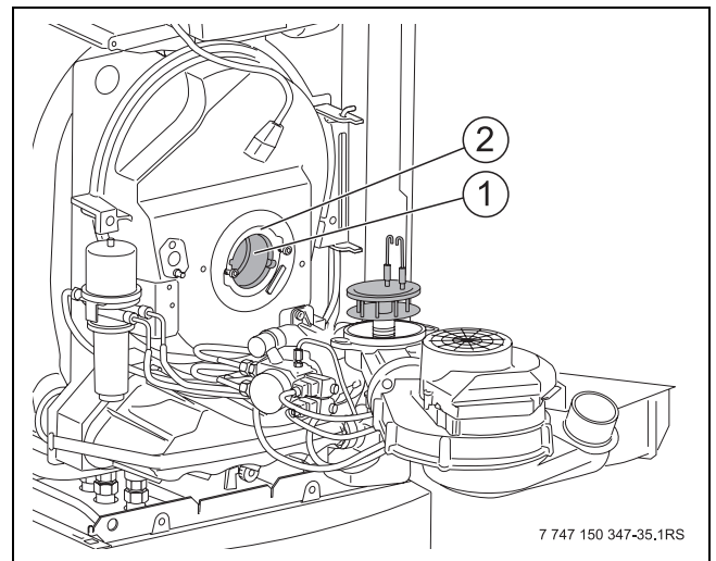
Bild 54 Brennerrohr austauschen
