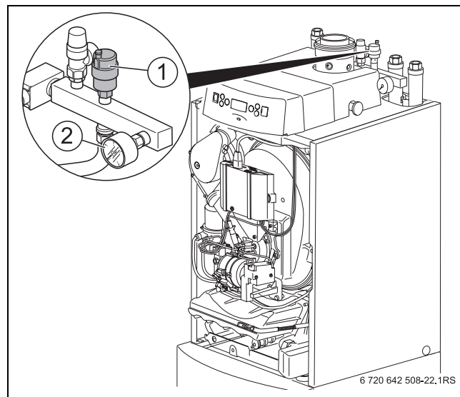
Bild 24 Heizungsanlage befüllen
