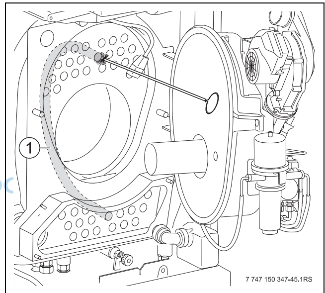
Bild 62 Heizgaszüge im Feuerraum reinigen
