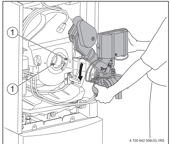
Bild 48 Brenner herausnehmen
