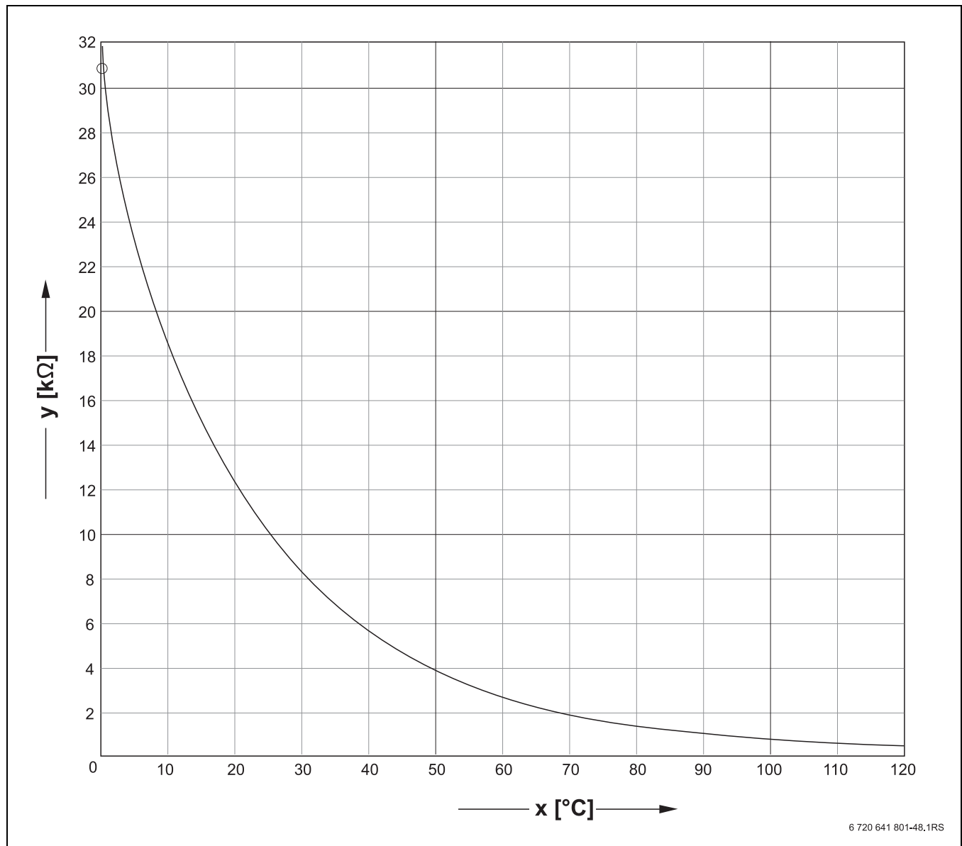
Bild 78 Fühlerkennlinien: Kesselwasser-, Rück- und Vorlauftemperaturfühler
