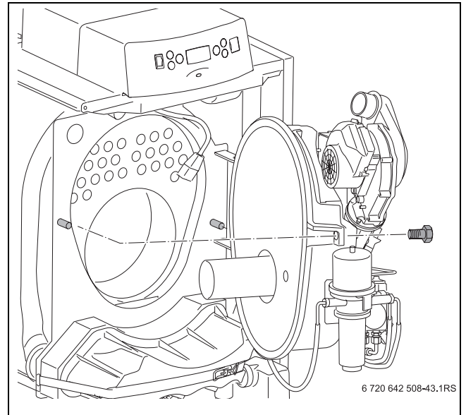
Bild 59 Brenntür öffnen
