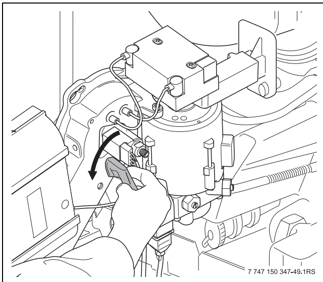
Bild 71 Winkelhalter demontieren
