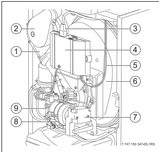
Bild 2 Ölbrenner
