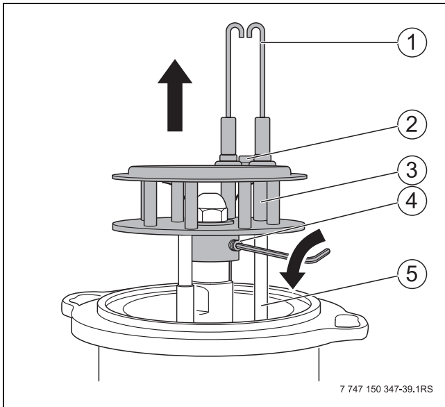
Bild 70 Mischsystem demontieren
