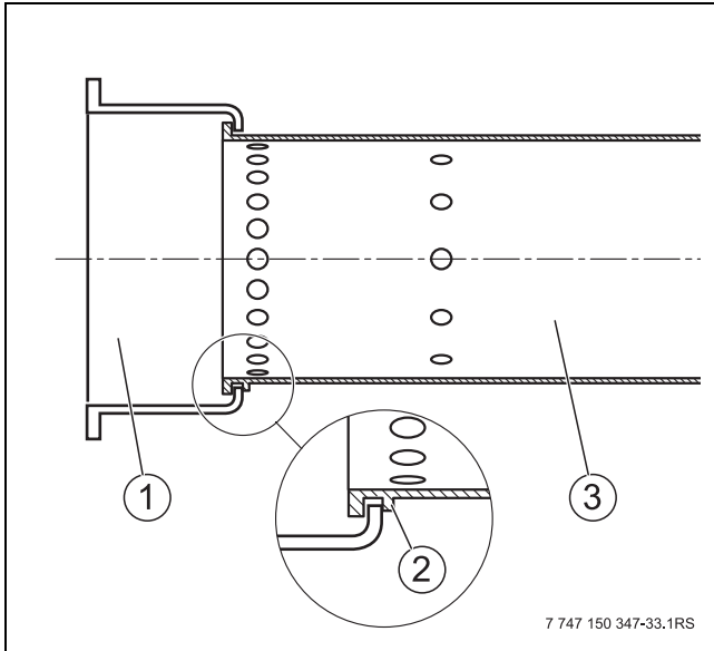
Bild 55 Brennerrohr einsetzen
