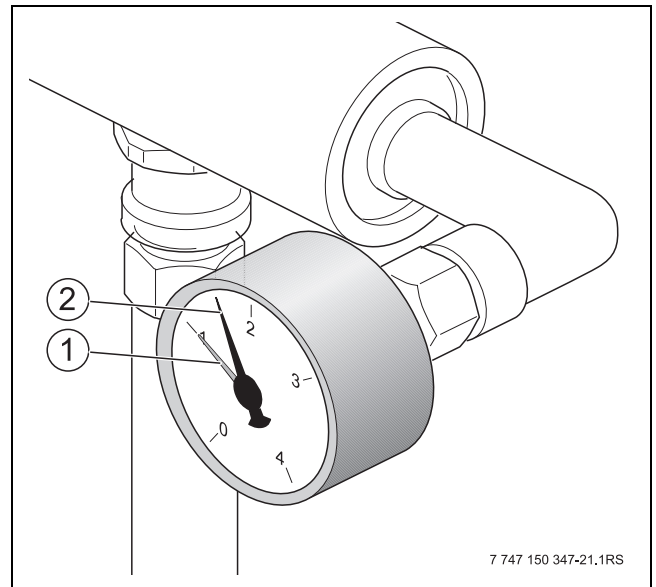
Bild 66 Manometer
