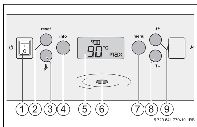
Bild 32 Bedienelemente
