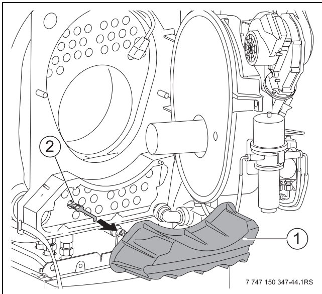
Bild 61 Turbulatoren herausziehen
