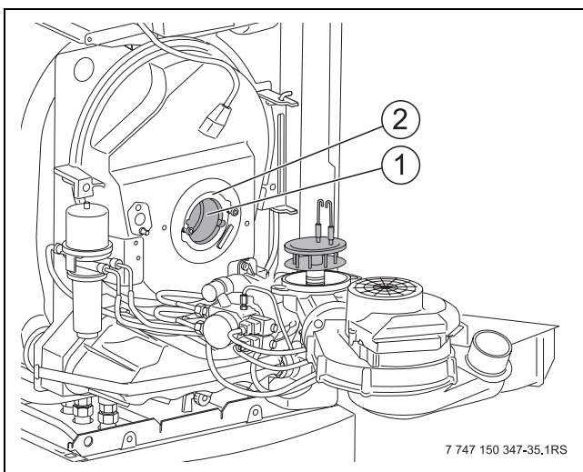
Bild 56 Dichtung prüfen
