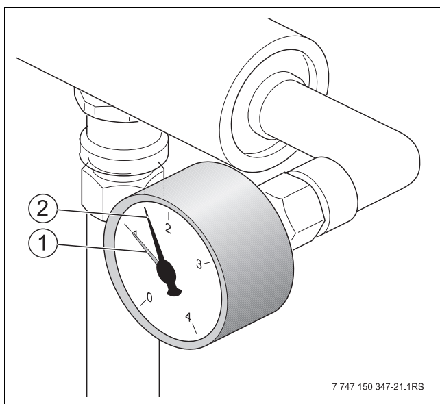
Bild 23 Manometer
