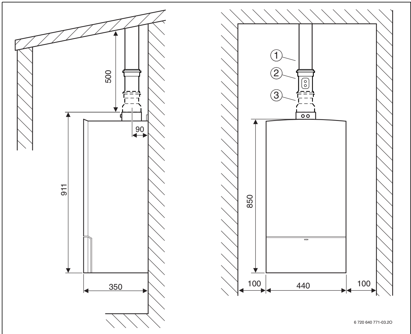
Bild 7 Schrägdach
