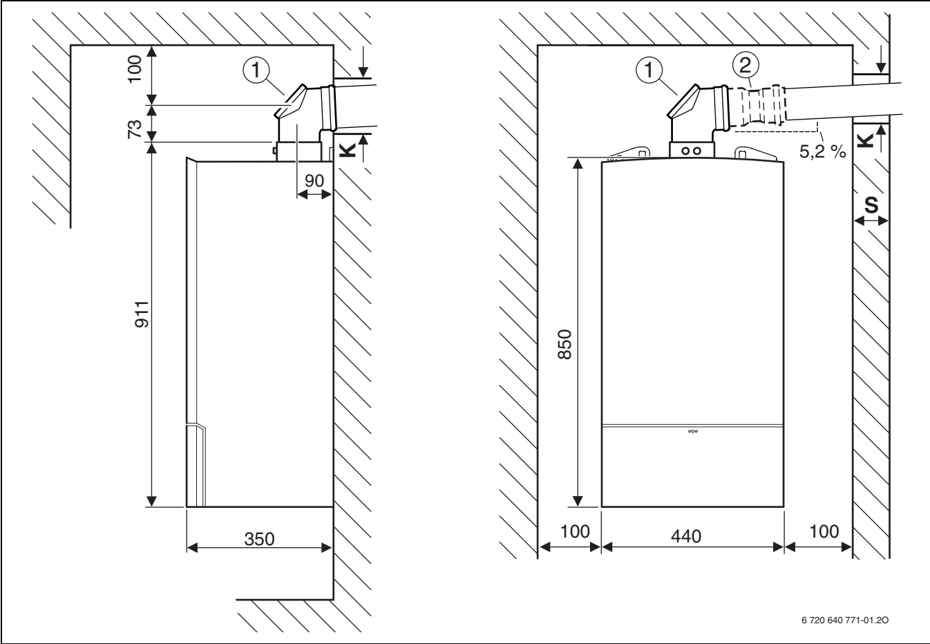
Bild 5 Abgasführung Ø 80/125 mm, Ø 80 mm oder Ø 60/100 mm [1] Bogen 90° mit Prüföffnung Ø 80/125 mm [2] Adapter Ø 80/125 mm auf Ø 60/100 mm (nur erforderlich bei Abgaszubehör Ø 60/100 mm)
