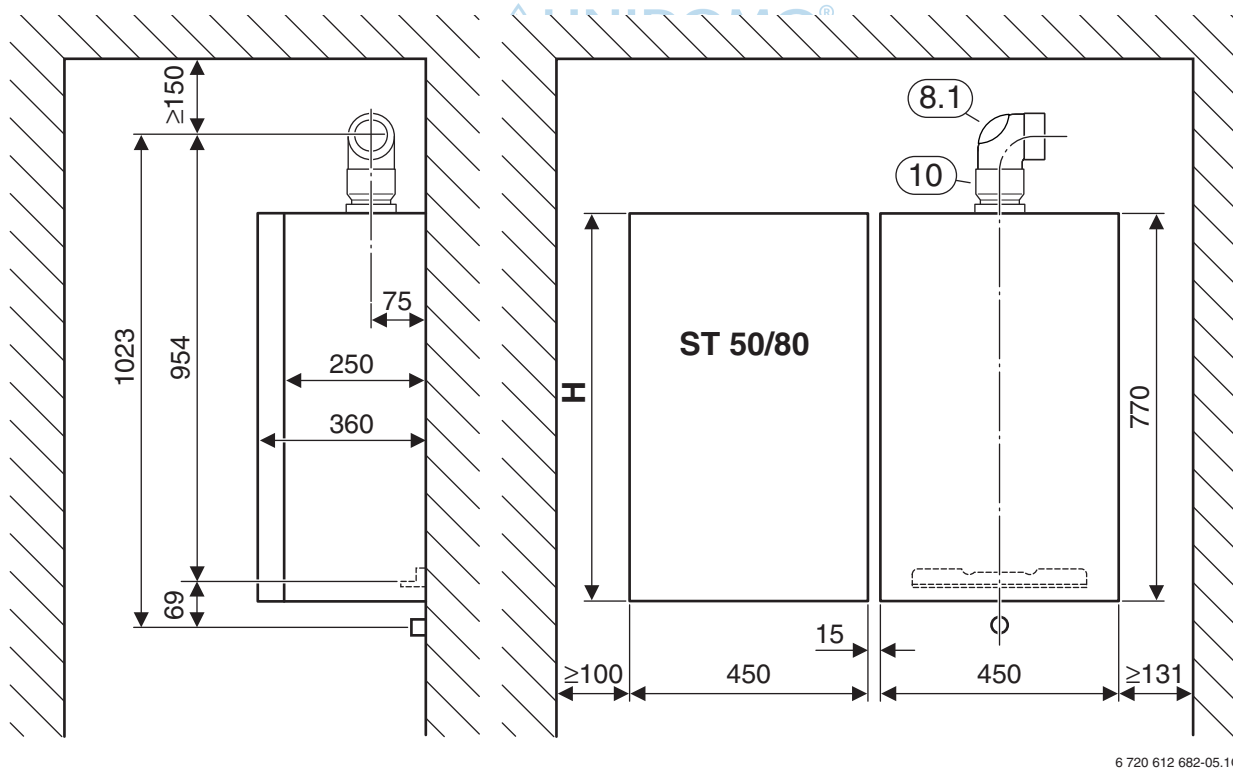
Bild 5 Gas-Kesseltherme neben Speicher ST 50/80
