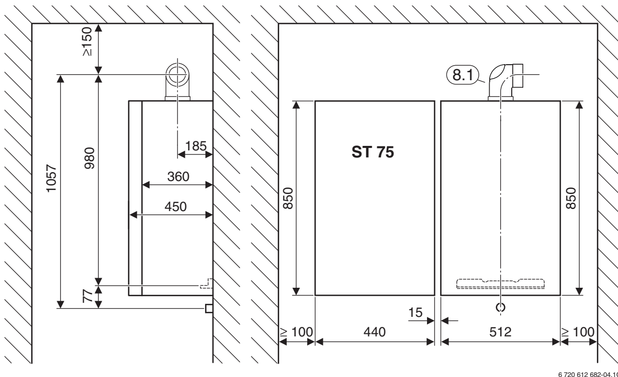
Bild 4 Gas-Kesseltherme neben Speicher ST 75
