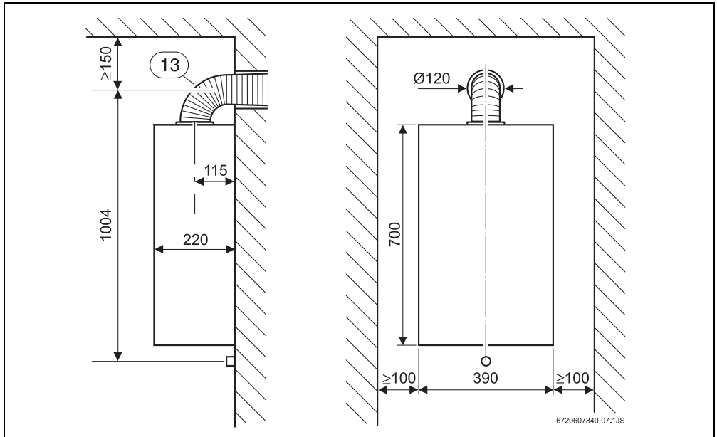
Bild 8 LAS Ø 80/110 mit Wellrohr
