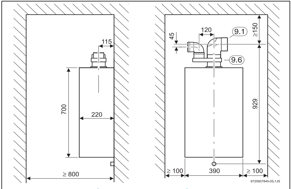
Bild 6 Abgasführung nach rechts, Verbrennungsluftführung von links
