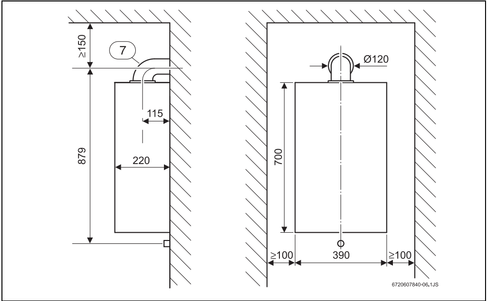
Bild 7 LAS Ø 80/110 mit 90°-Rohrbogen
