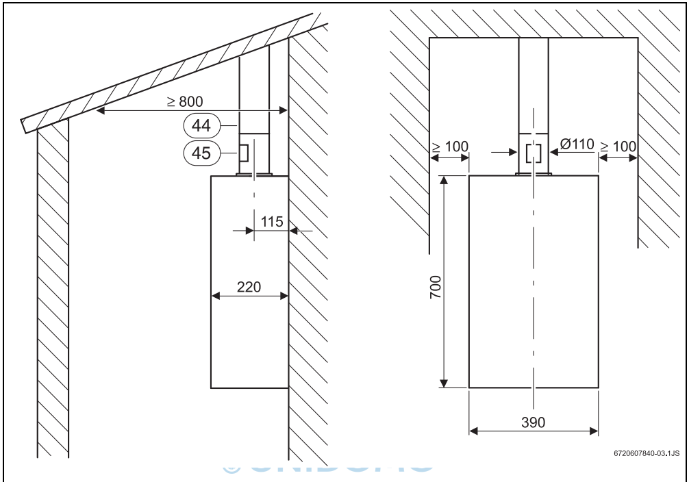
Bild 4 Schrägdach
