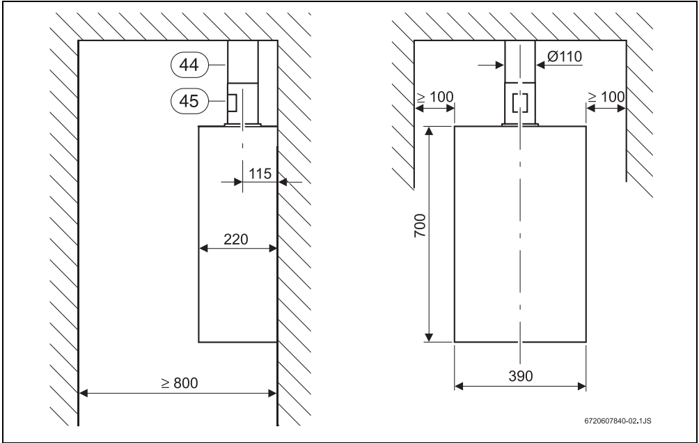
Bild 3 Flachdach
