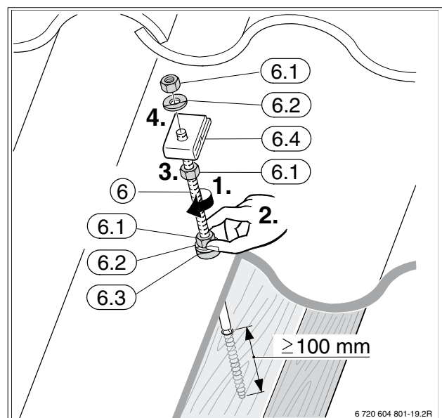
Bild 23 Stockschrabe montieren (Mindesteinschraubtiefe 100 mm)
