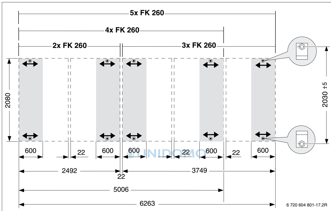
Bild 21 Kollektorfeldmaße und Toleranzbereiche für die Befestigung der Stockschraben
