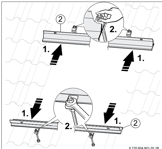
Bild 24 Trageprofile montieren
