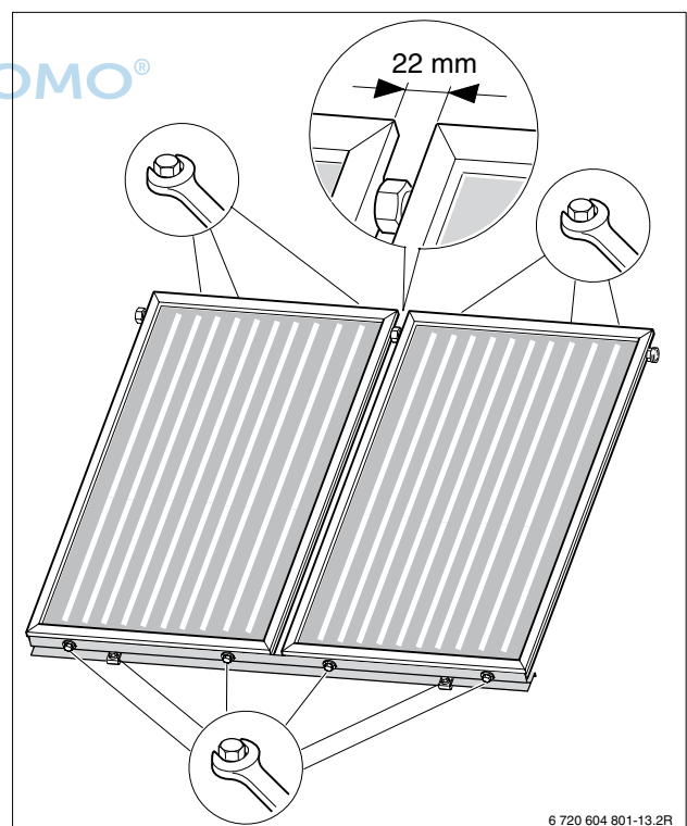
Bild 28 Flachkollektoren ausrichten und befestigen
