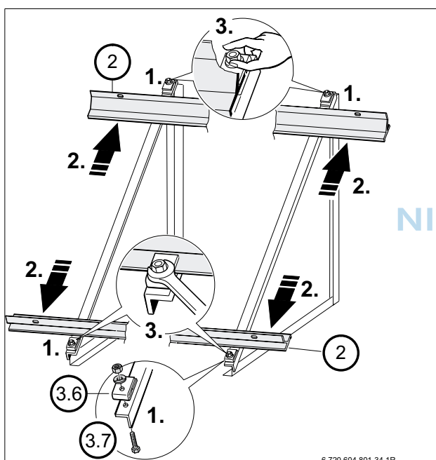
Bild 45 Trageprofile montieren
