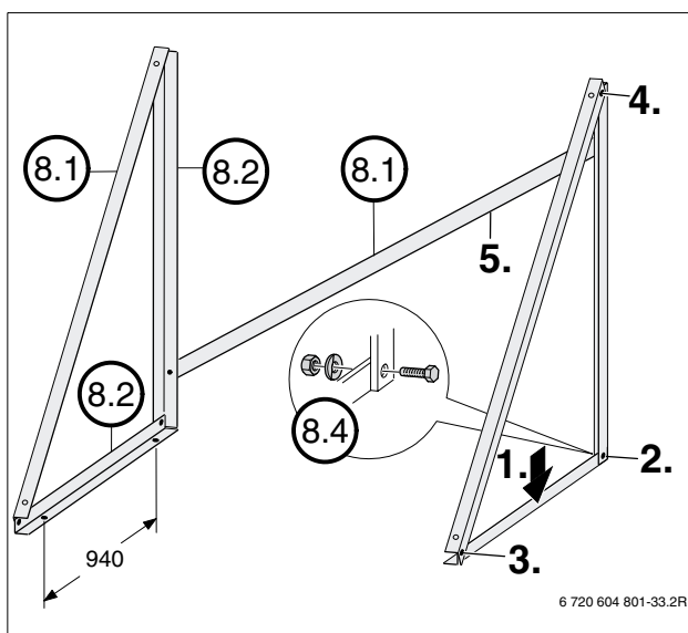
Bild 44 Flachdachgestell montieren
