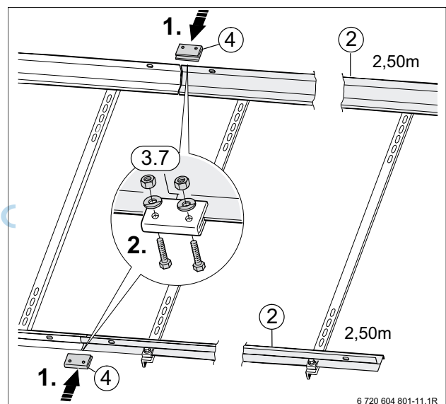
Bild 15 Erweiterung um zwei Flachkollektoren
