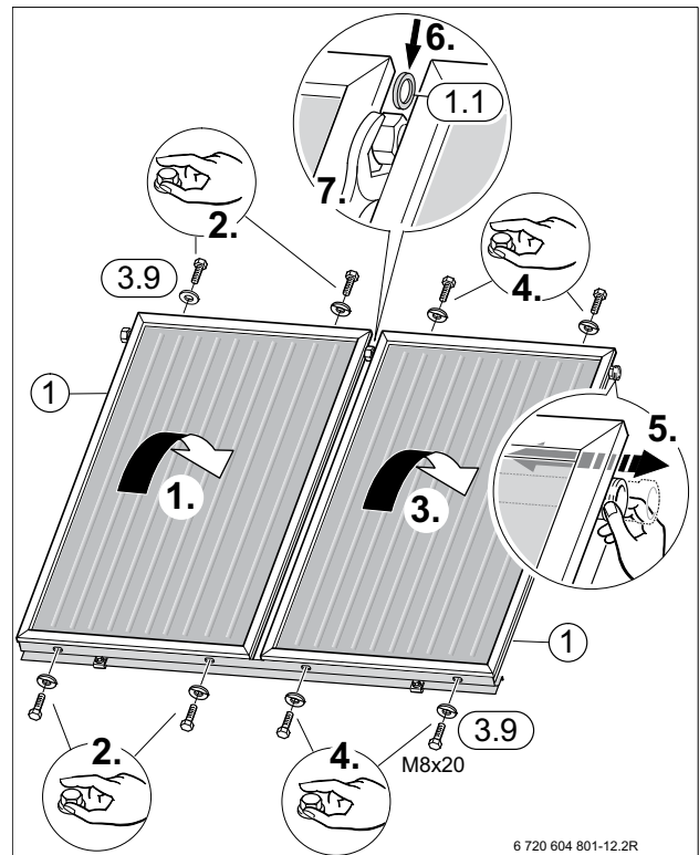
Bild 27 Flachkollektoren einlegen, mit Schrauben sichern und zusammenschließen
