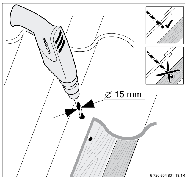
Bild 22 Dachpfanne durchbohren
