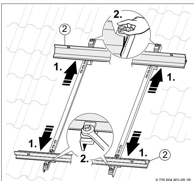
Bild 13 Trageprofile montieren
