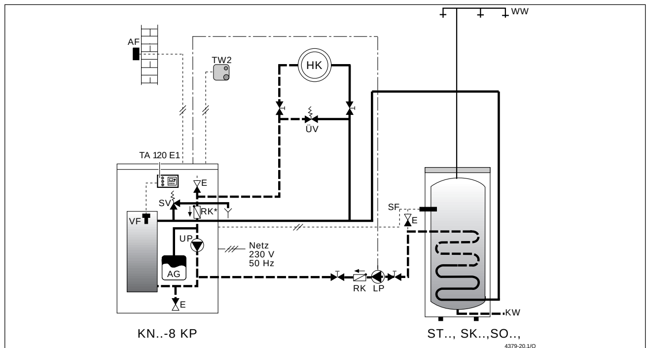
Bild 1: * Rückschlagklappe RK 1 (24)
