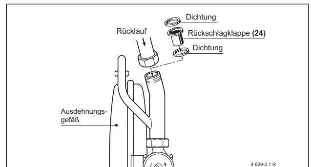
Bild 2: Einbau Rückschlagklappe RK 1 (24)
