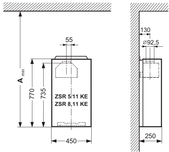
Bild 3 Heizgerät (in Raum 1)
