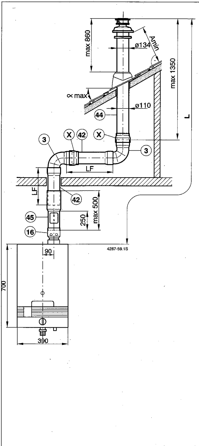
Bild 74: Montagebeispiel
