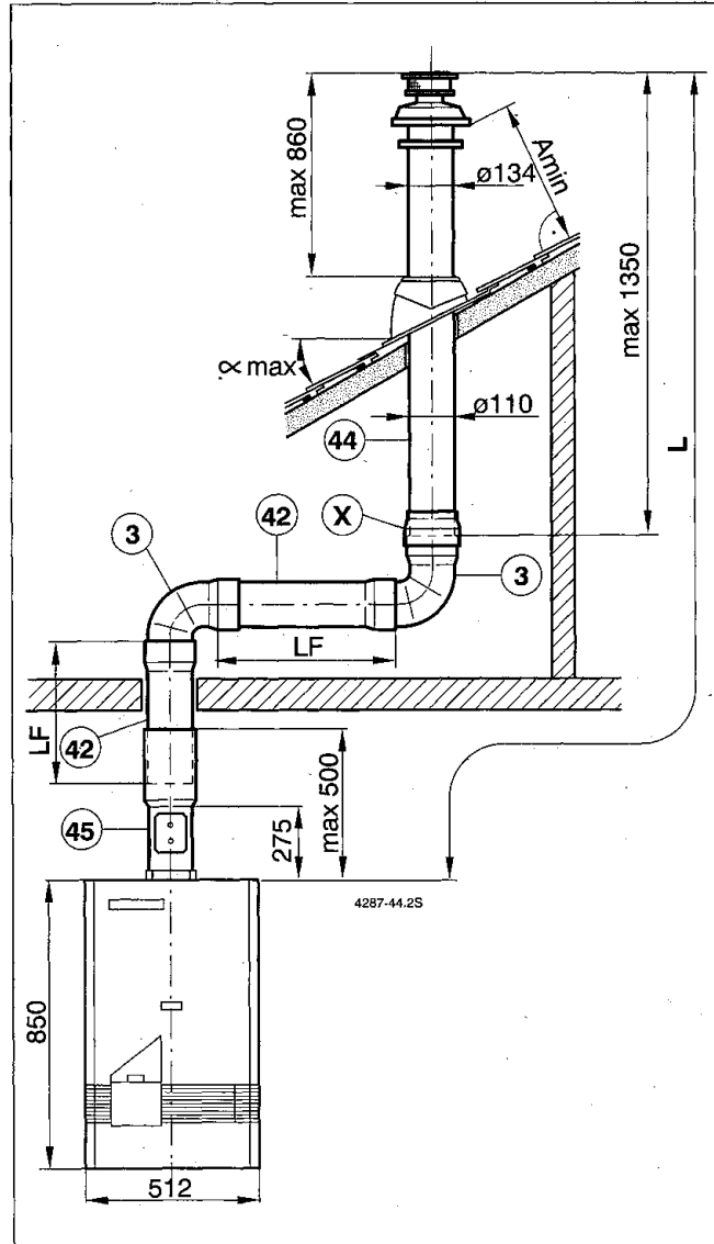
Bild 59: Montagebeispiel
