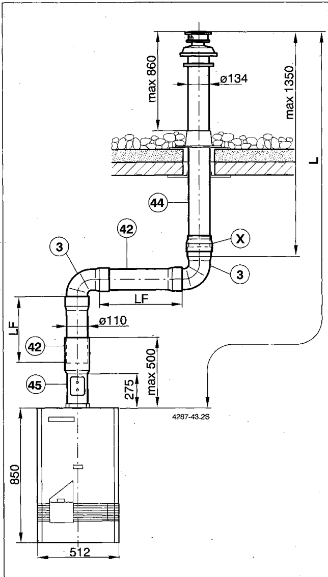
Bild 58: Montagebeispiel
