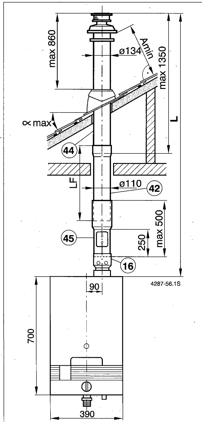
Bild 71: Montagebeispiel
