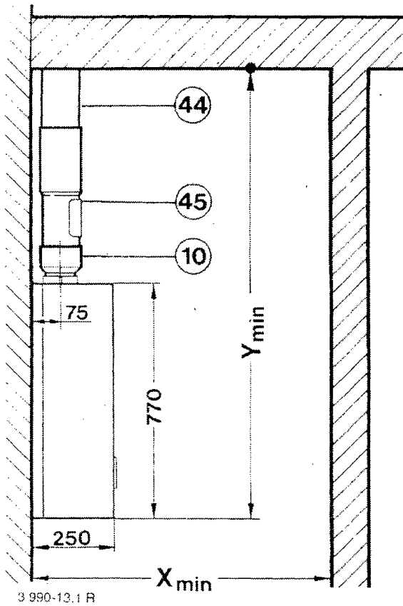
Bild 13: Flachdach
