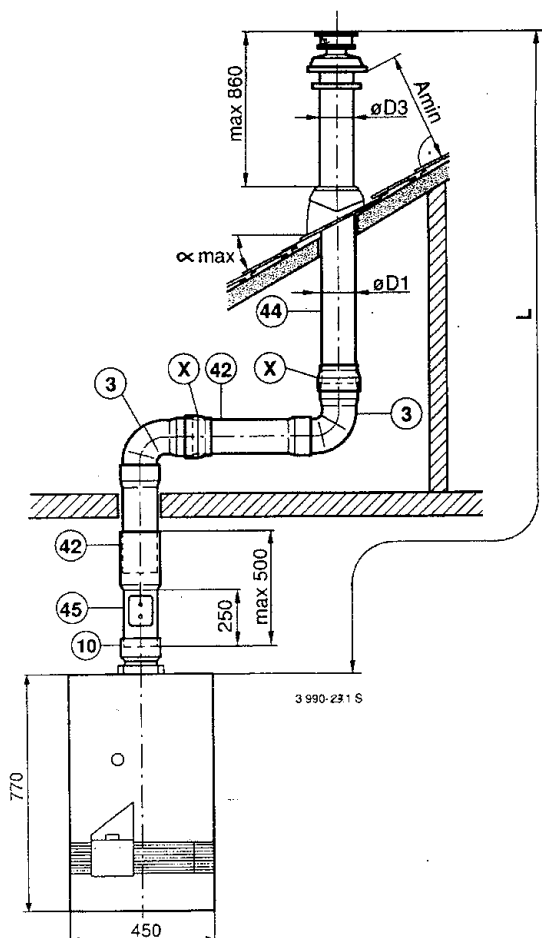
Bild 23 Montagebeispiel
