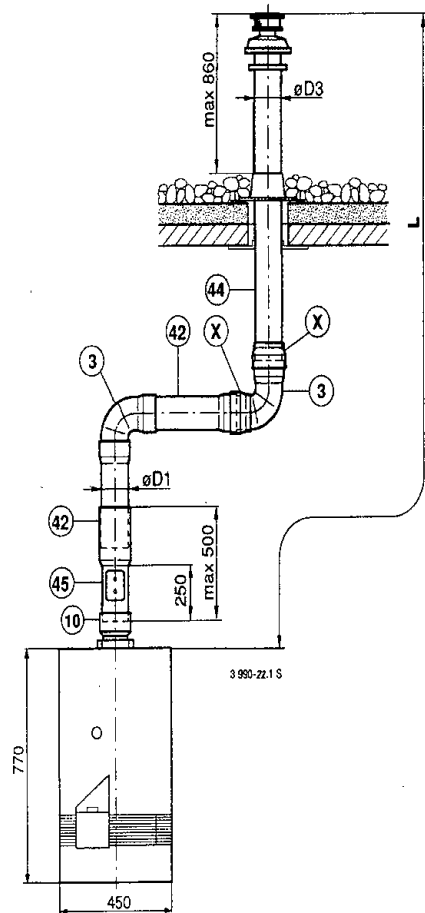
Bild 22 Montagebeispiel
