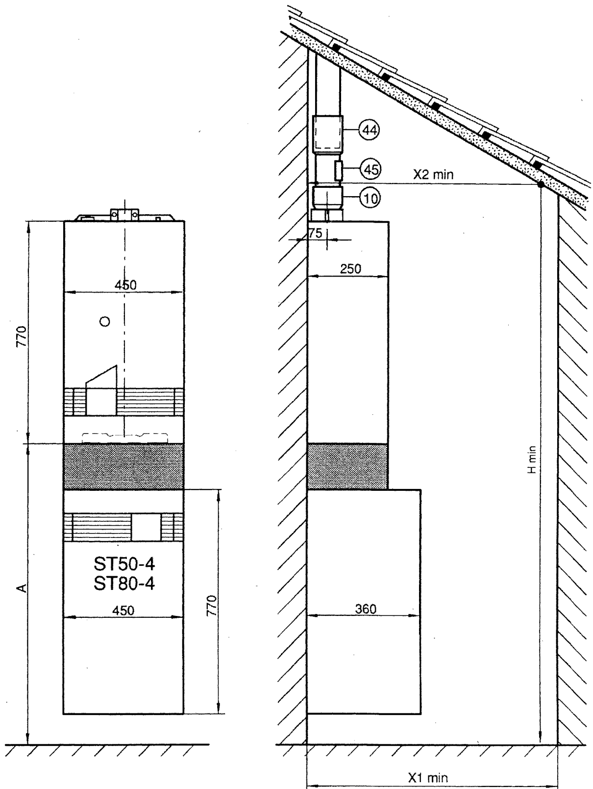
Bild 18 Schrägdach
