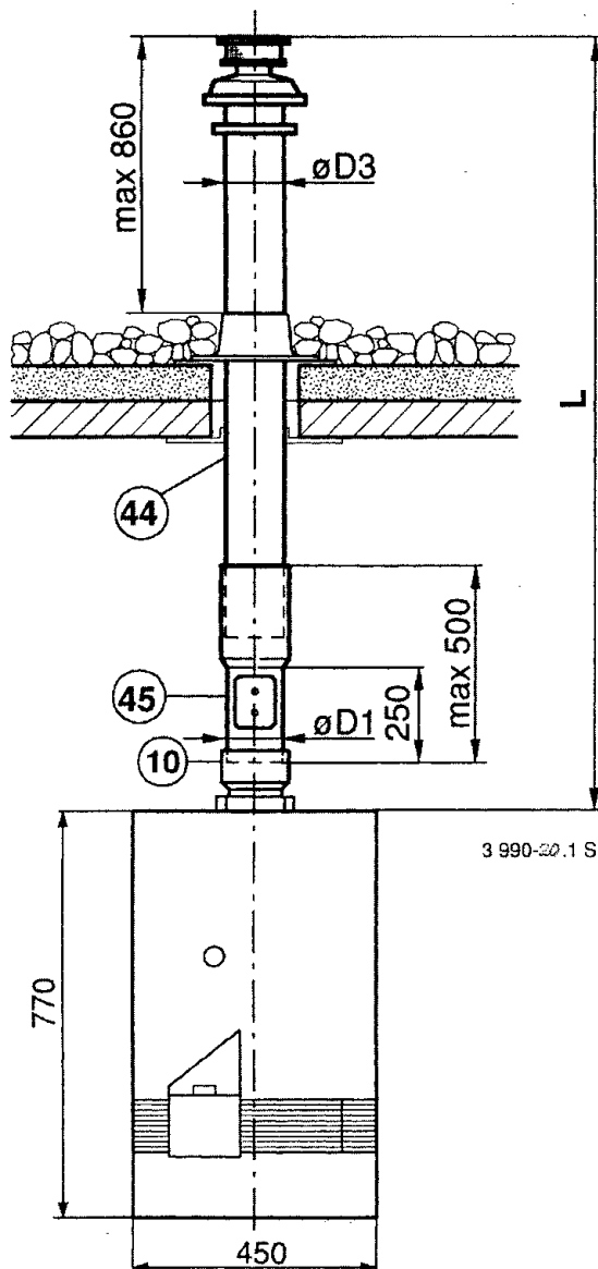
Bild 20 Montagebeispiel
