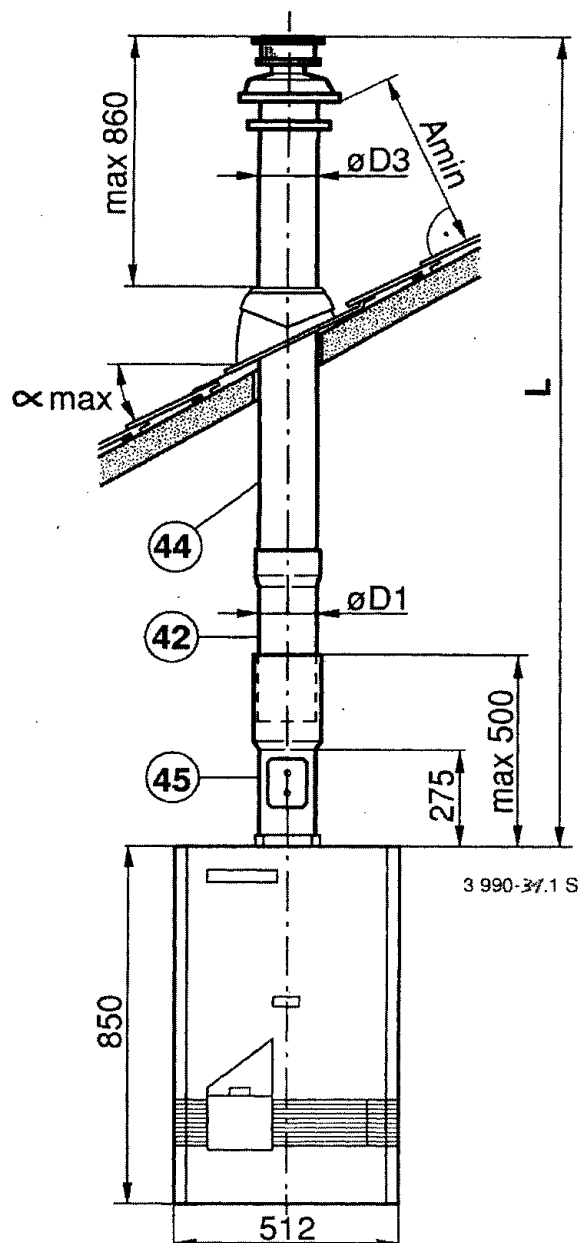
Bild 31 Montagebeispiel
