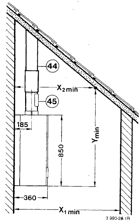
Bild 26: Schrägdach
