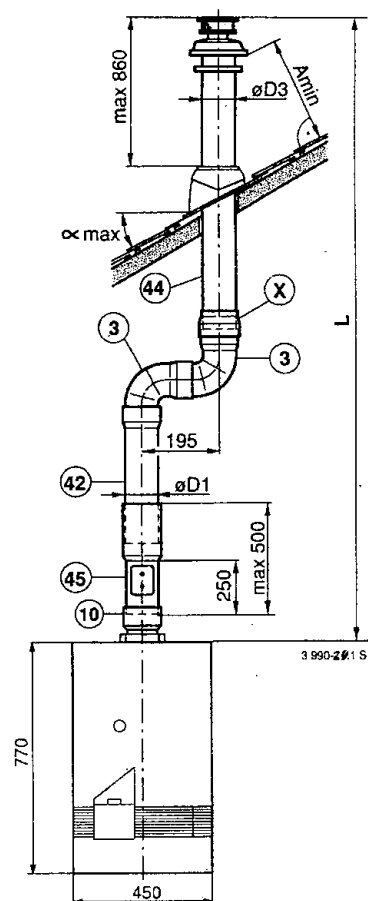
Bild 24 Montagebeispiel
