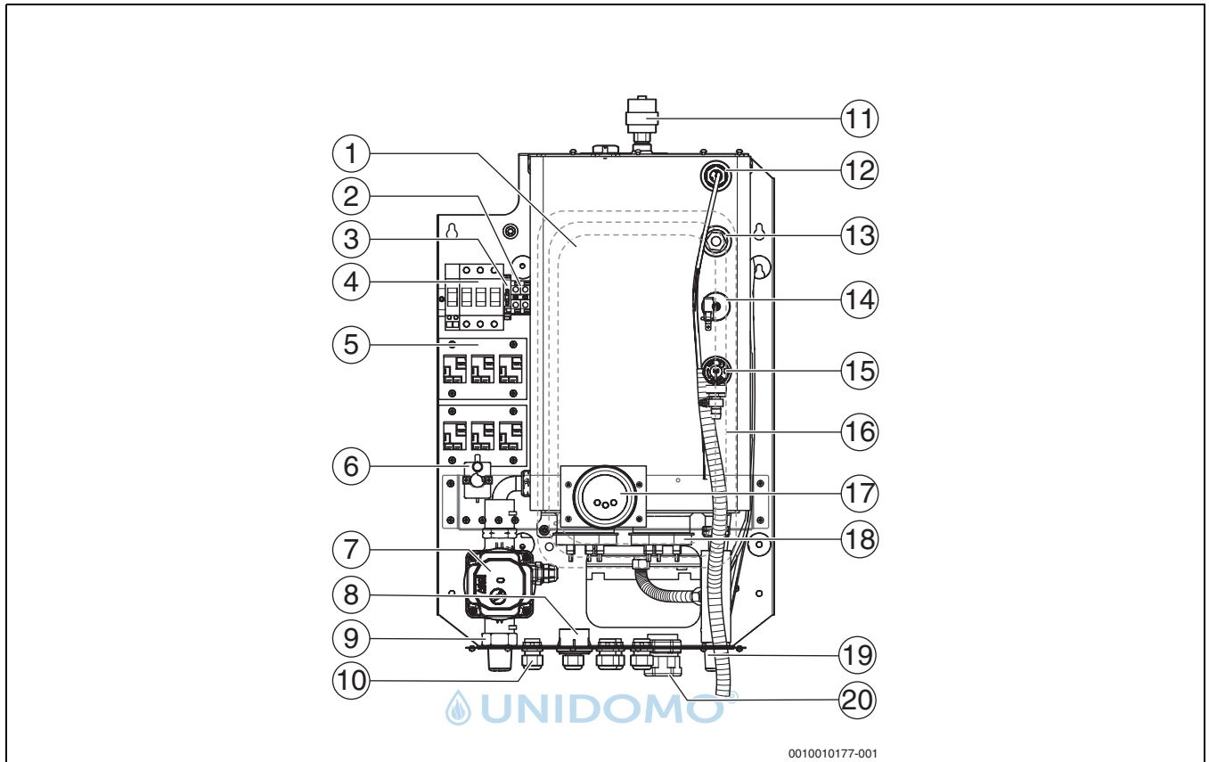
Bild 2 Funktionselemente des Heizgeräts Tronic Heat 3000/Tronic Heat 3500 15-24 kW
