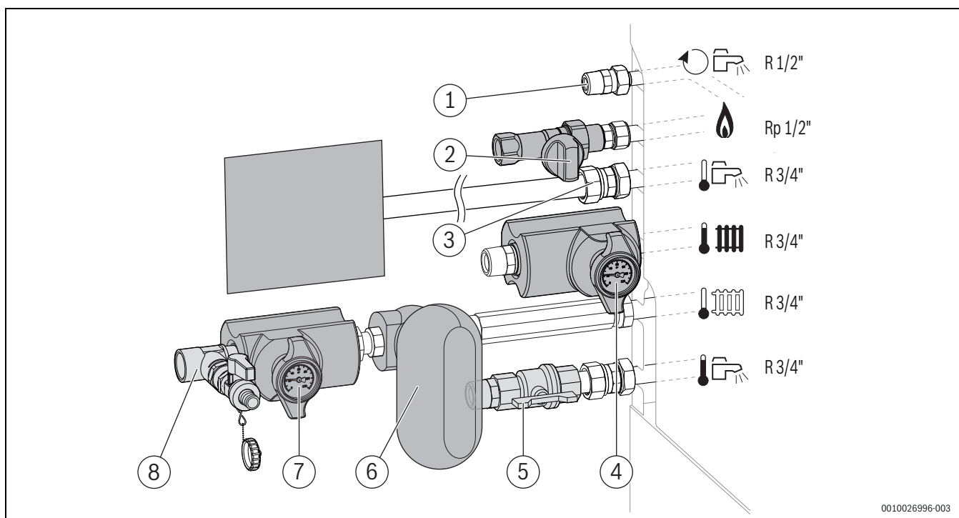
Bild 6 Beispiel: Gas- und wasserseitiger Anschluss mit dem Anschluss-Set Hähne (Zubehör CS 28-1) auf der linken Seite
