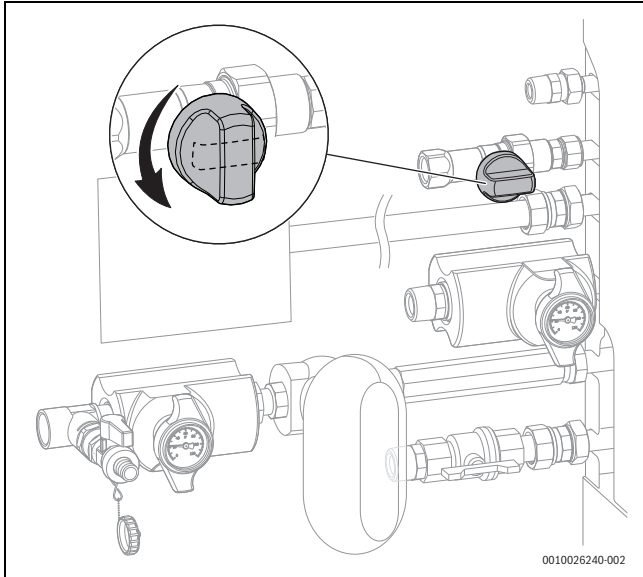
Bild 5 Gashahn öffnen
