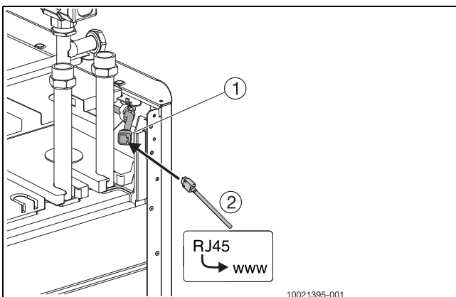
Bild 10 RJ45-Anschluss oben an der Rückseite des Geräts
