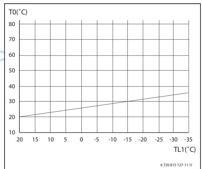
Bild 3 Fußbodenheizung
