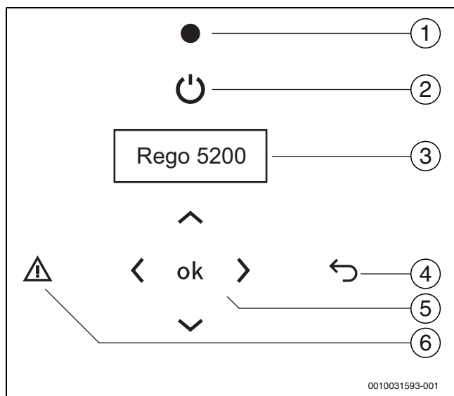
Bild 1 Bedienfeld
