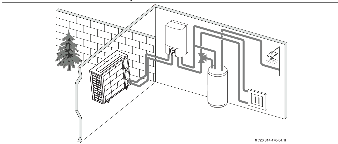
Bild 2 Wärmepumpe Außeneinheit, Inneneinheit ASE mit elektrischem Zuheizer, externer Warmwasserspeicher
