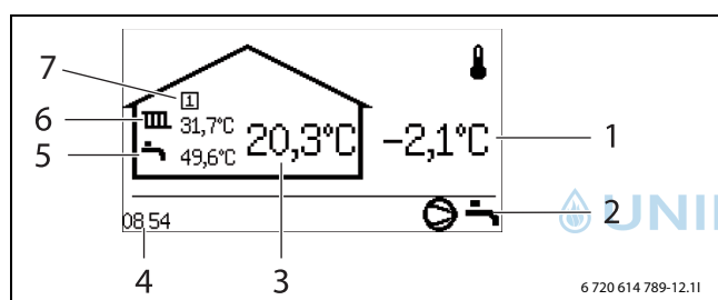
Bild 4 Standardanzeige
