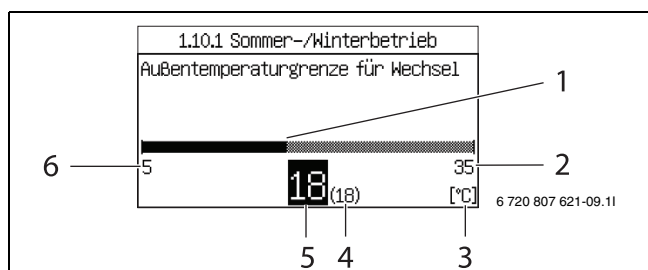
Bild 14 Hilfsinformation 2
