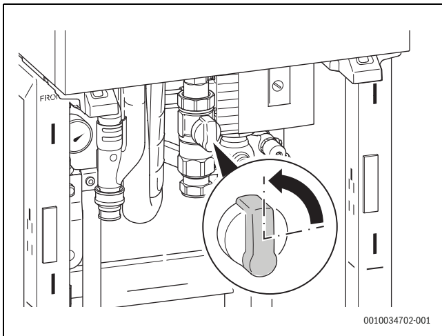
Bild 2 Öffnen des Gashahns
