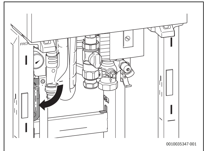
Bild 3 Öffnen der Serviceabsperrentile
