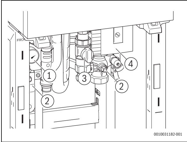
Bild 1 Übersicht Bauteile
