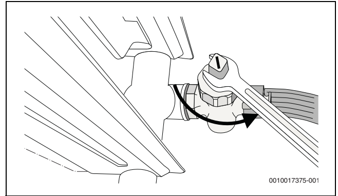
Bild 6 Entleeren der Heizungsanlage
