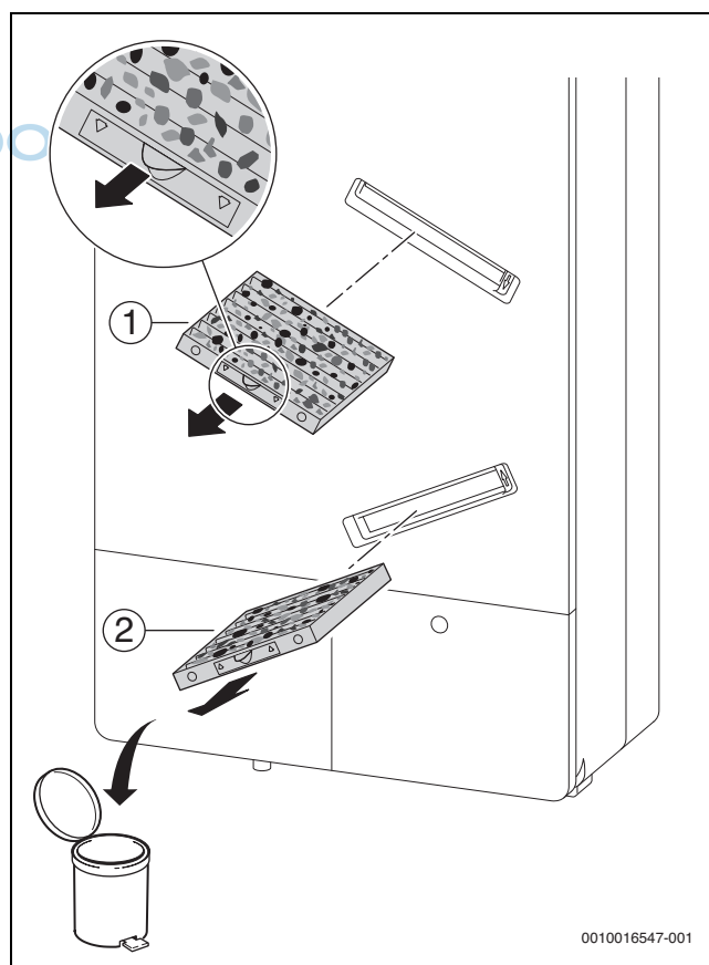
Bild 5 Filter herausziehen
