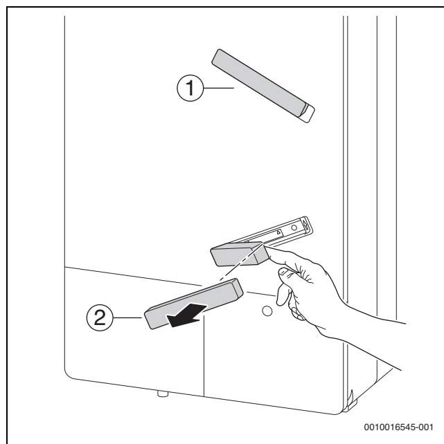
Bild 4 Filterabdeckung abnehmen
