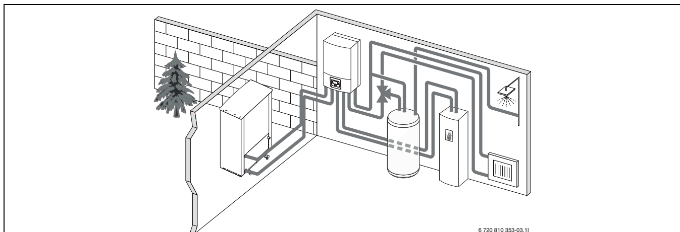
Bild 3 Wärmepumpe SAO-2/SAO-2 HT, Wärmepumpen-Kompakteinheit ACB ohne elektrischen Zuheizter, externer Warmwasserspeicher und externer Zuheizter
