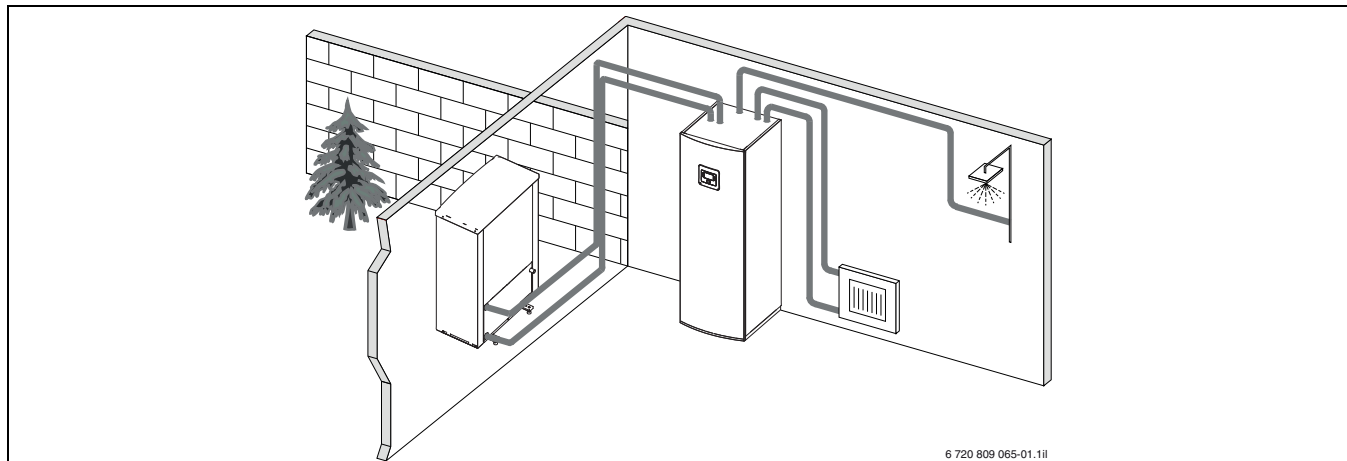
Bild 1 Wärmepumpe SAO-2/SAO-2 HT, Wärmepumpen-Kompakteinheit ACM mit integriertem Warmwasserspeicher und elektrischem Zuheizter
