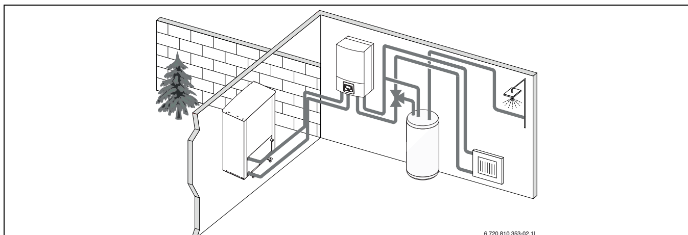
Bild 2 Wärmepumpe SAO-2/SAO-2 HT, Wärmepumpen-Kompakteinheit ACE mit elektrischem Zuheizter, externer Warmwasserspeicher
