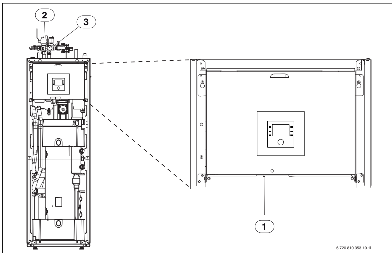
Bild 8 ACM/ACM solar
