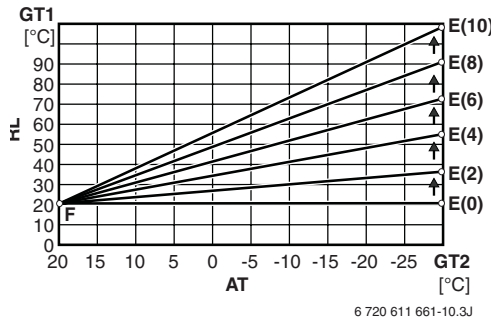
Bild 16 Anheben des Endpunkts der Heizkurve
