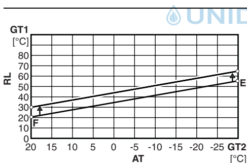
Bild 17 Parallelverschiebung der Heizkurve
