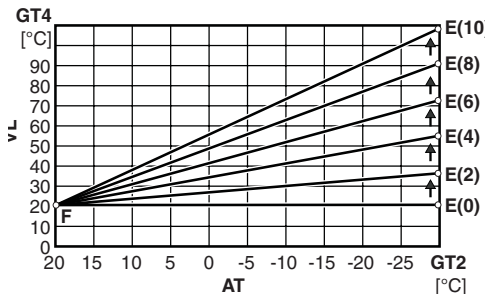
Bild 21 Anheben des Endpunkts der Heizkurve des Mischerkreises
