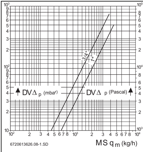
Bild 6 Druckverlust-Diagramm 3-Wege-Ventil
