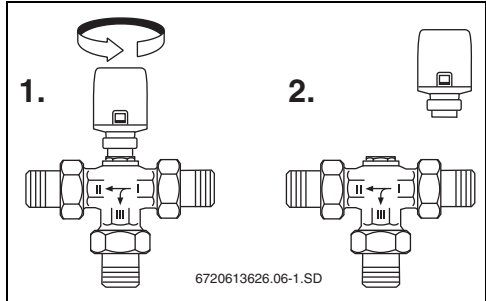
Bild 10 Stellantrieb demontieren
