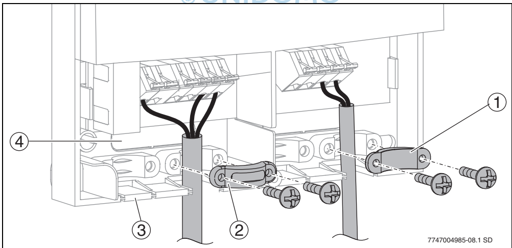
Bild 11 Durchföhrung und Befestigung der Kabel
