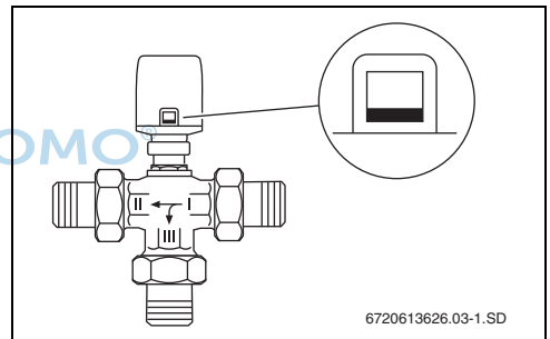
Bild 8 Hubanzeige im stromlosen Zustand
