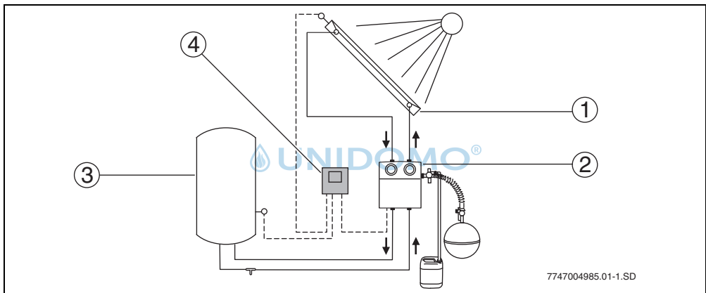
Bild 2 Anlagenschema
