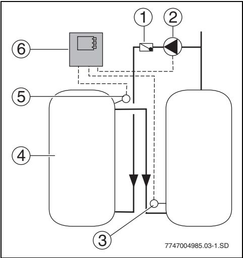
Bild 4 Umschichtfunktion
