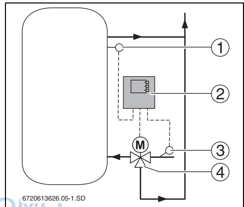
Bild 3 Rücklaufanhebung
